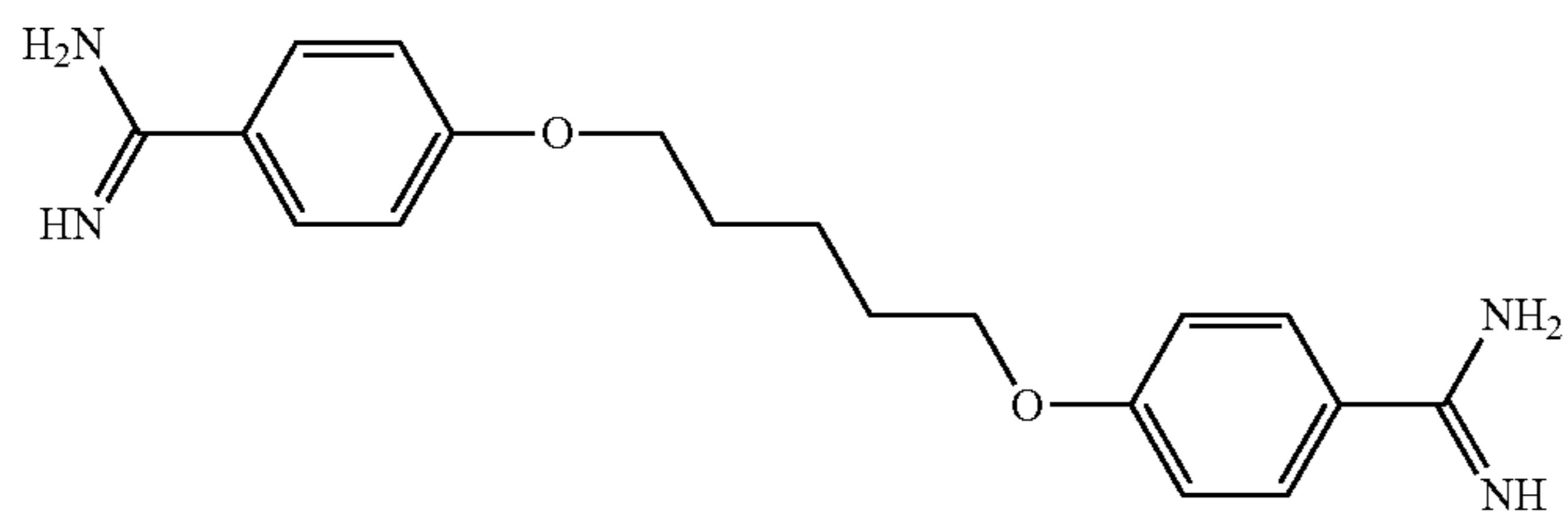
4,4'-pentanediyldioxy-bis-benzamidine
