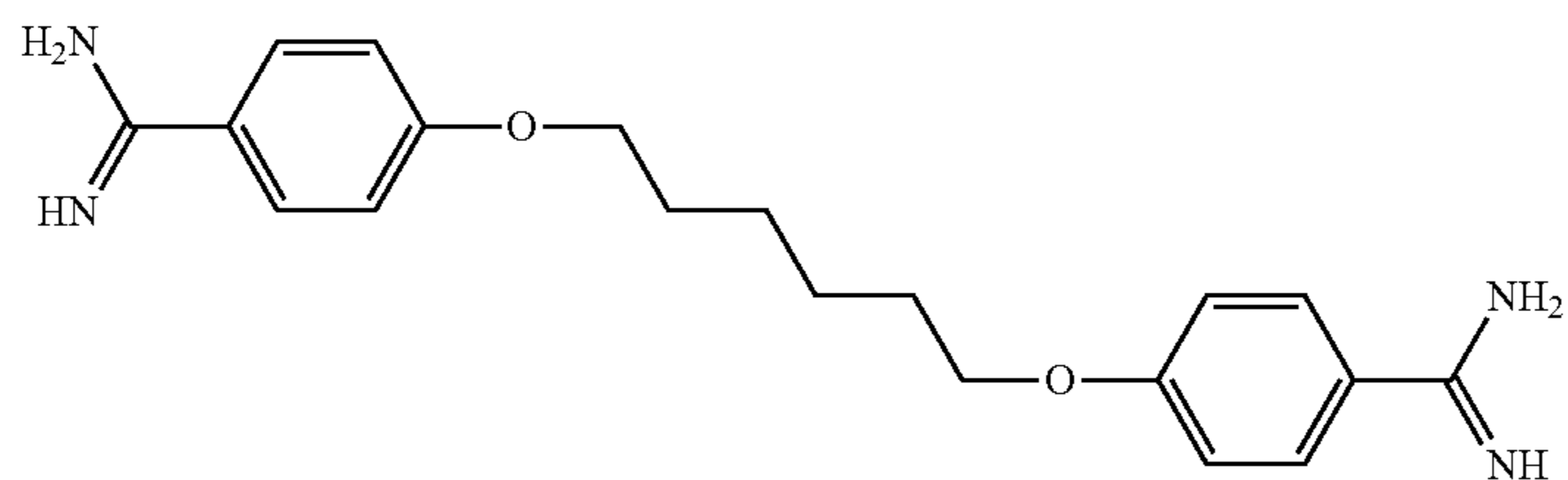
4,4'-hexanediyldioxy-bis-benzamidine
