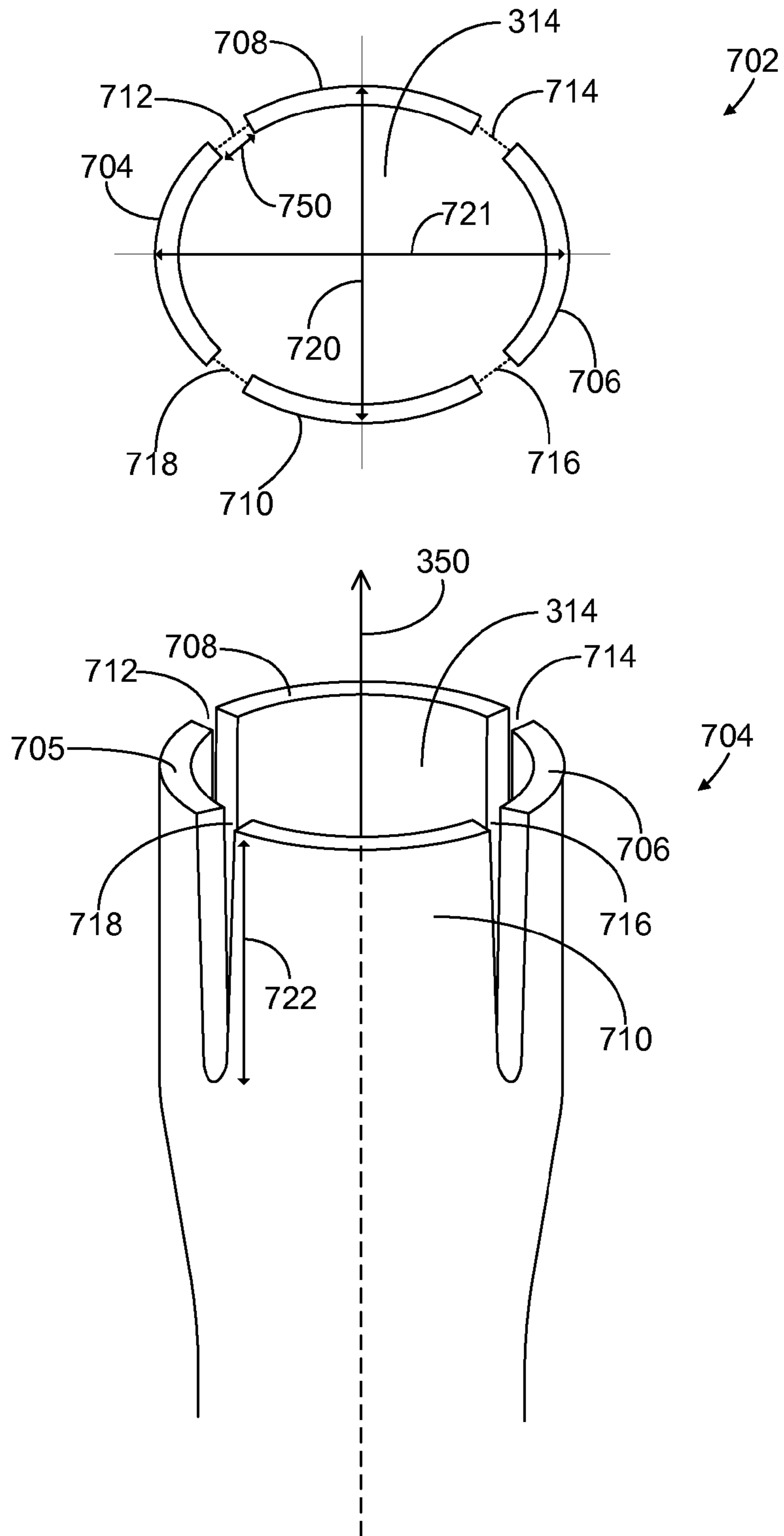
FIG. 7
