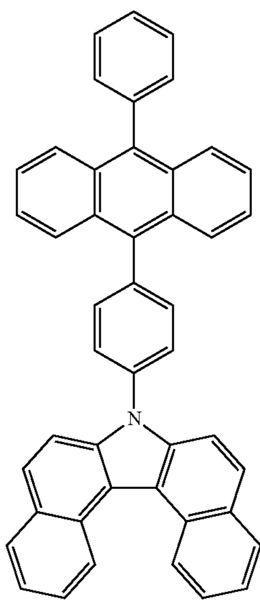
cgDBCzPA
