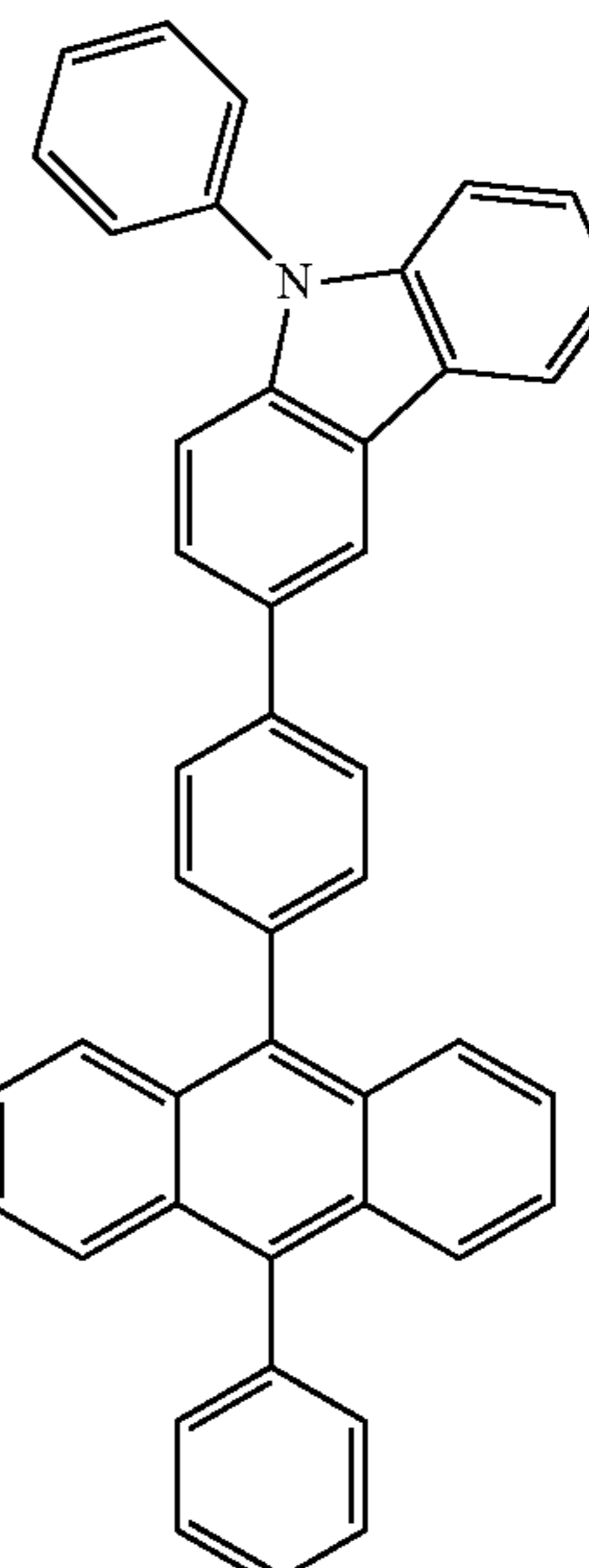
PCzPA
