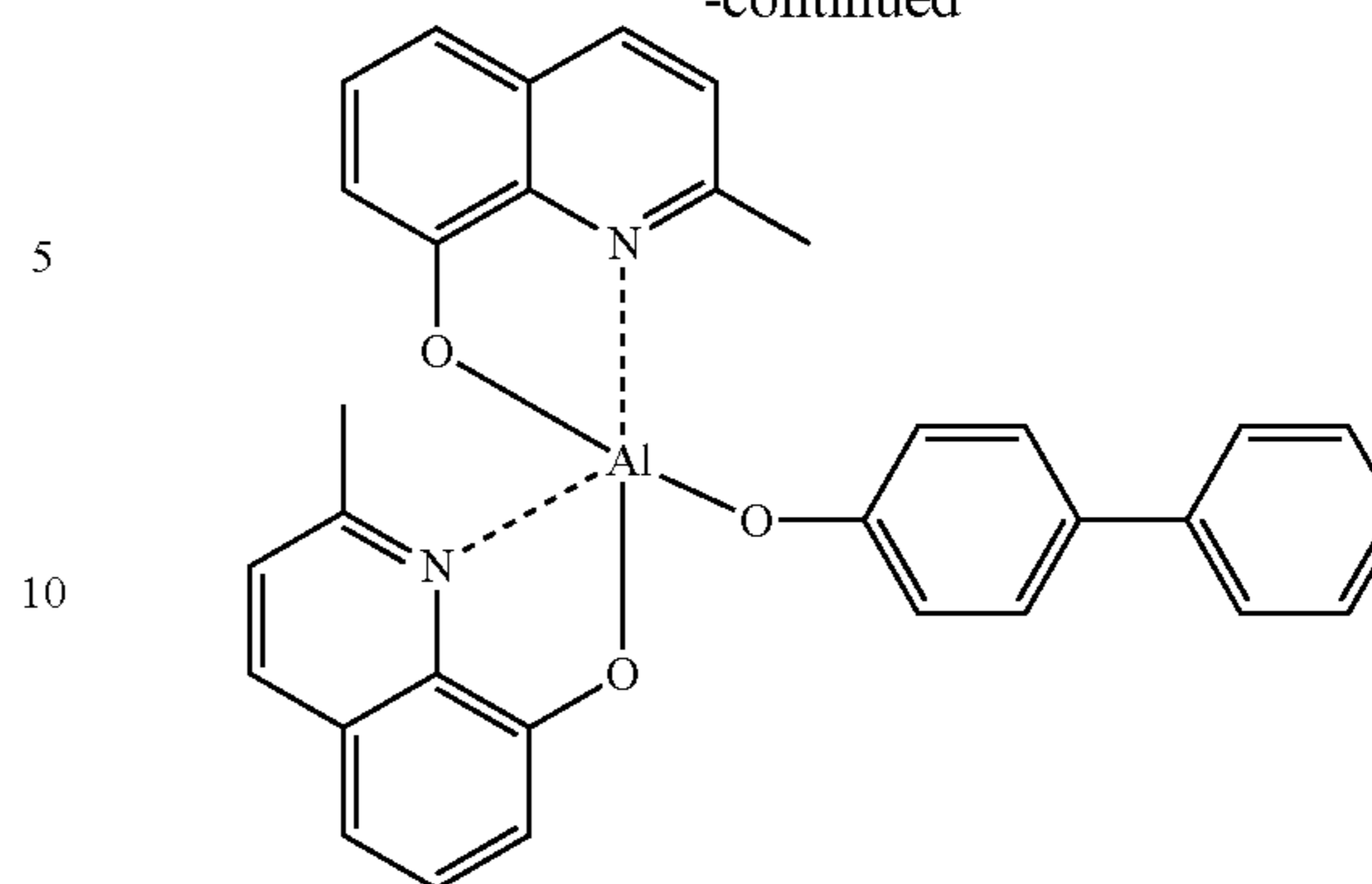
BAAlq
