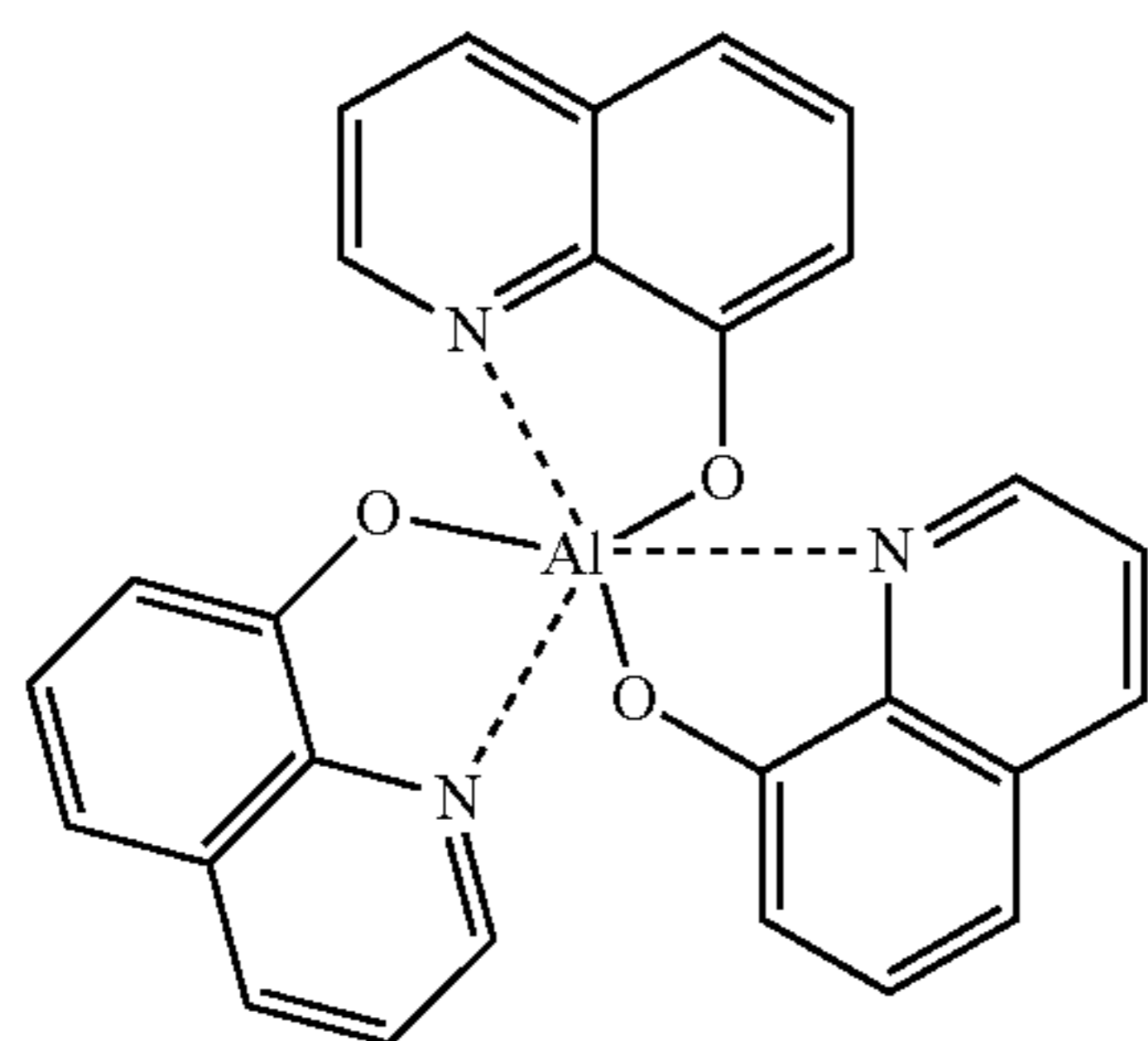
Alq 3
