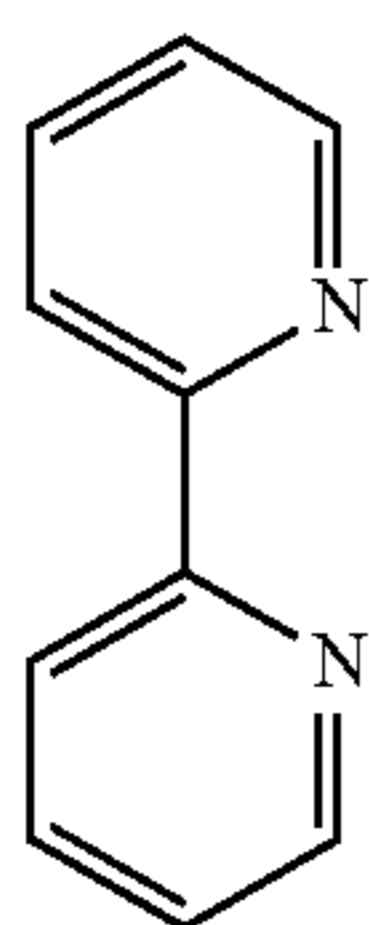
bpy
