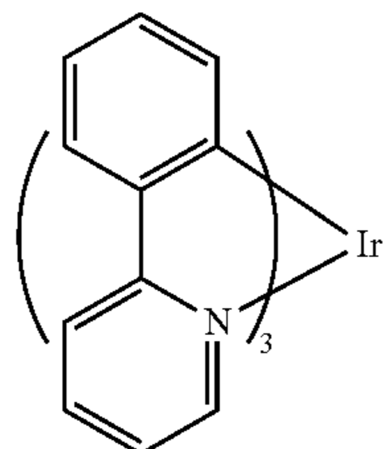
Ir(ppy) 3
