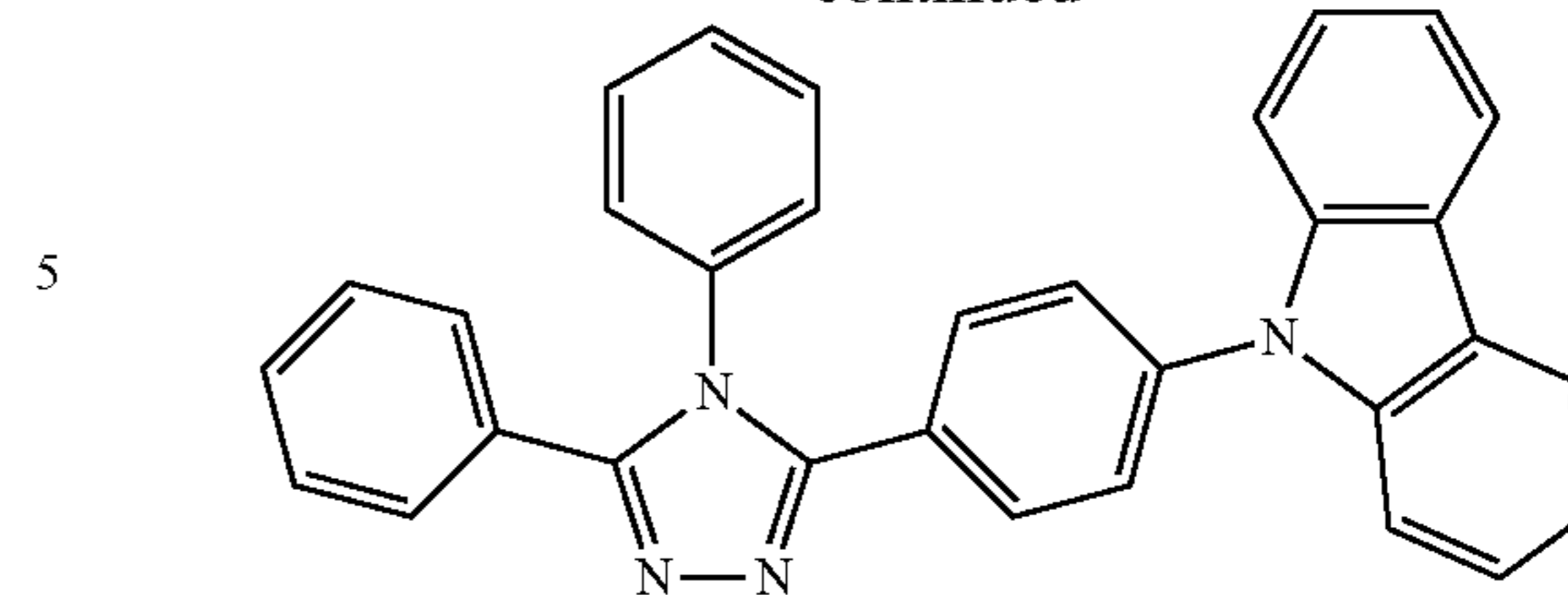
CzTAZ-I
