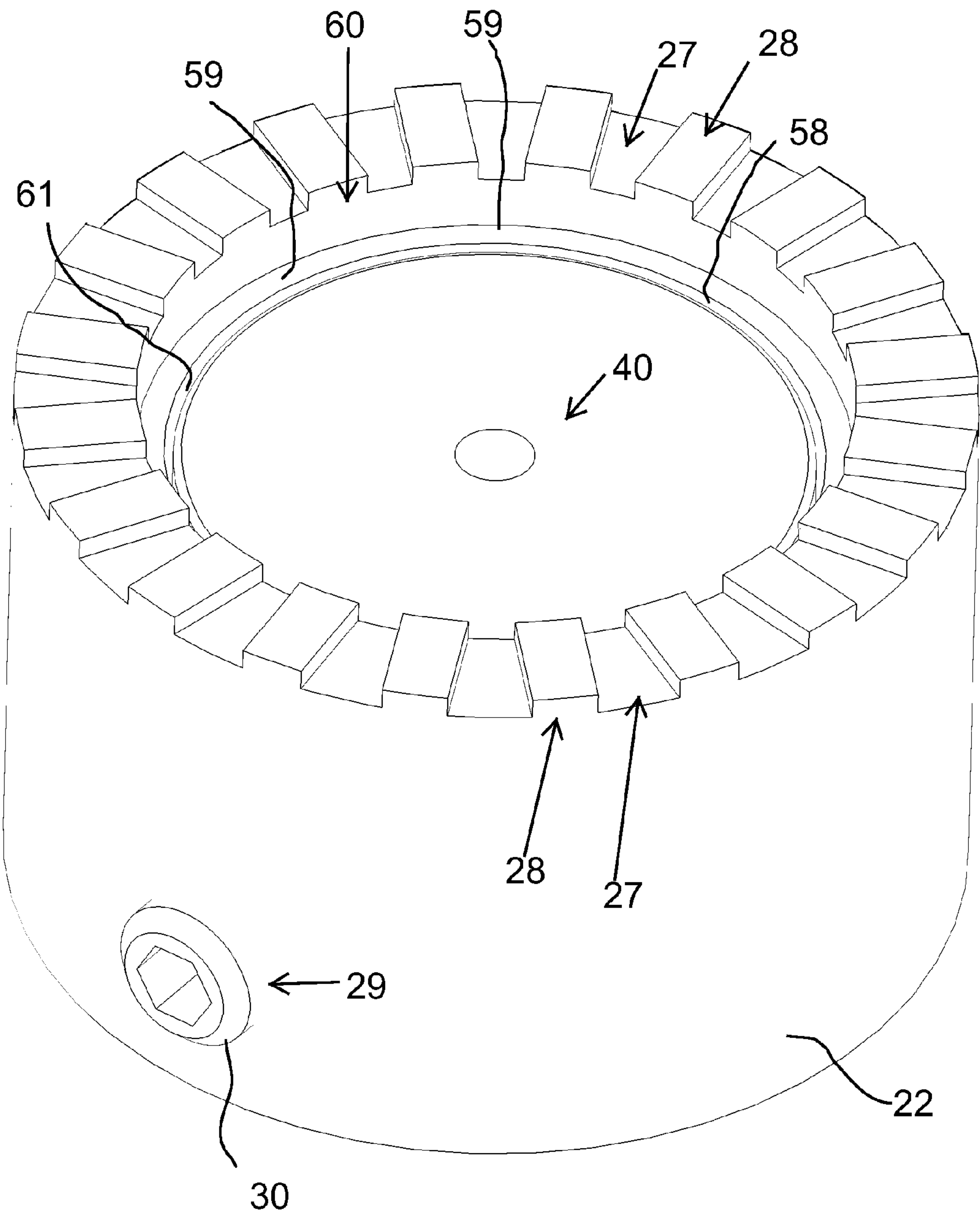
FIG. 6a
