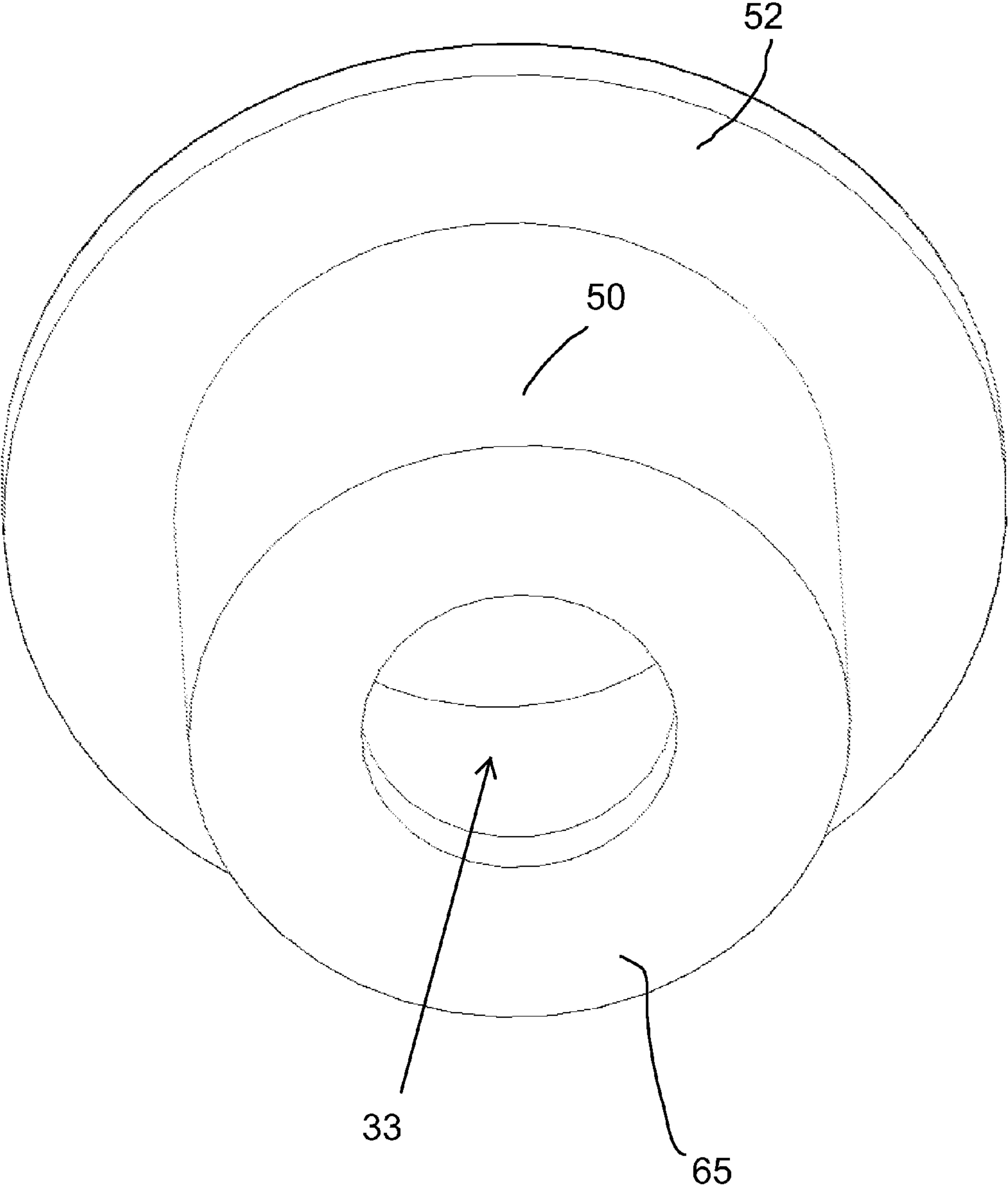
FIG. 10c
