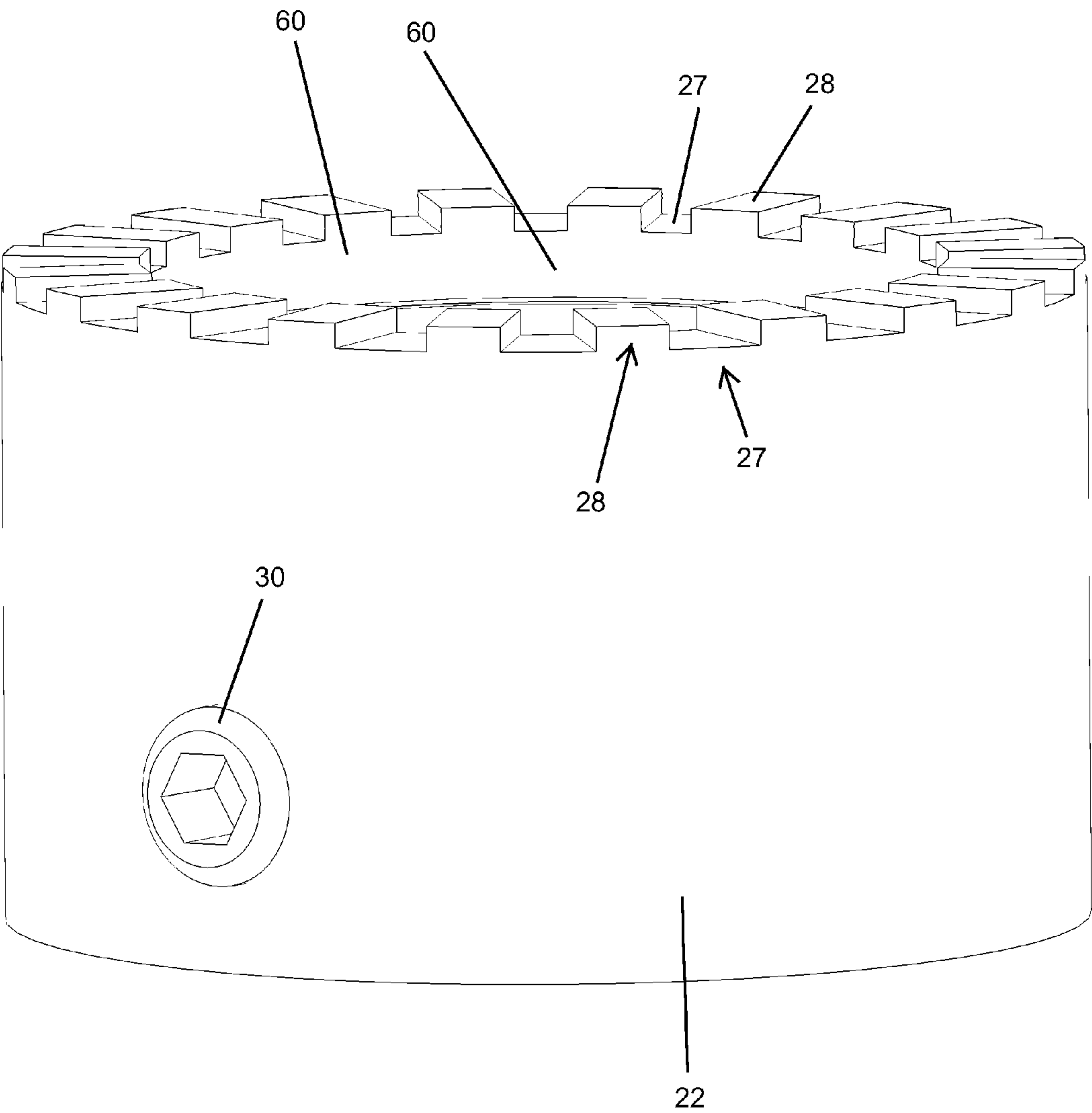
FIG. 6b
