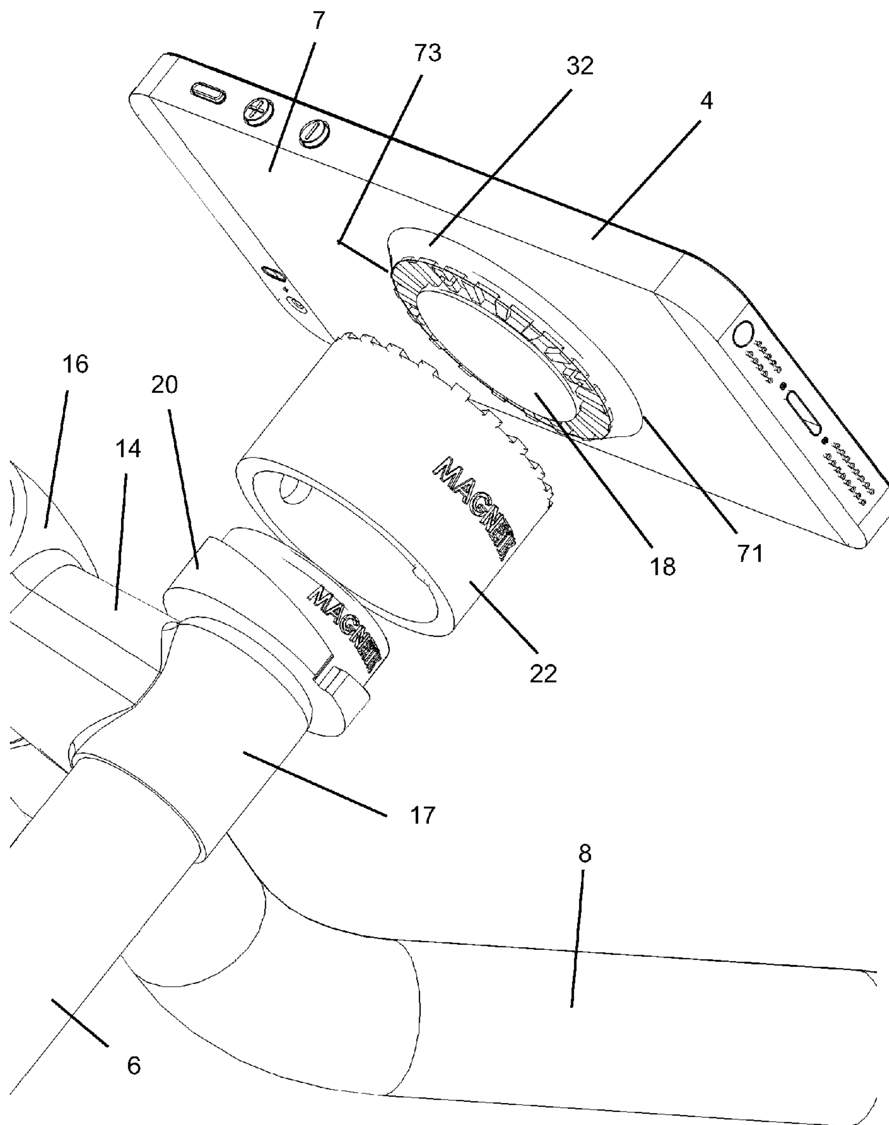
FIG. 1b
