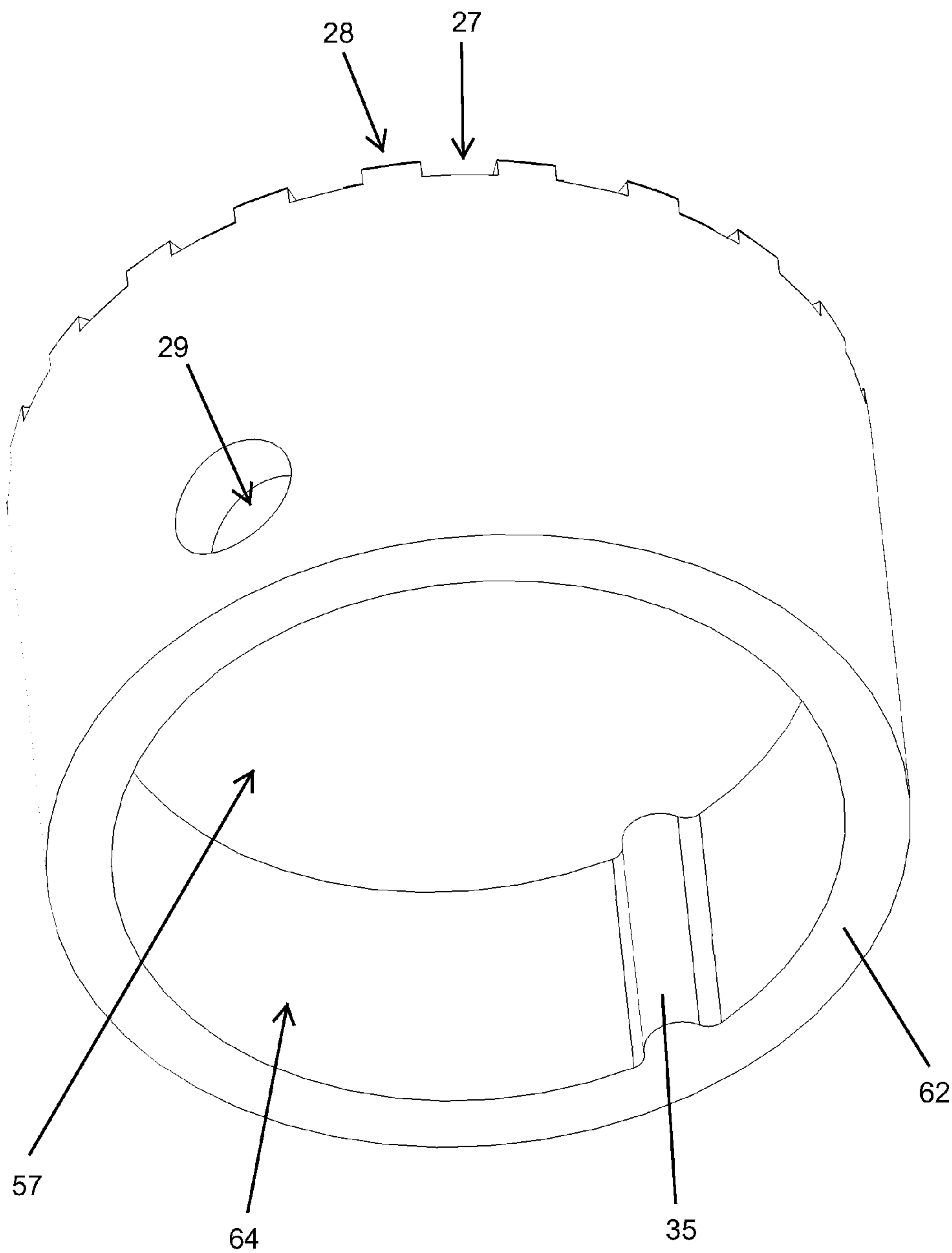
FIG. 7c
