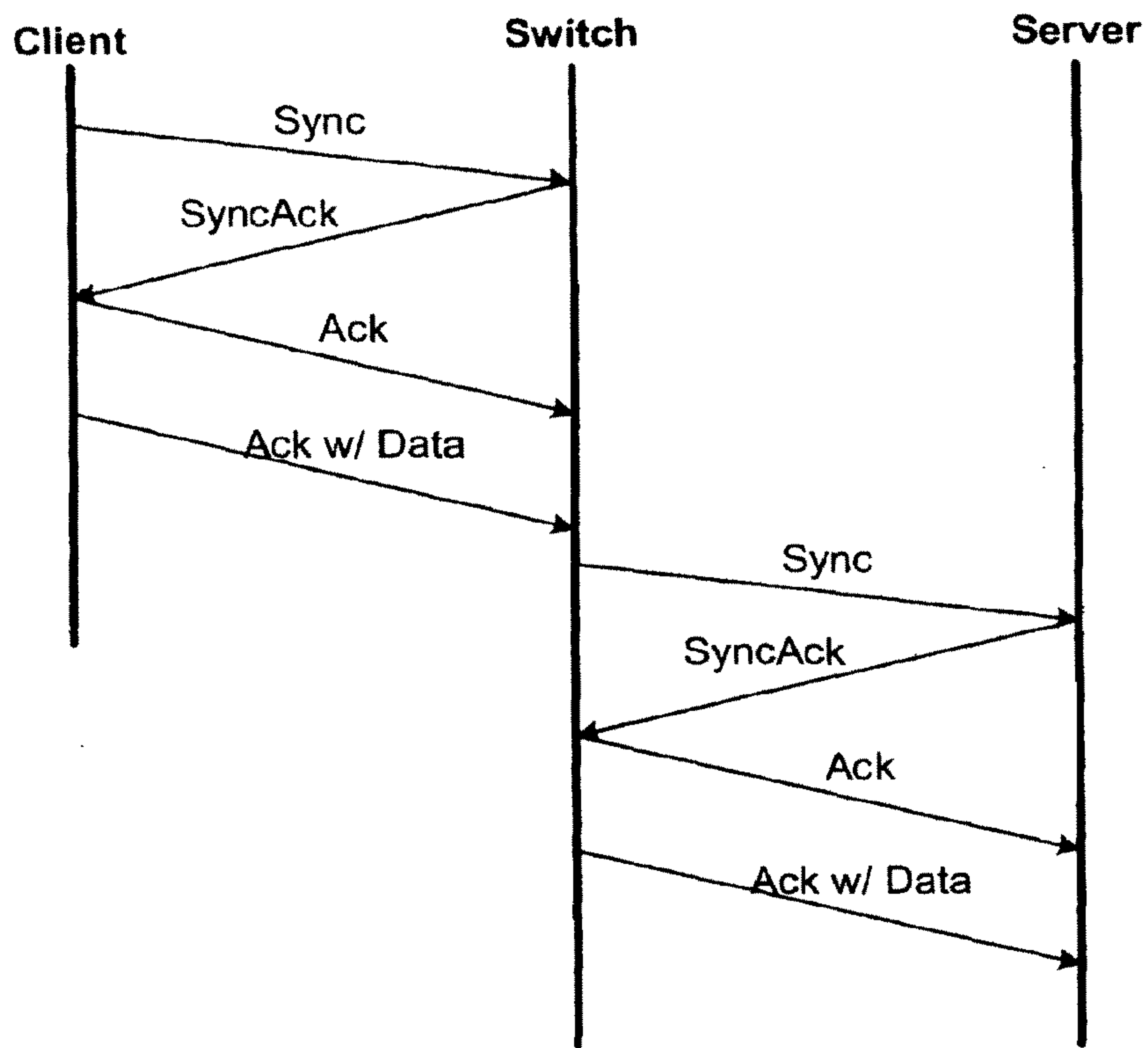
FIG. 17 TCP Slicing
