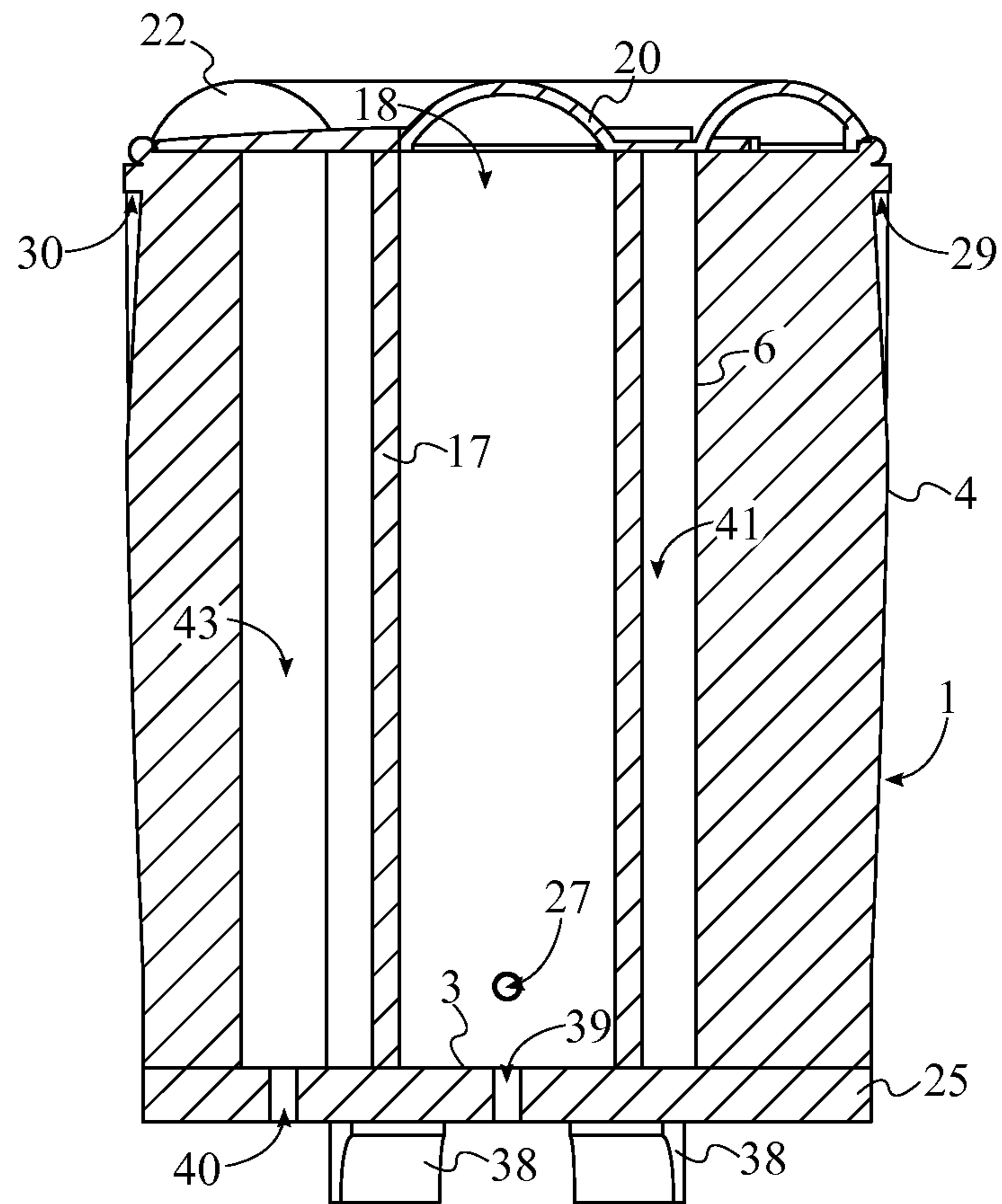
SECTION A-A
