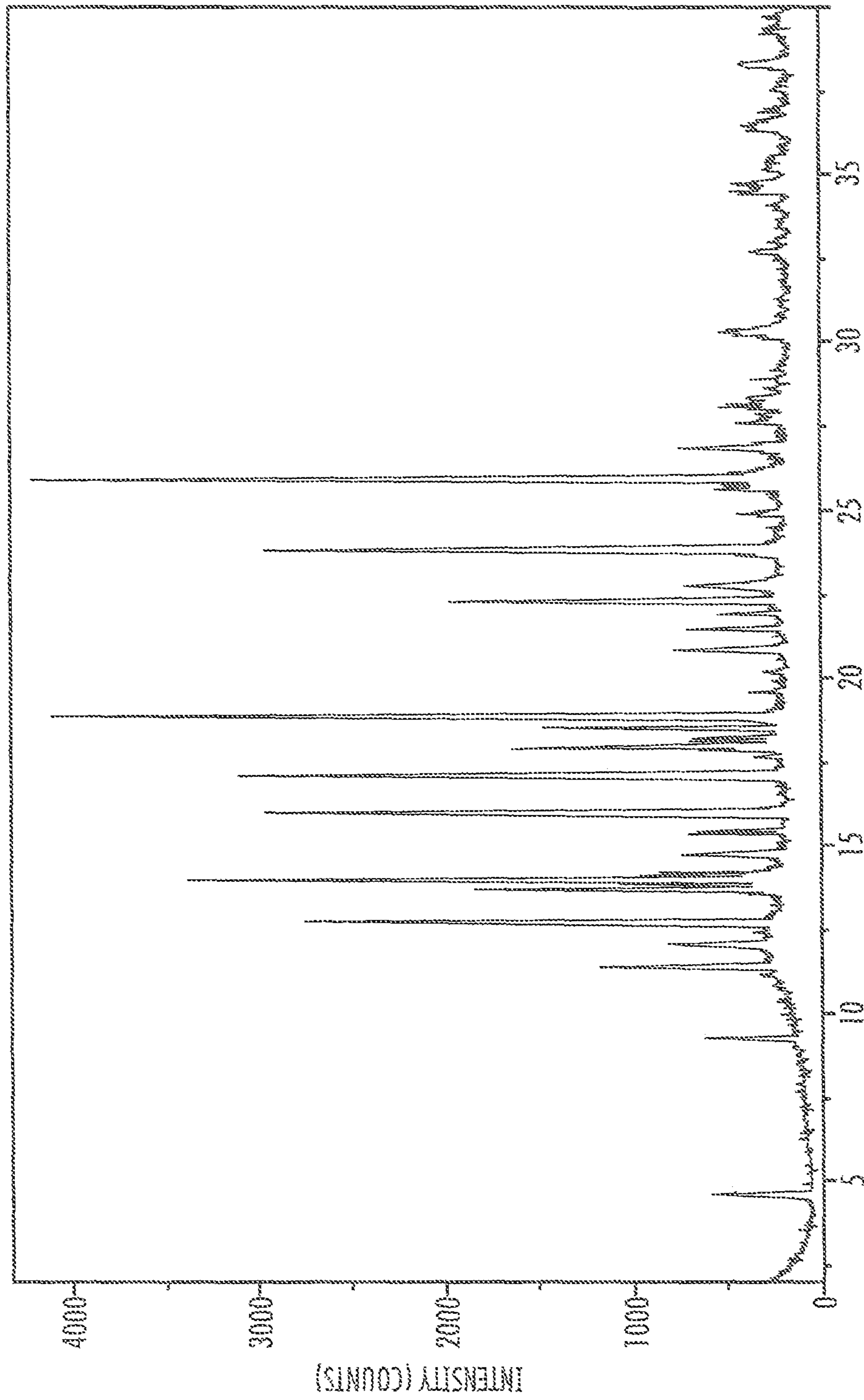
2THETA (°)
