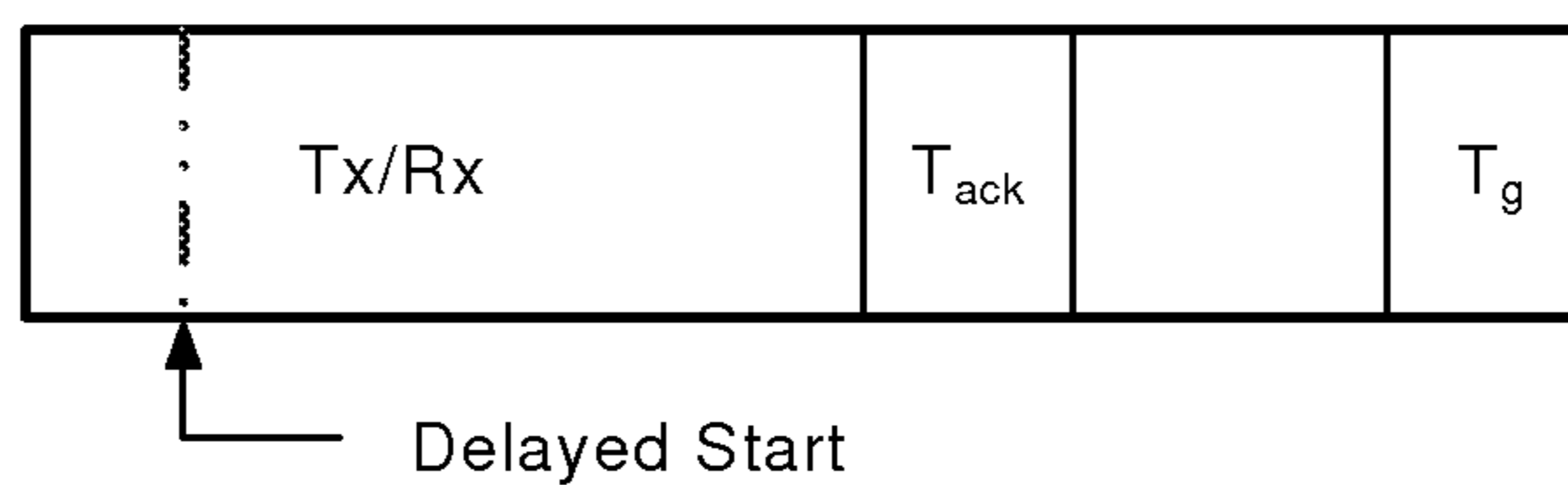
FIG. 5 OR2 Timeslot Format
