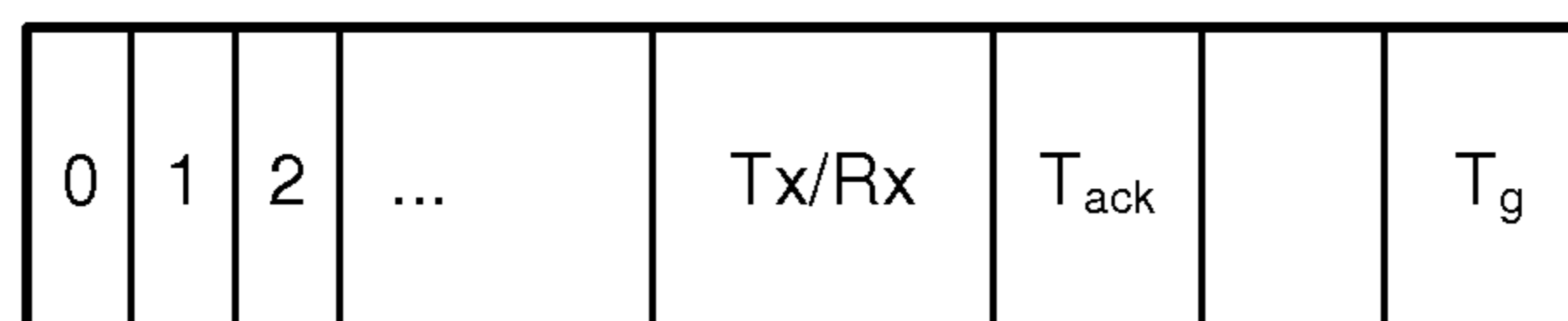
FIG. 4 OR1 Timeslot Format
