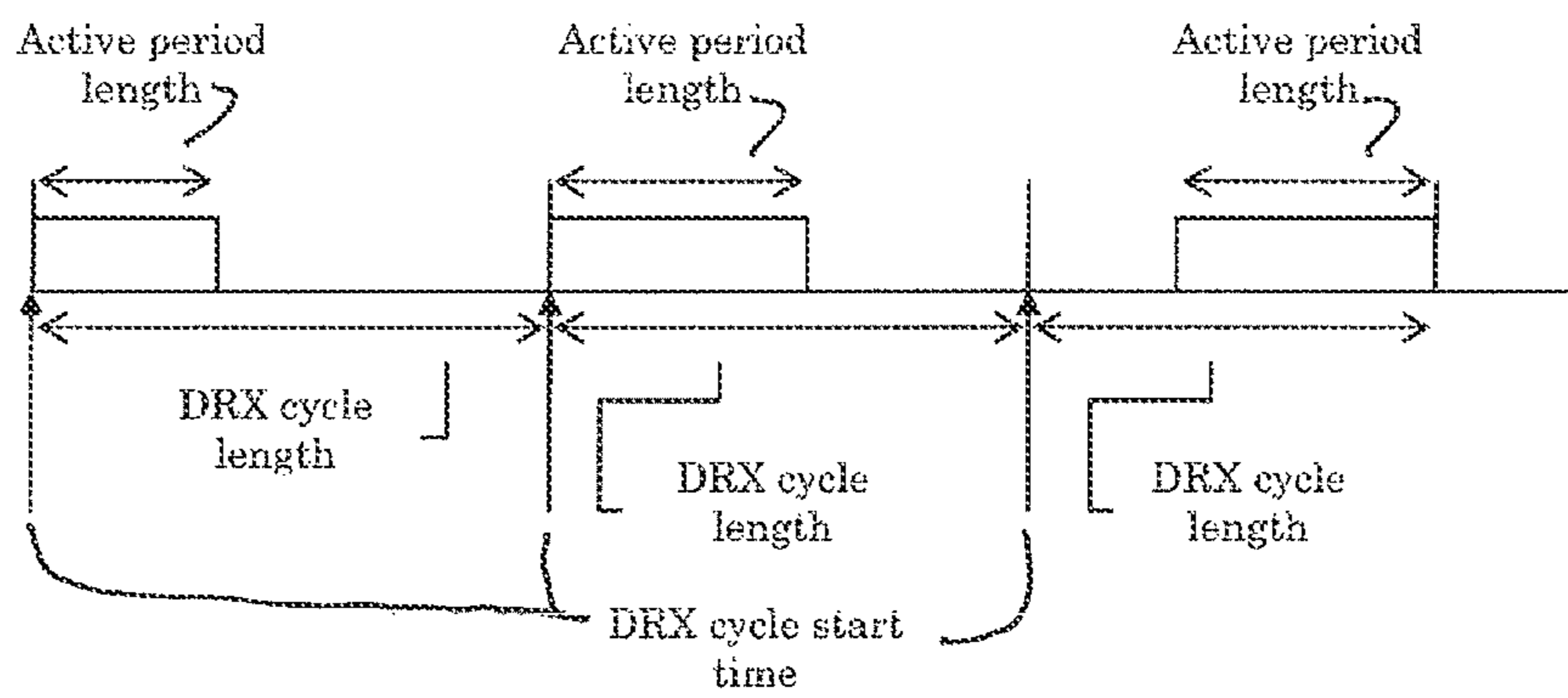
FIG.2
