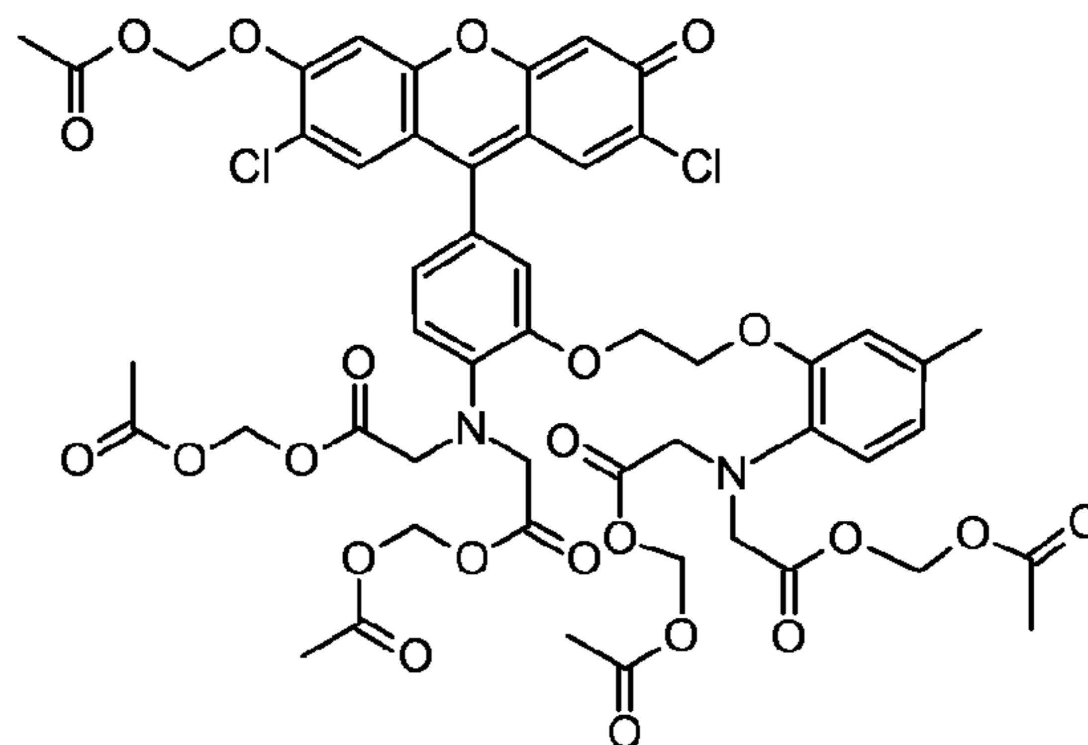
Fluo-3 AM
