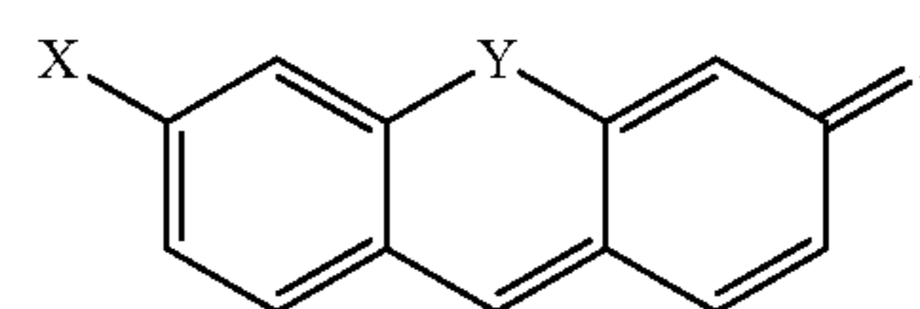
Xanthene
