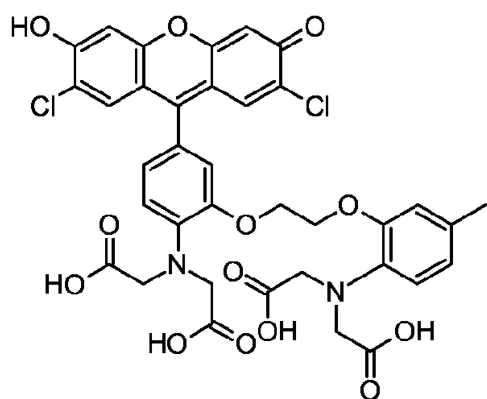
Fluo-3
