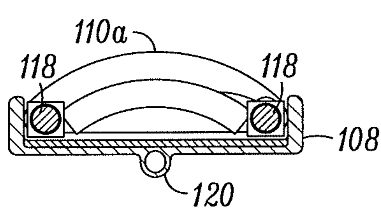
SECTION A-A
