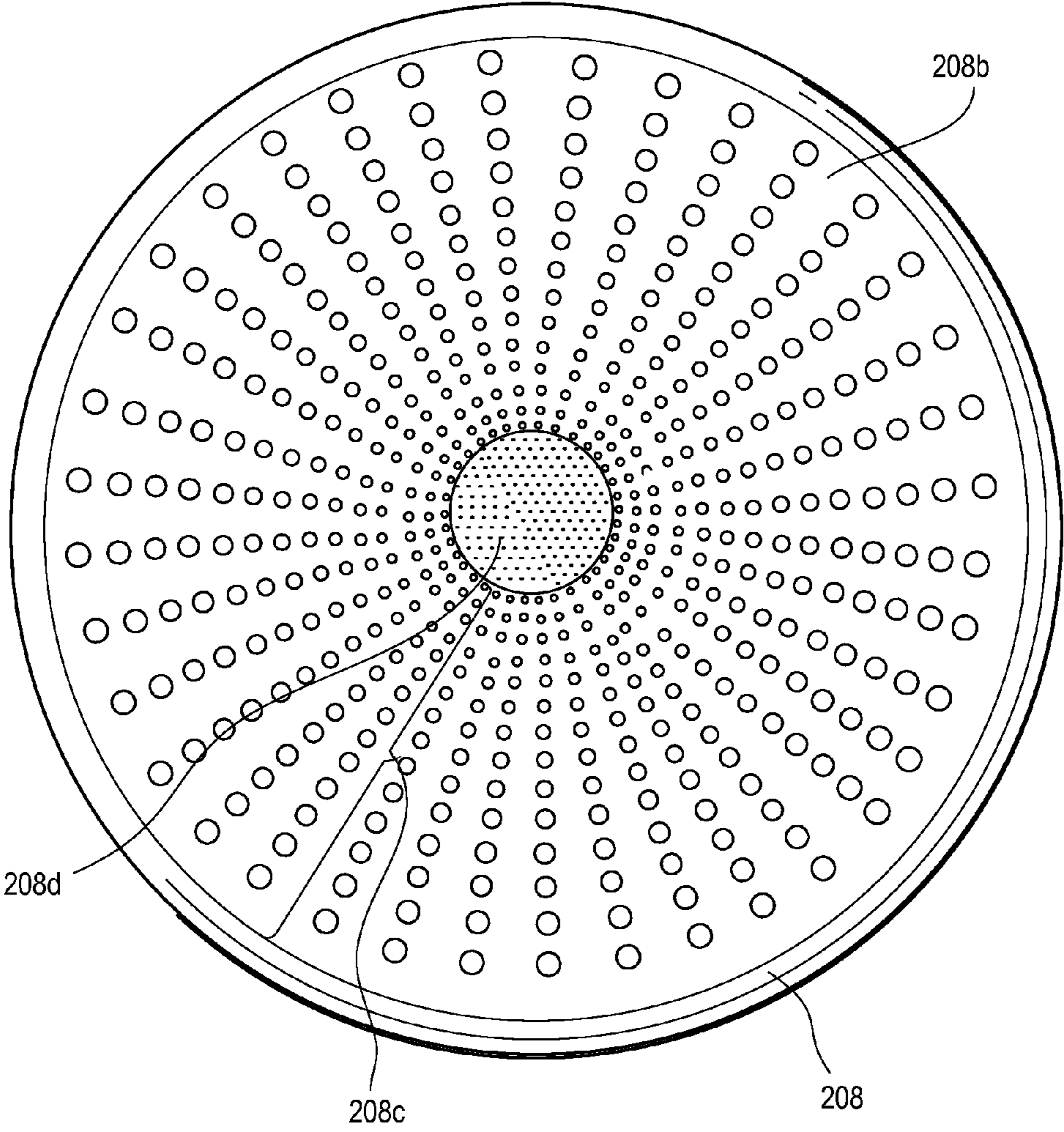
FIG. 2C
