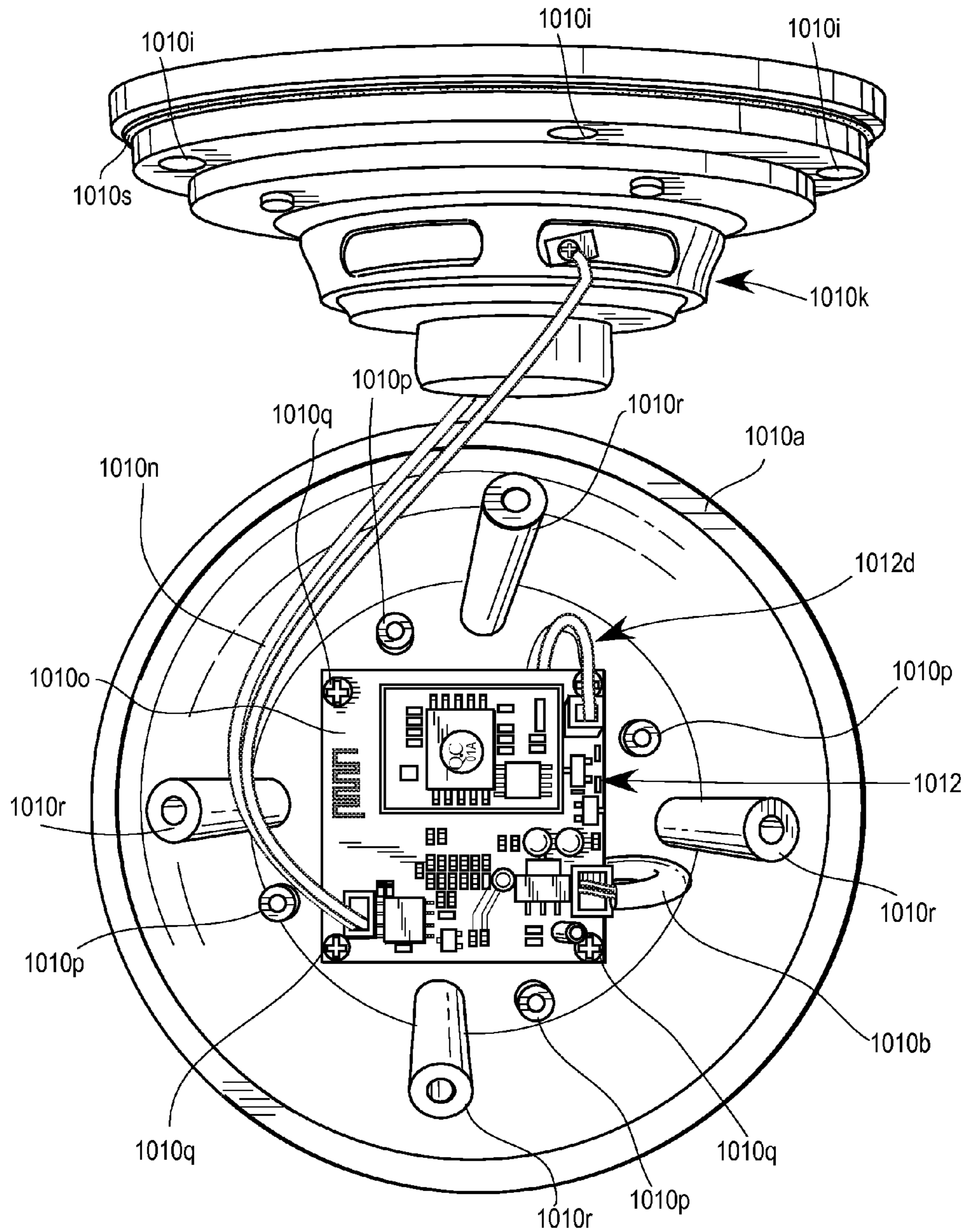
FIG. 10C
