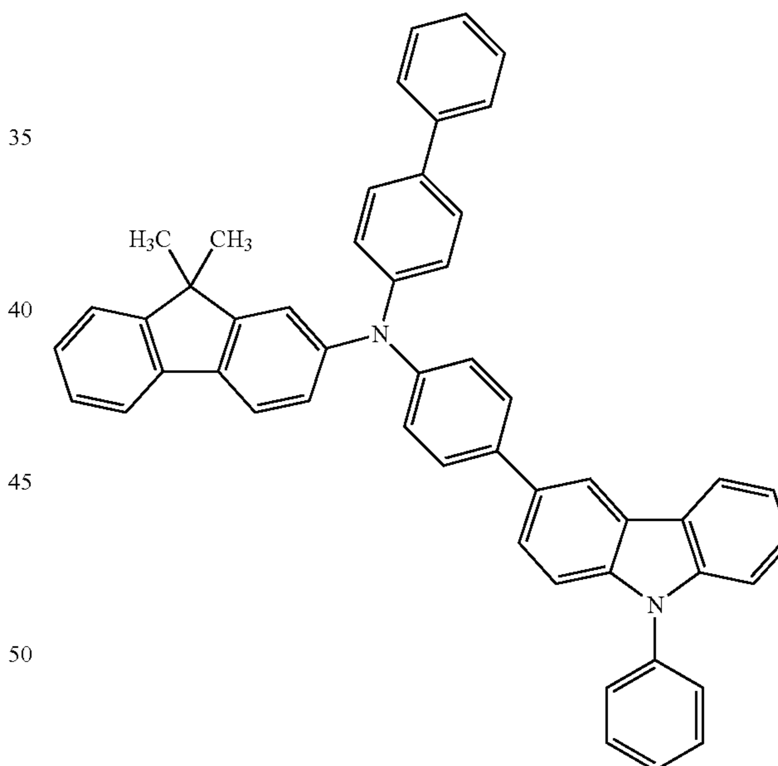
PCBBiF
