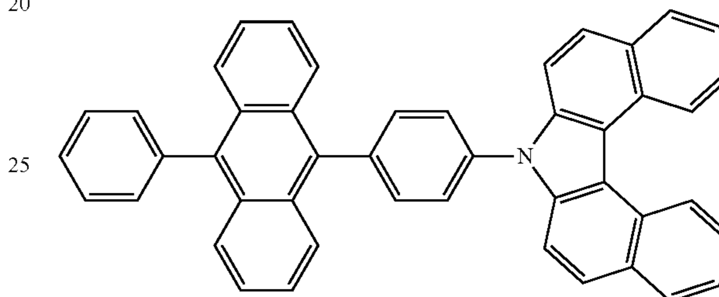
cgDBCzPA
