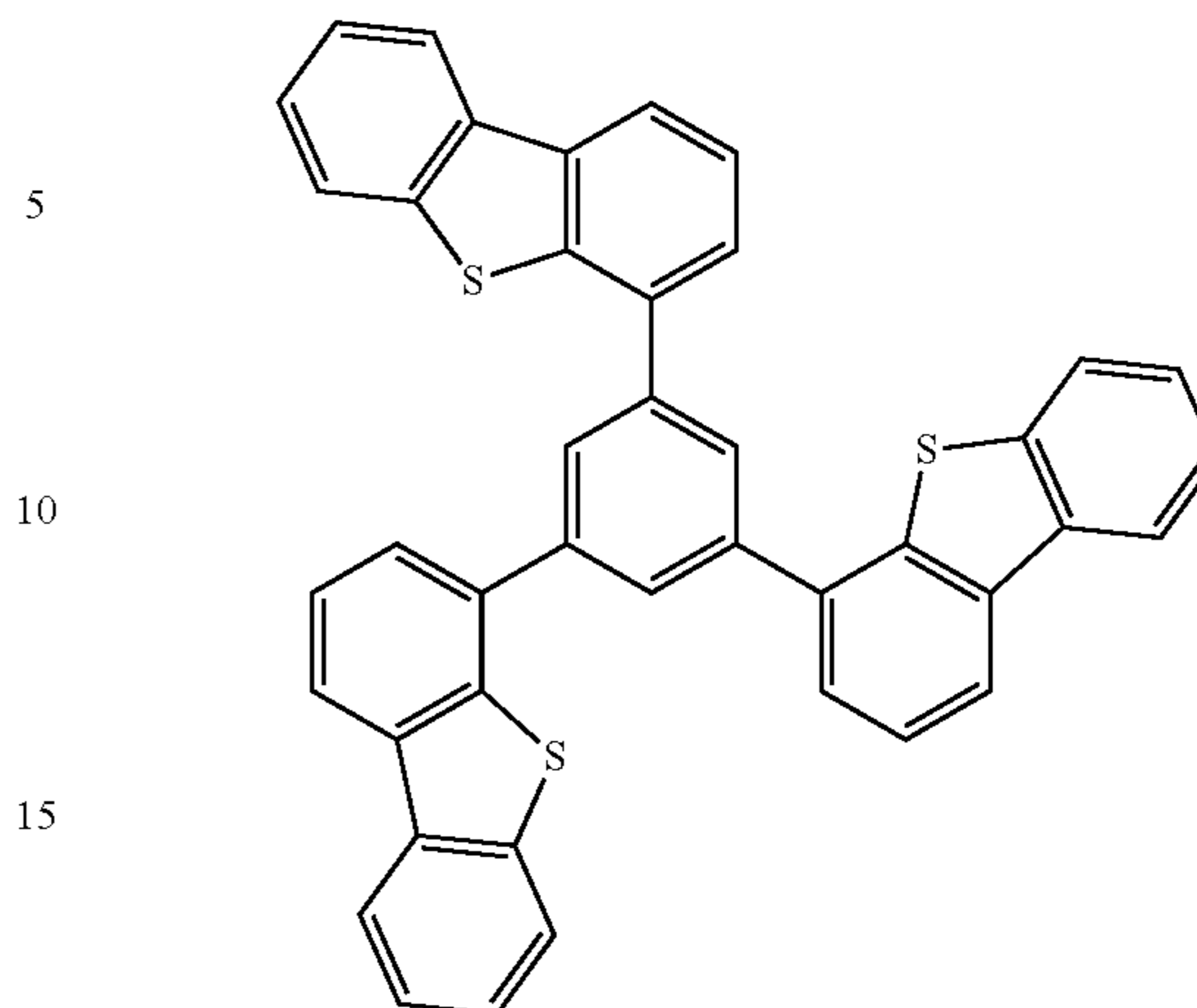
DPT3P-II
