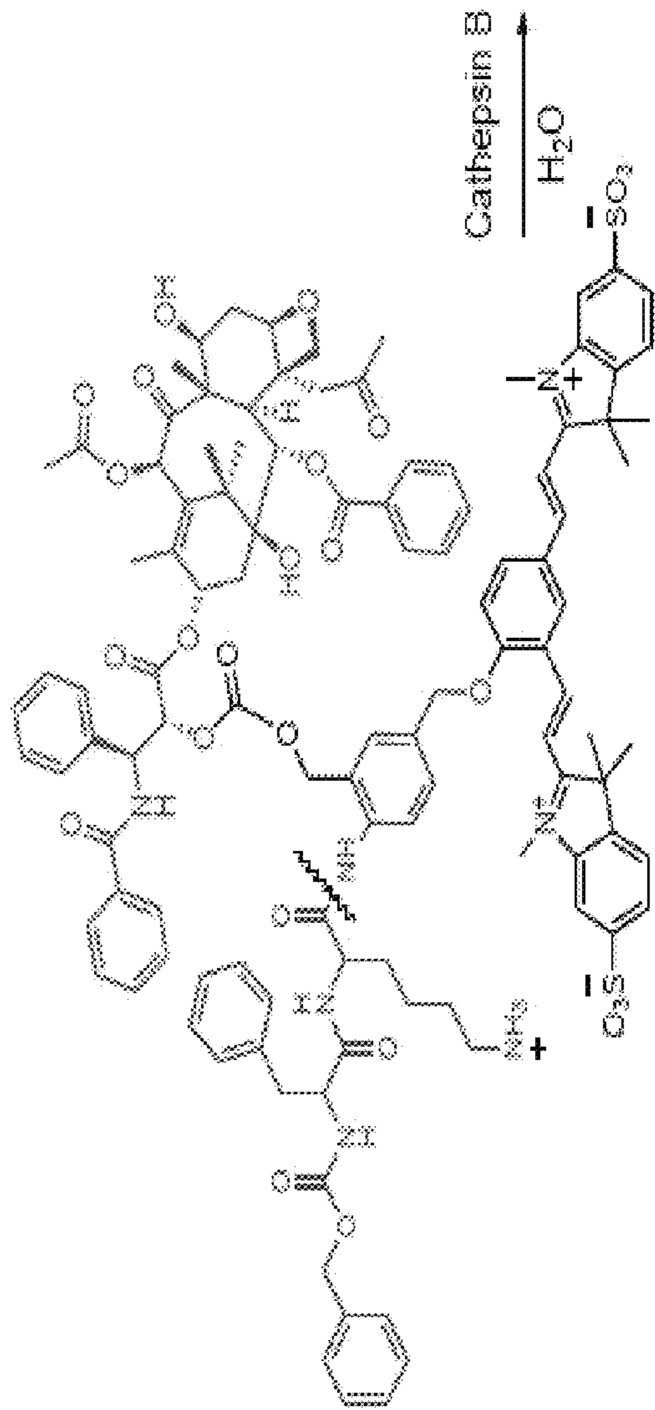
Prodrug 43
