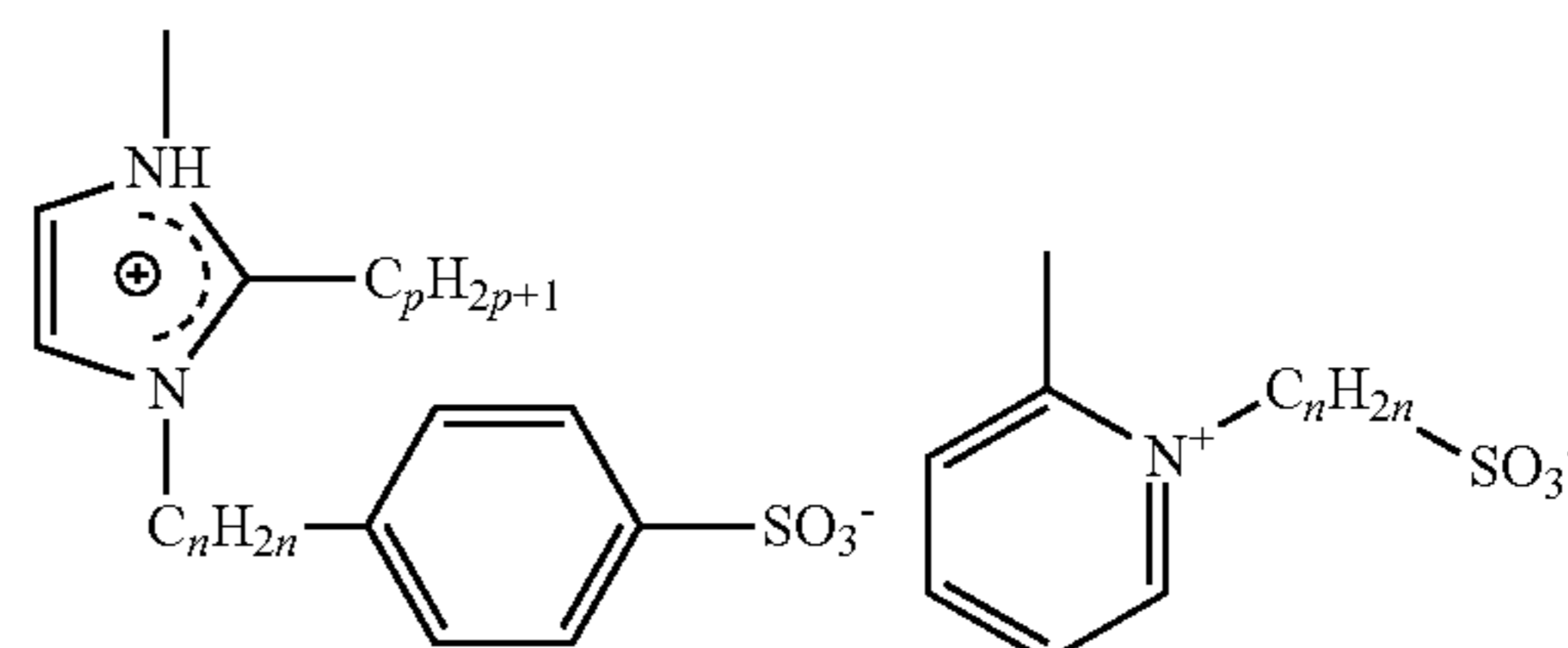
Sulfoaryl imidazolium salts
