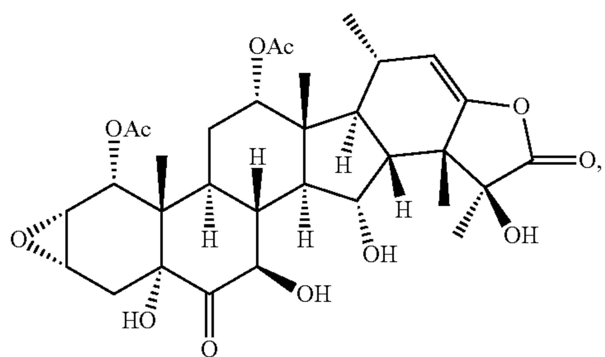
Taccalonolide AL
