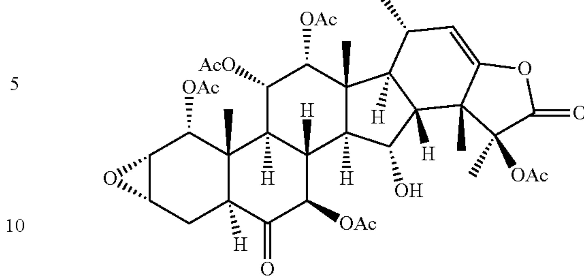
TB-Ac-16
