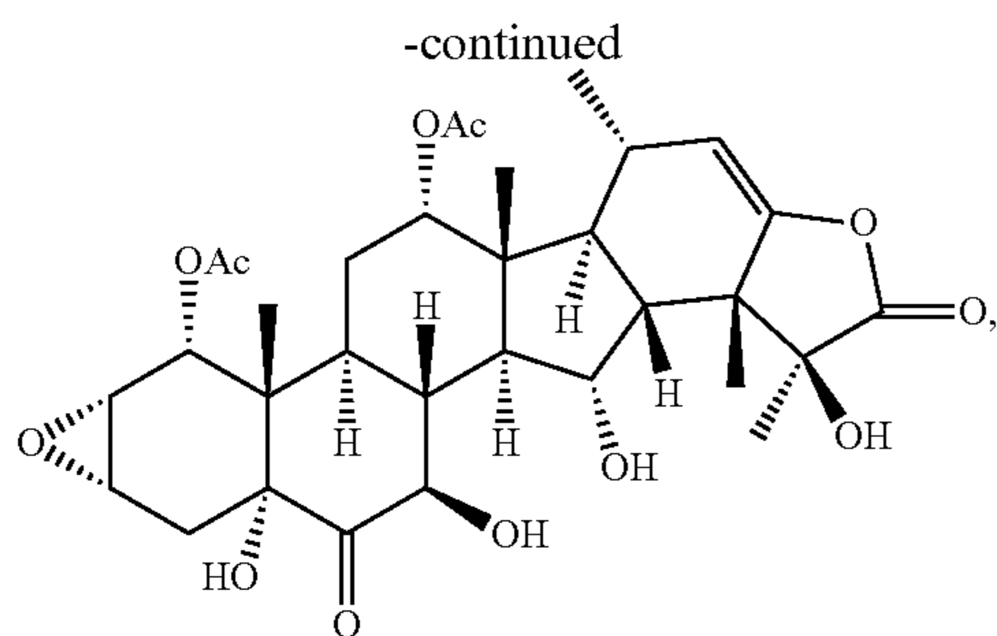
Taccalonolide AL
