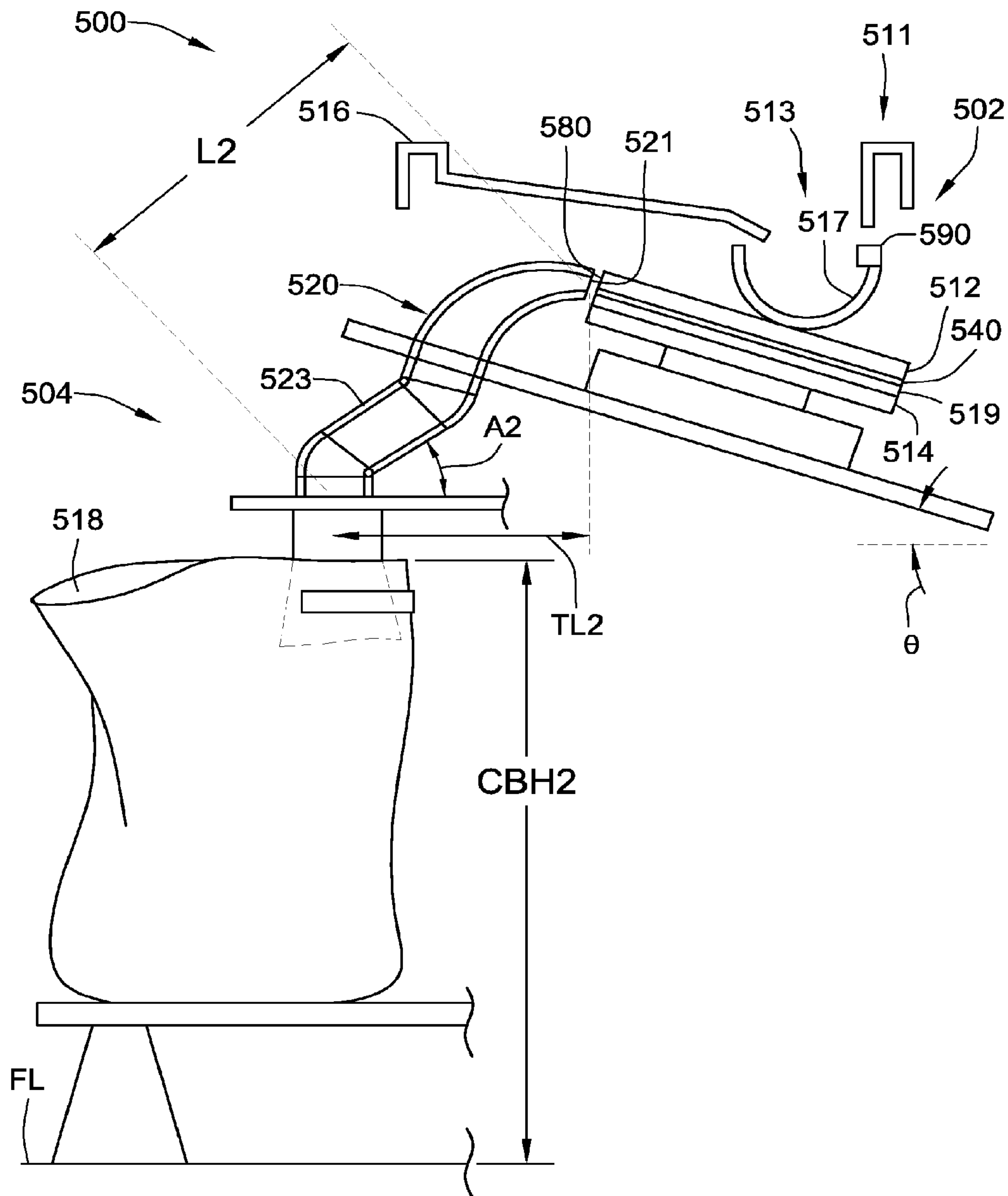
FIG. 8
