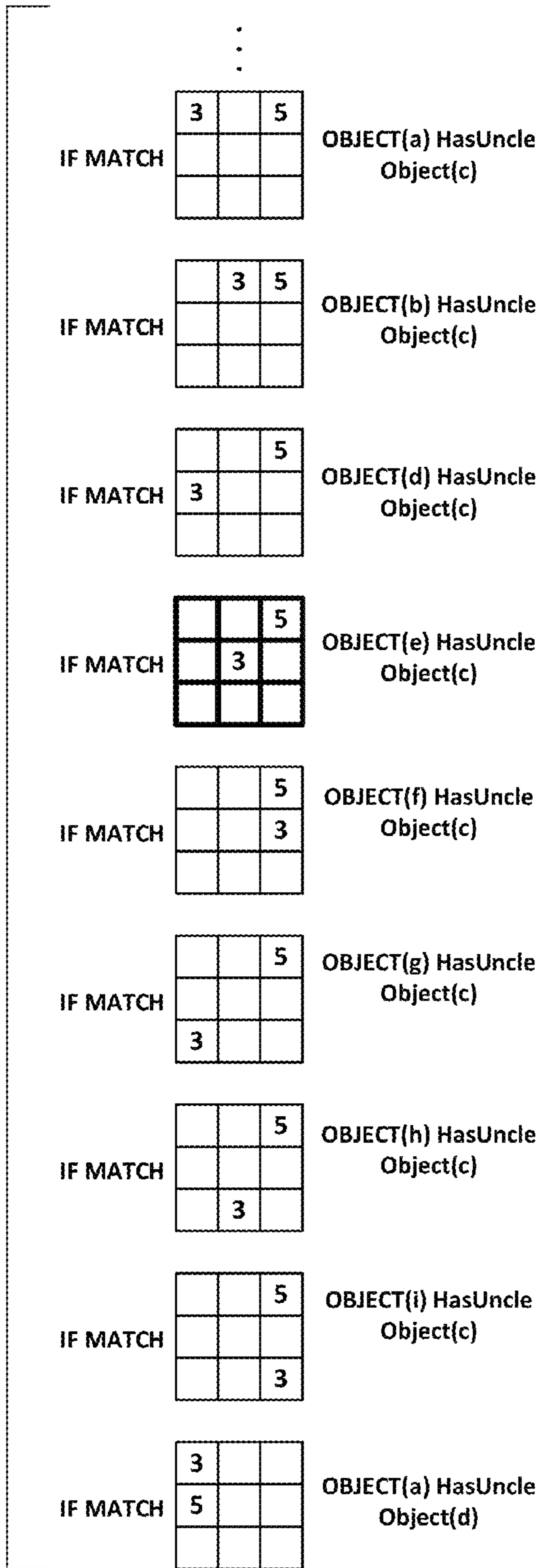
FIG. 26 – PREDICATE TEMPLATES
