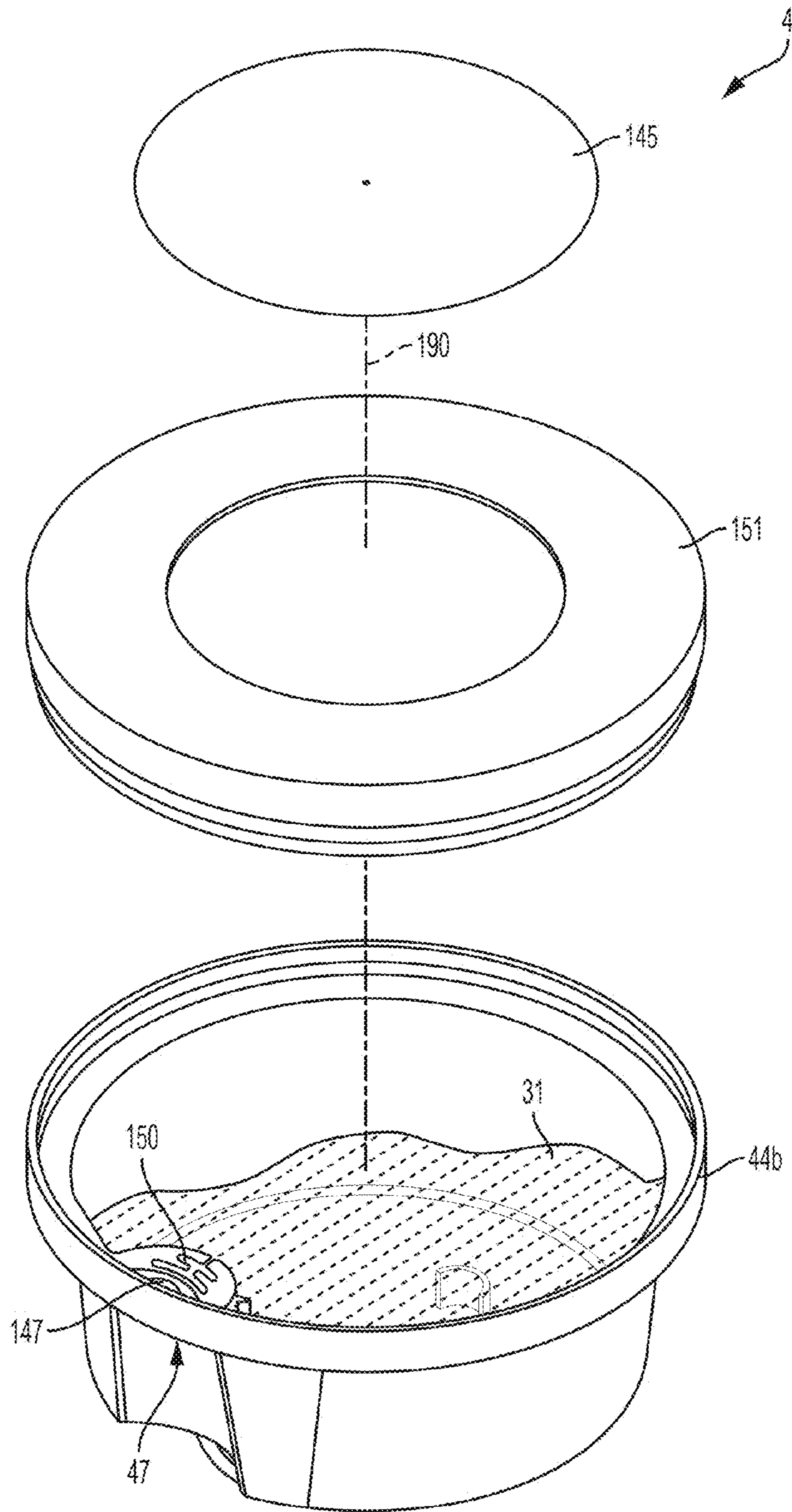
FIG. 18
