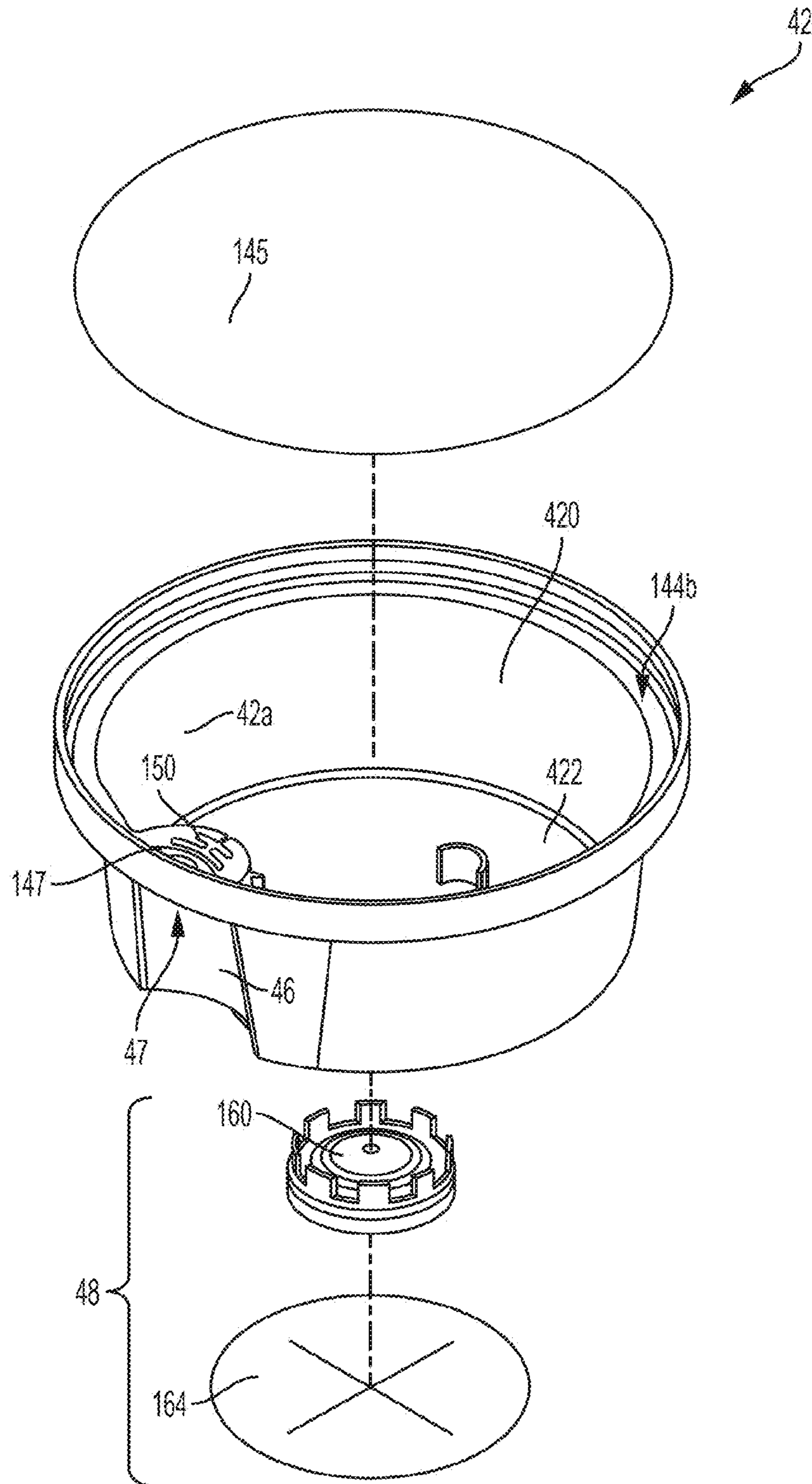
FIG. 5
