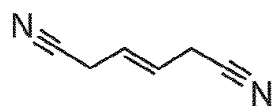
15 D trans-3-hexenedinitrile
