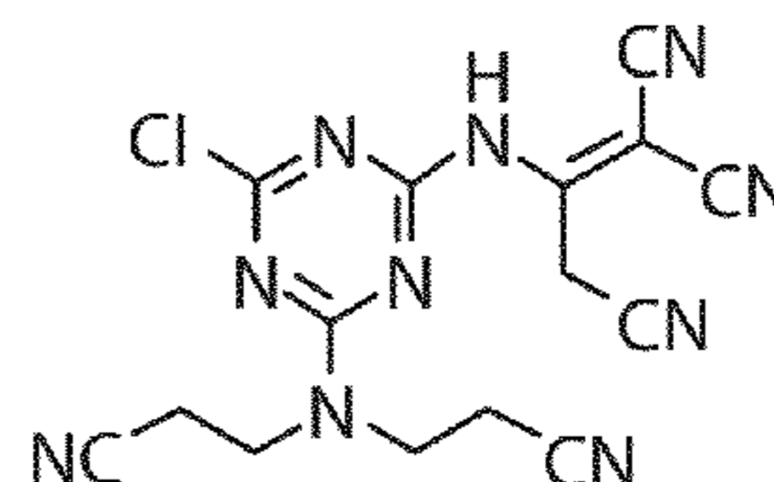
2-((4-(bis(2-cyanoethyl)amino)-6-chloro-1,3,5-triazin-2-yl) amino)prop-1-ene-1,1,3-tricarbonitrile
