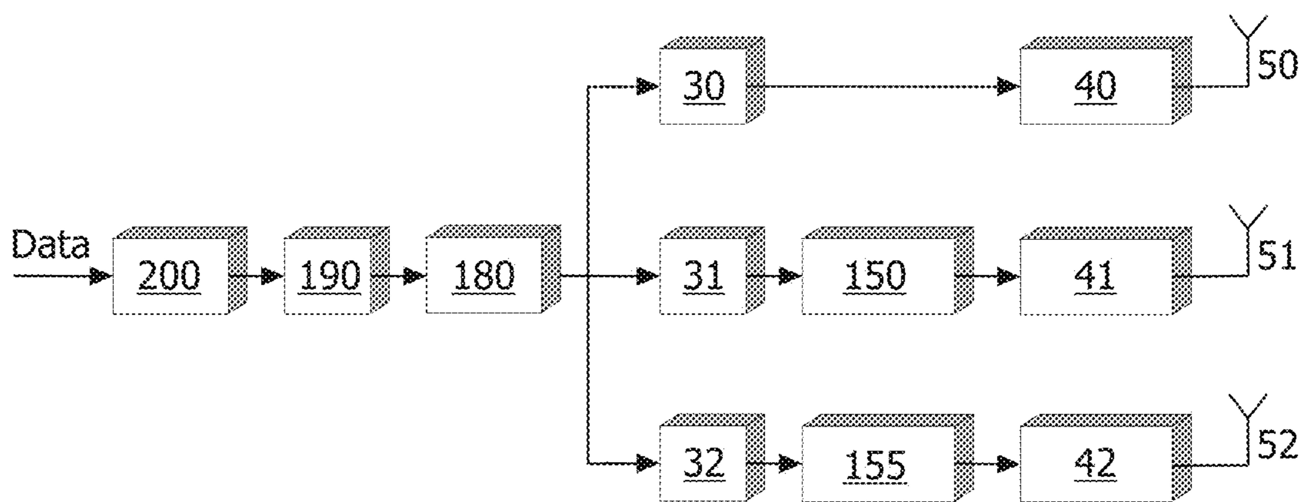
FIG. 15
