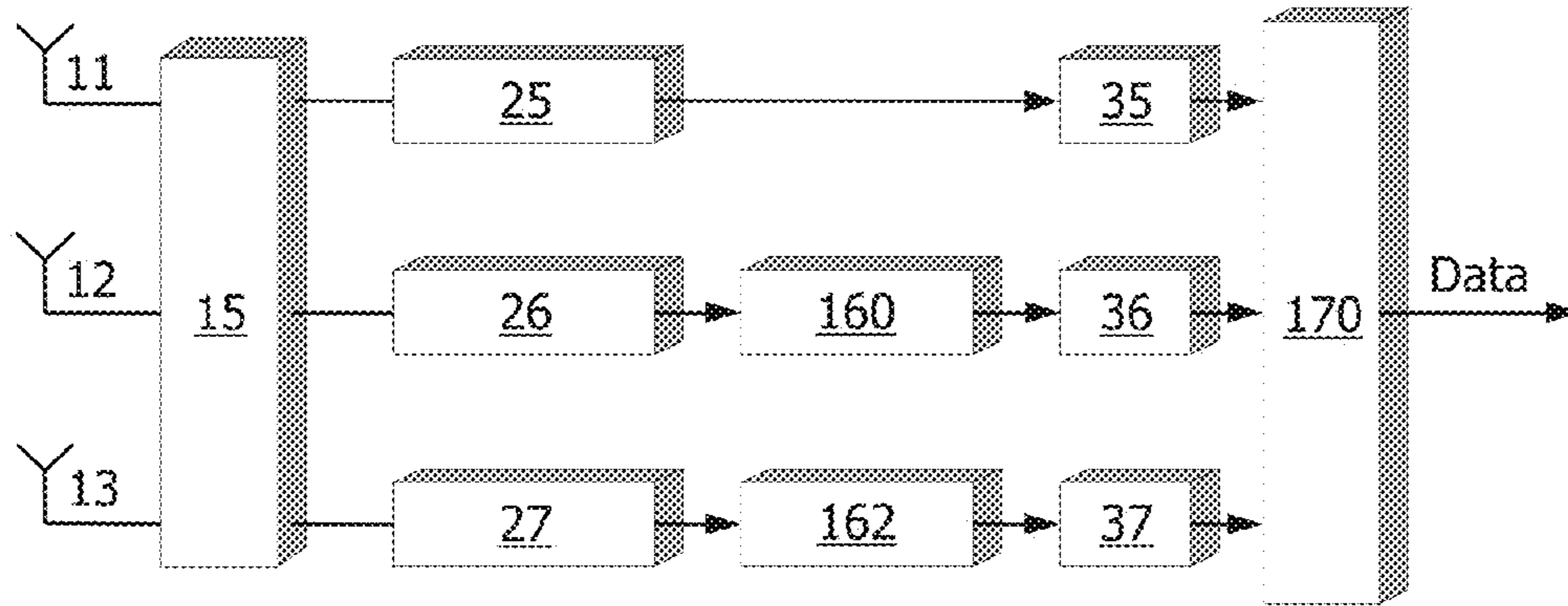
FIG. 11
