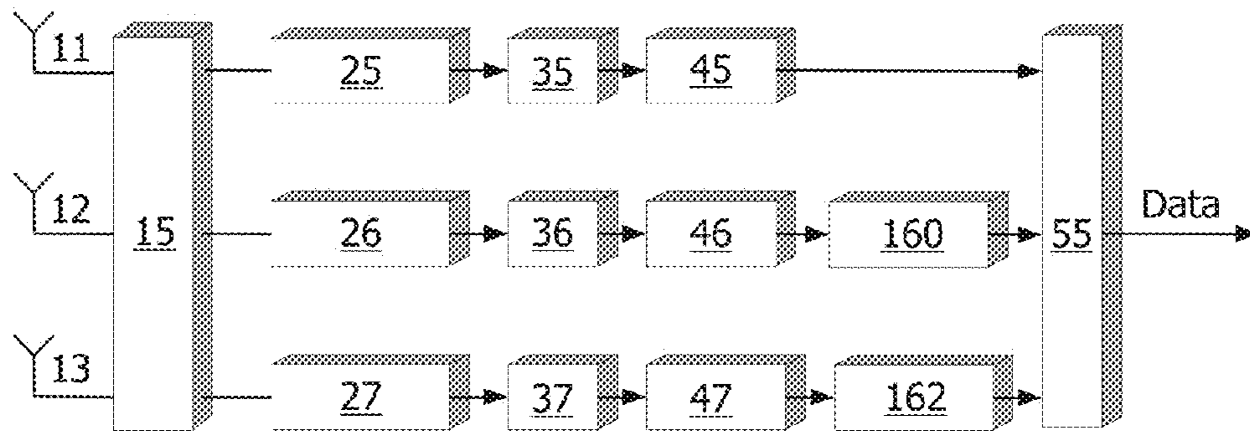
FIG. 8
