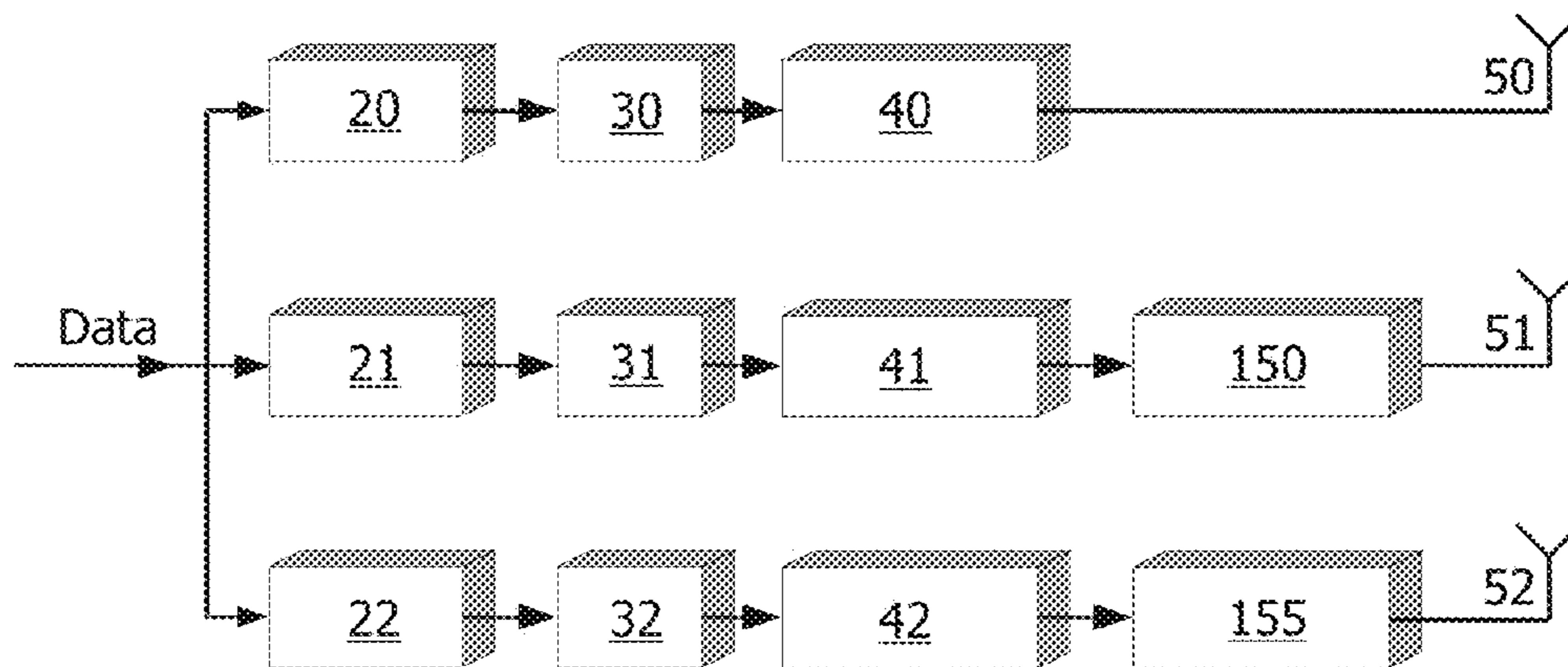
FIG. 12
