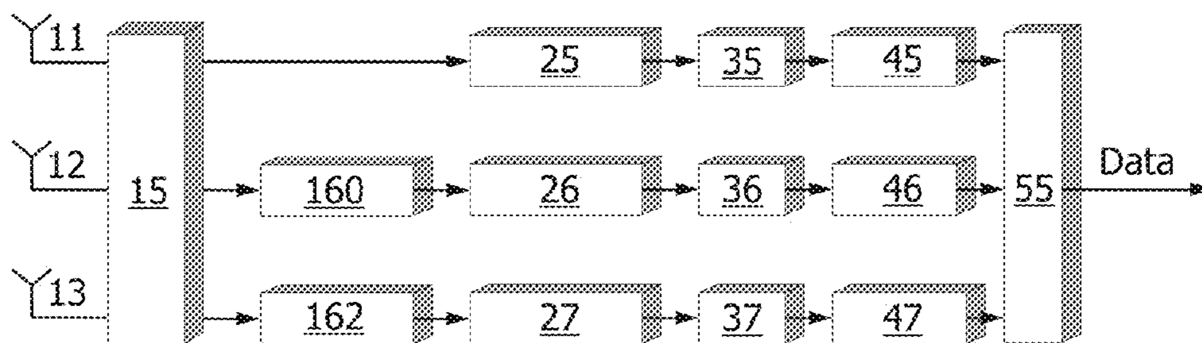
FIG. 13
