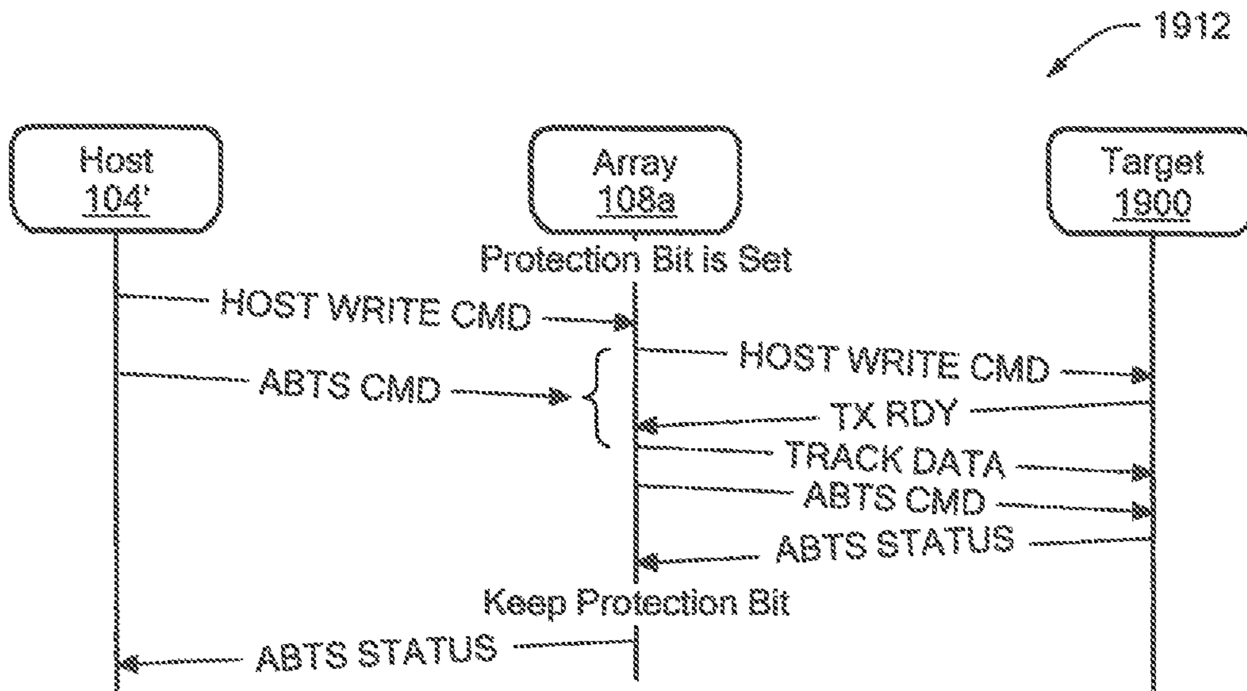
FIG. 19E
