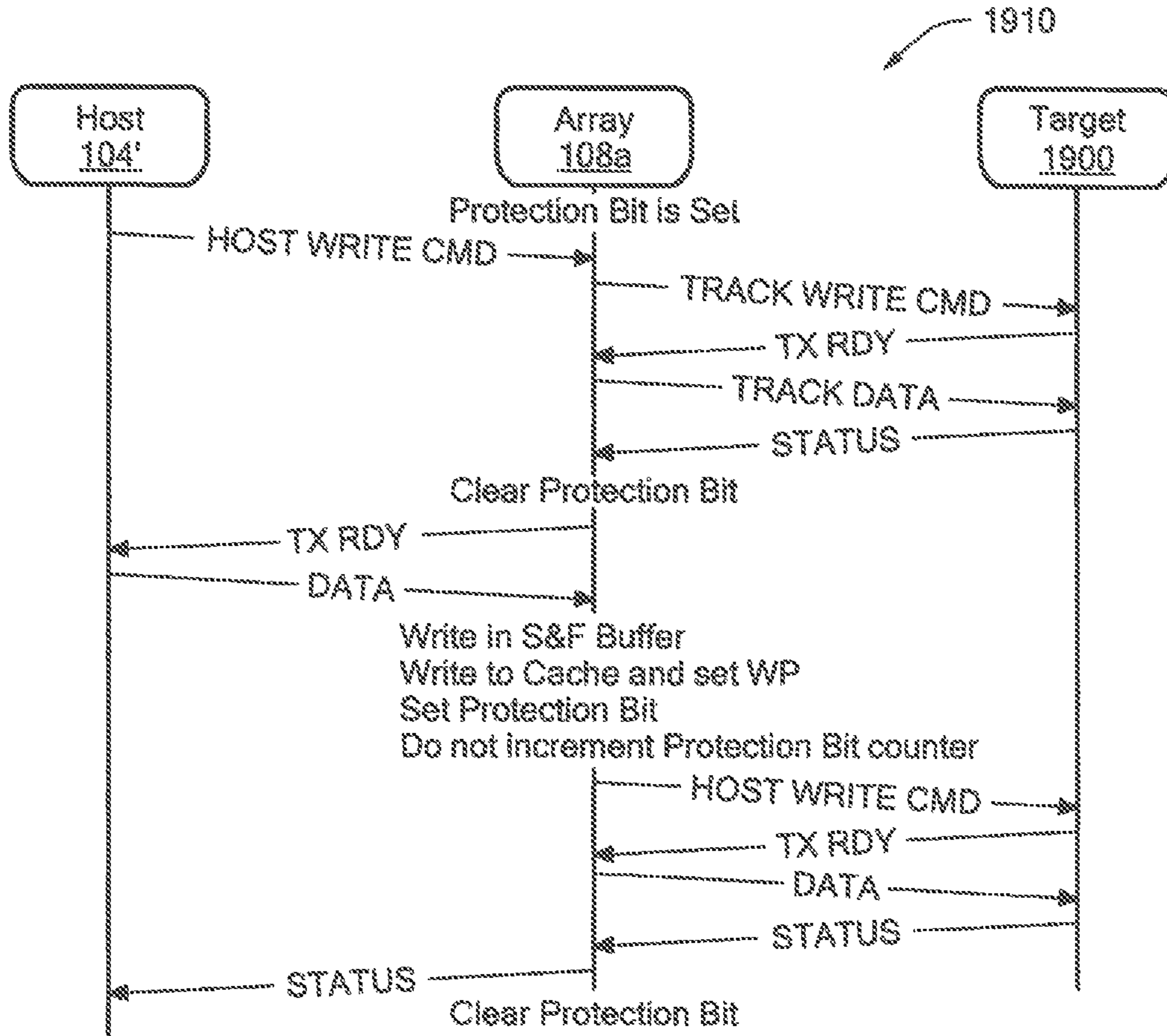
FIG. 19E
