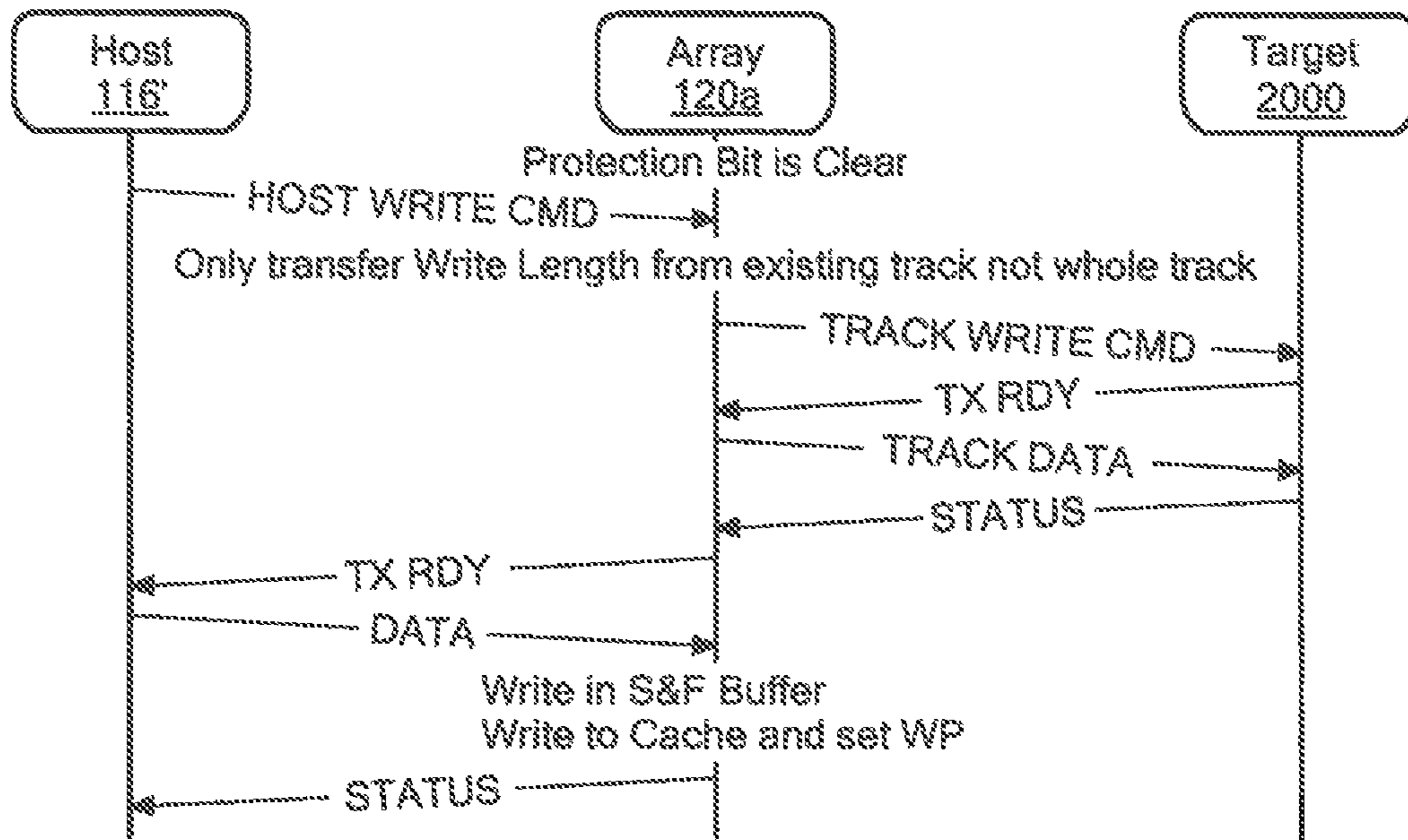
FIG. 20A
