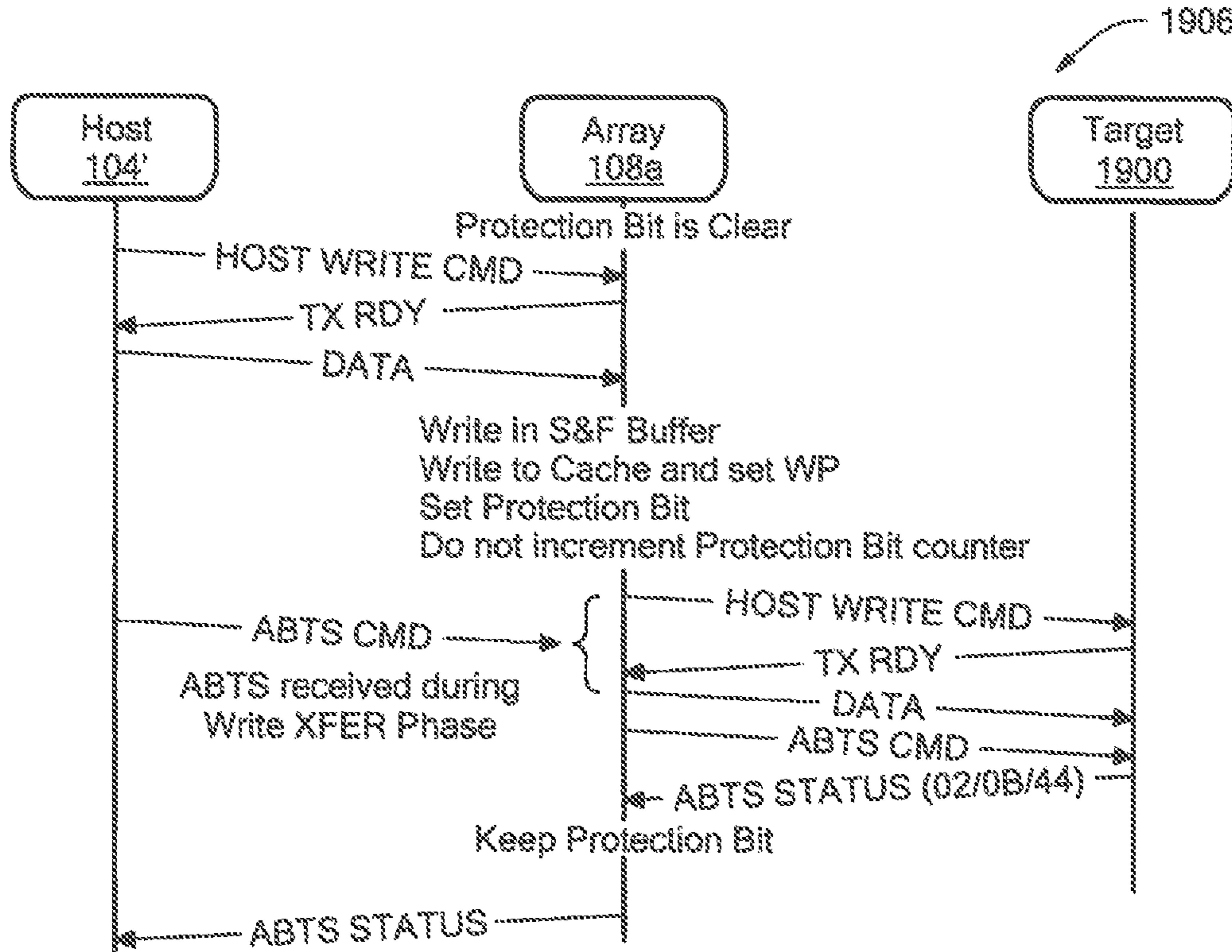
FIG. 19C
