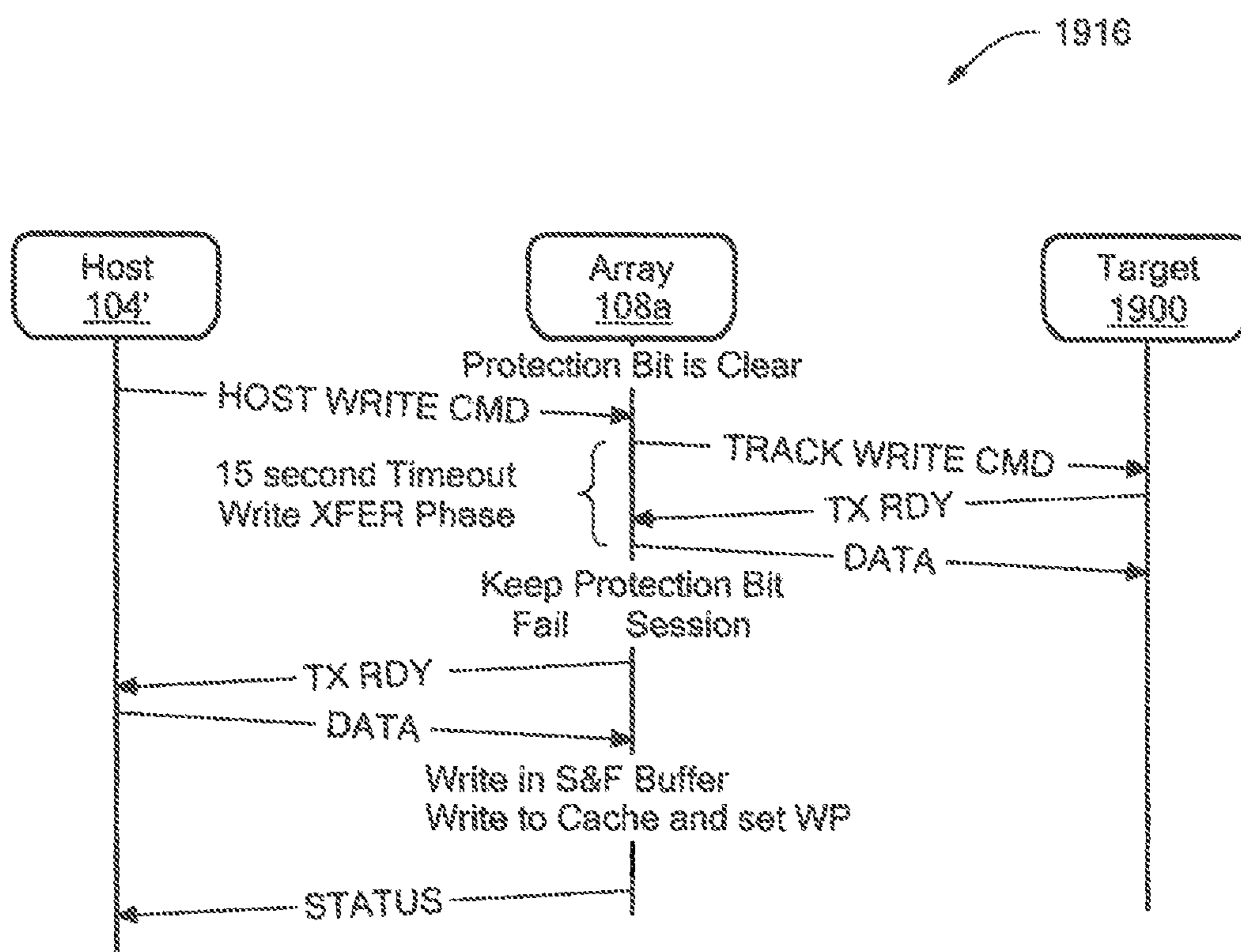
FIG. 19H
