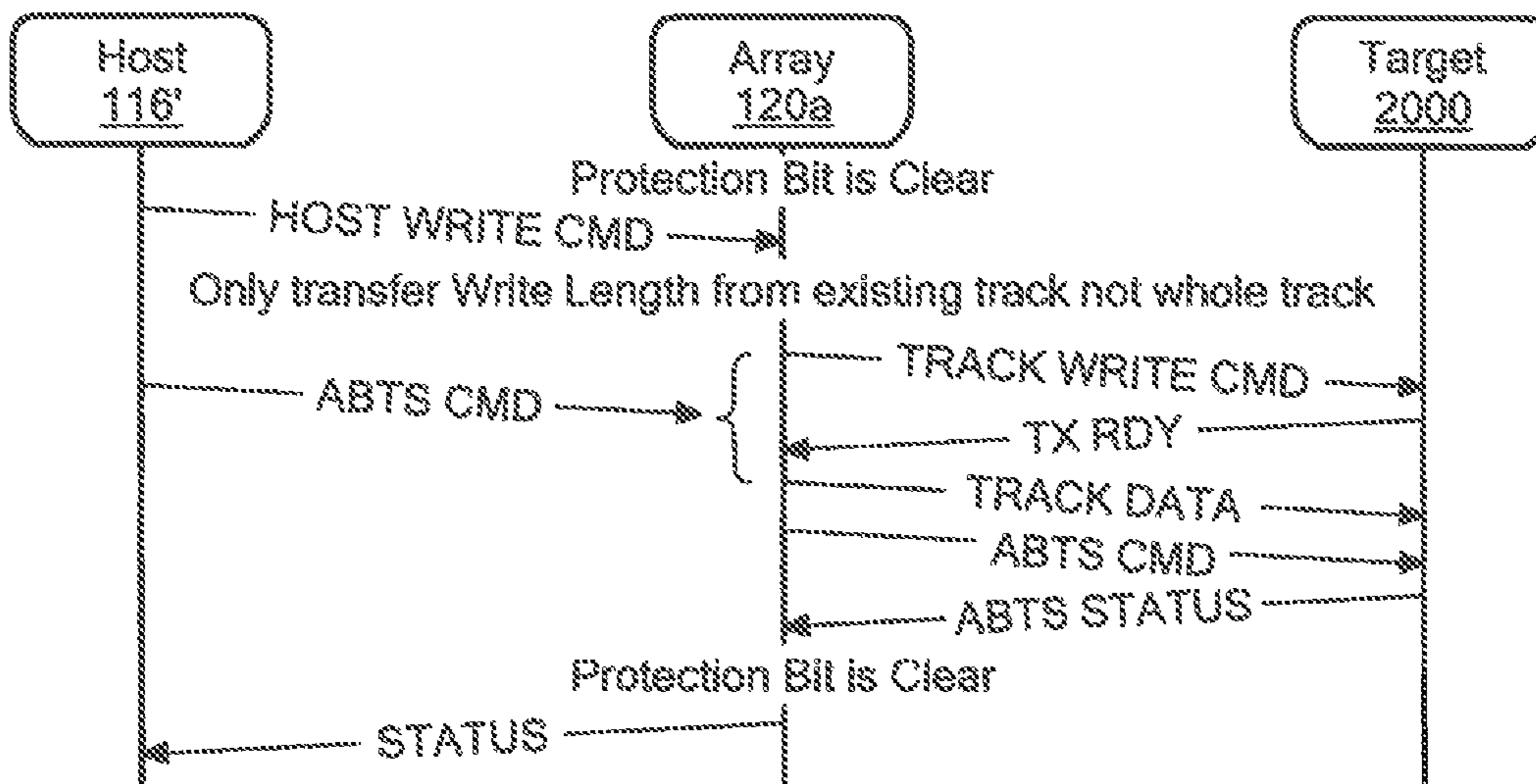
FIG. 20B
