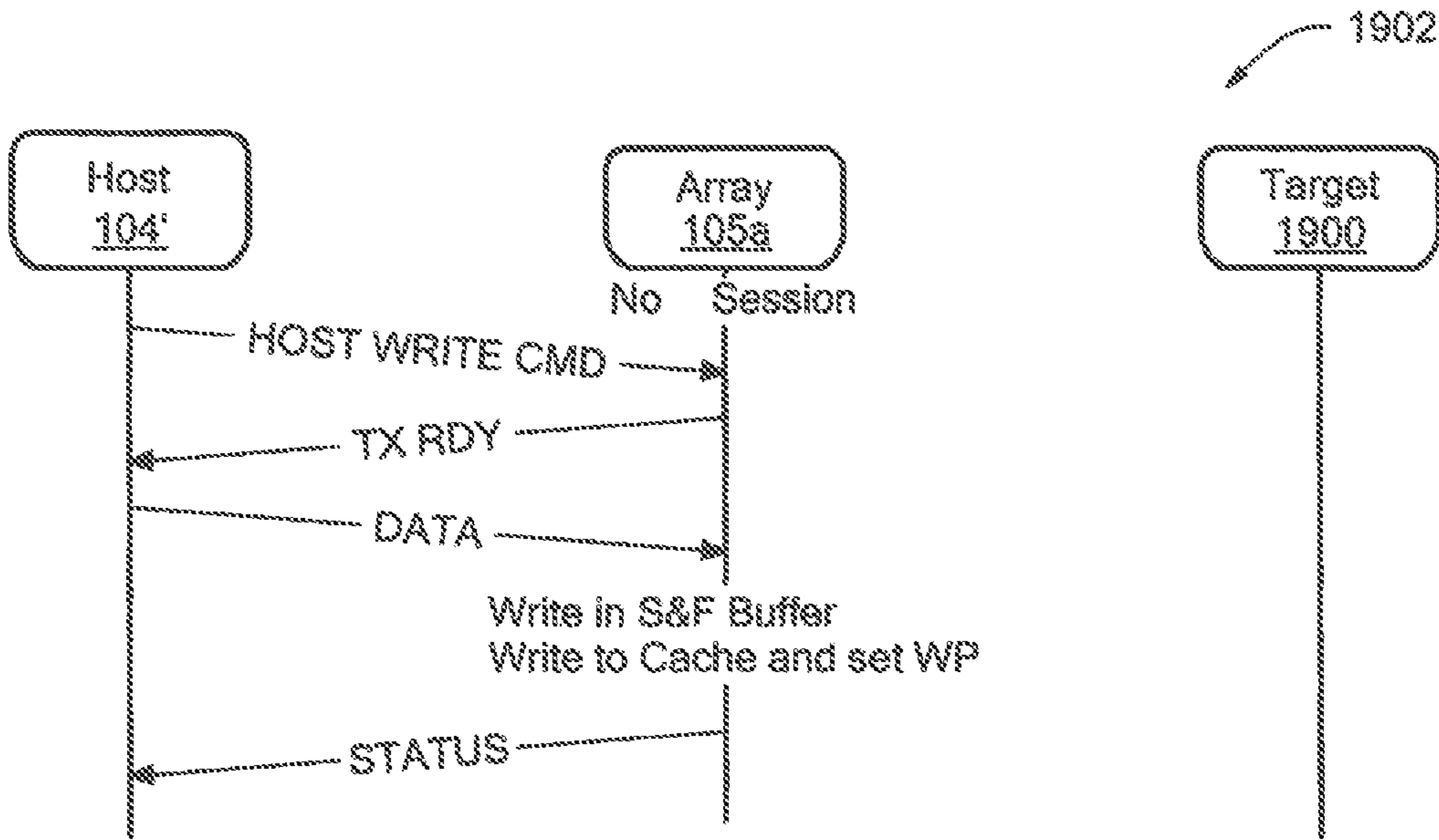
FIG. 19A
