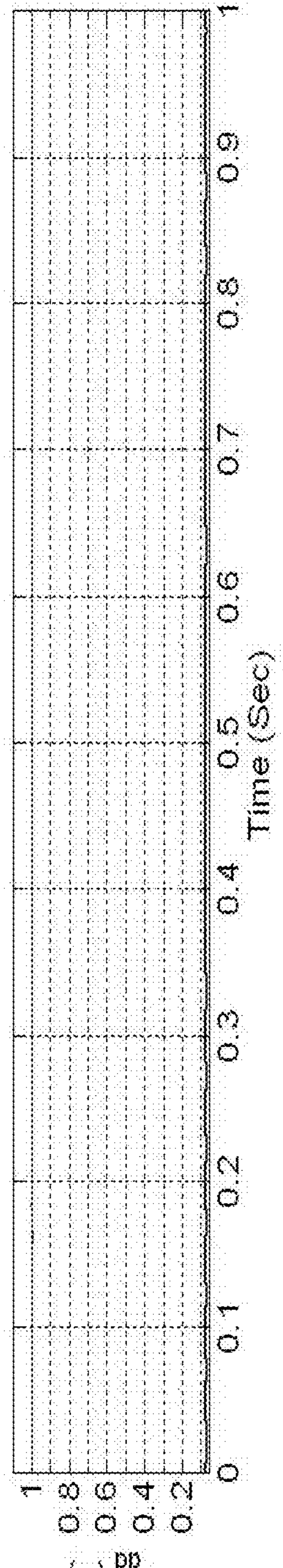
FIG. 6C S_{pp} (S)
