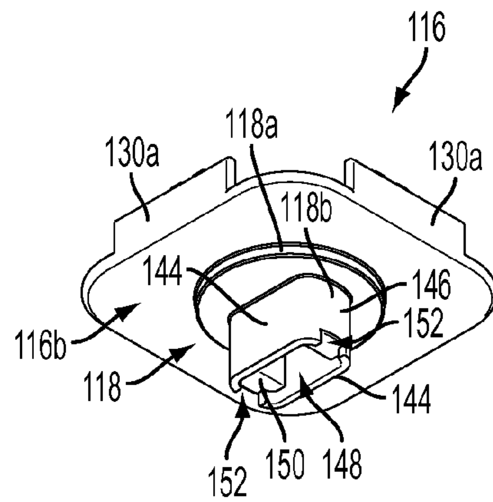
FIG. 20
