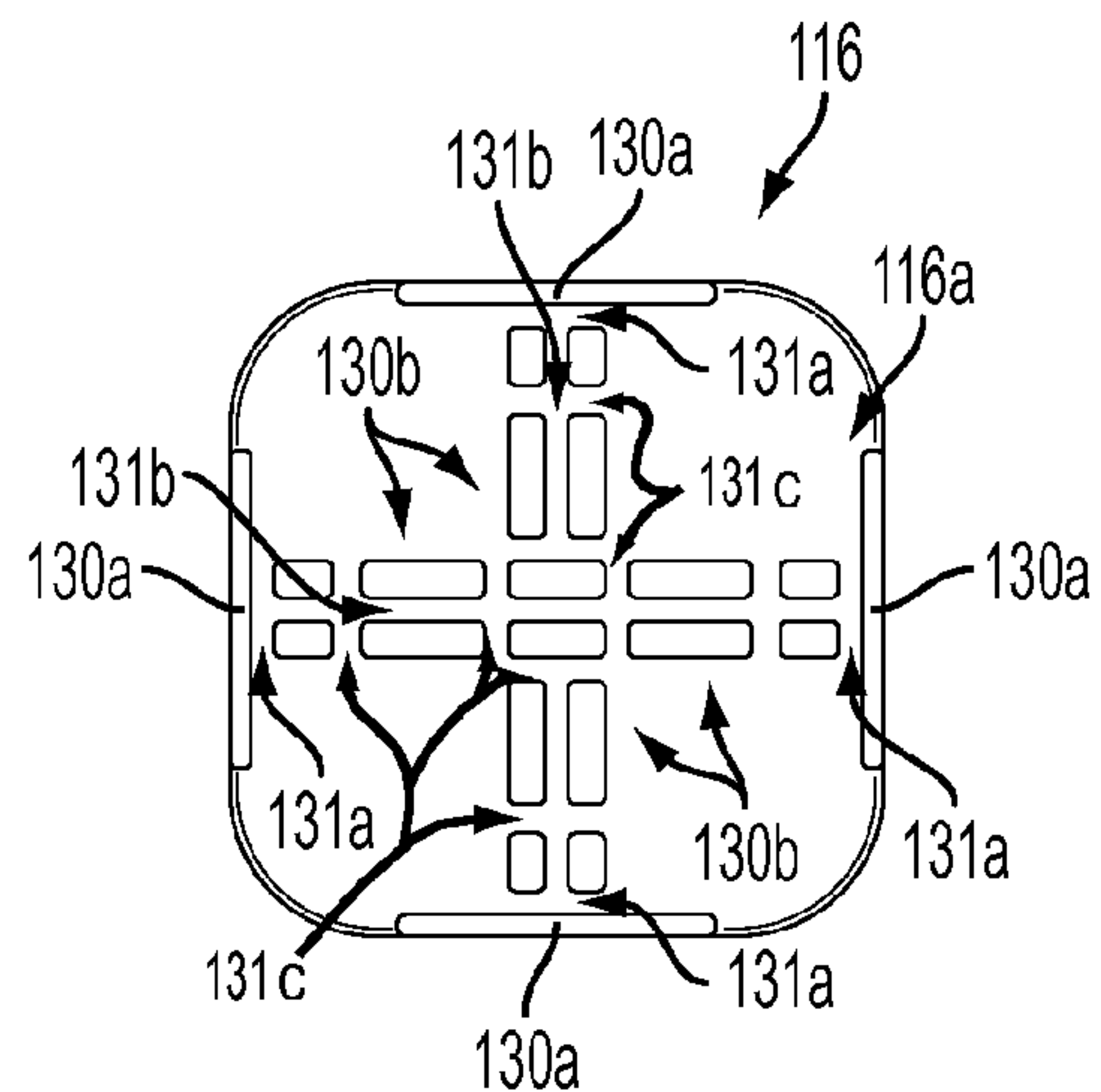
FIG. 21B
