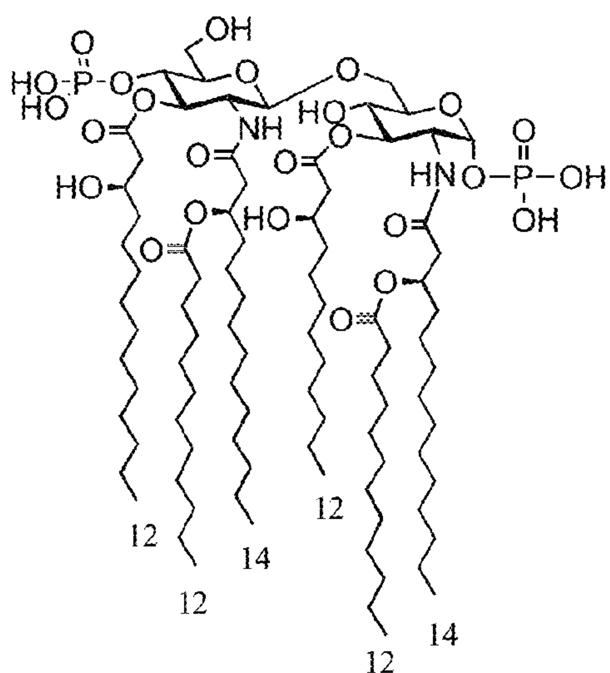
51. N. meningitidis lipid A
