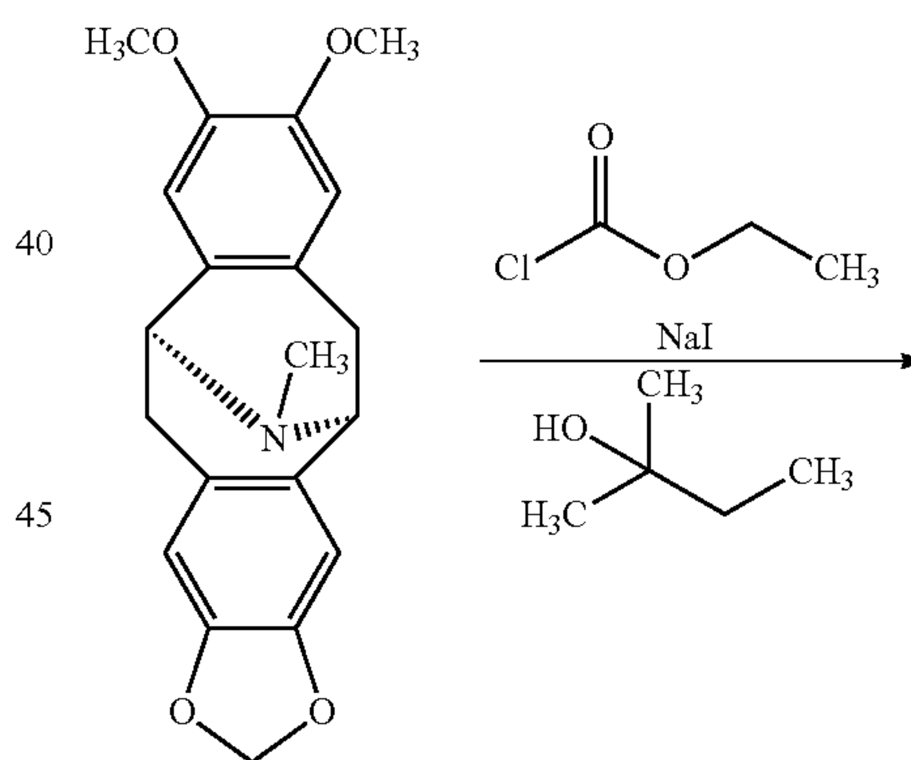
Scheme 17: (+)-Eschscholtzidine
