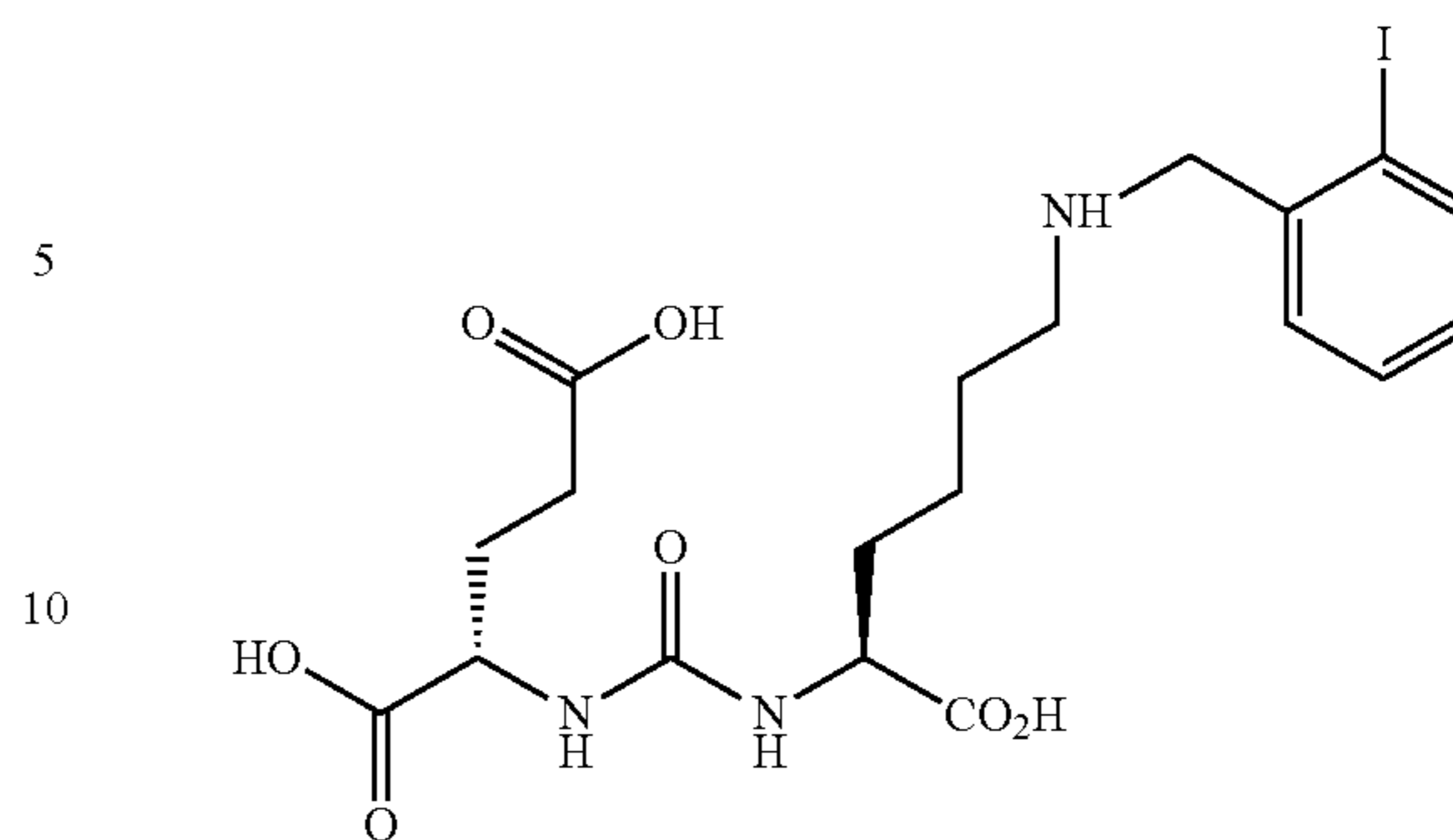
(S,S)-2-{3-[1-Carboxy-5-(3-iodo-benzylamino)-pentyl]-ureido}-pentanedioic (13) (MIP 1089)
