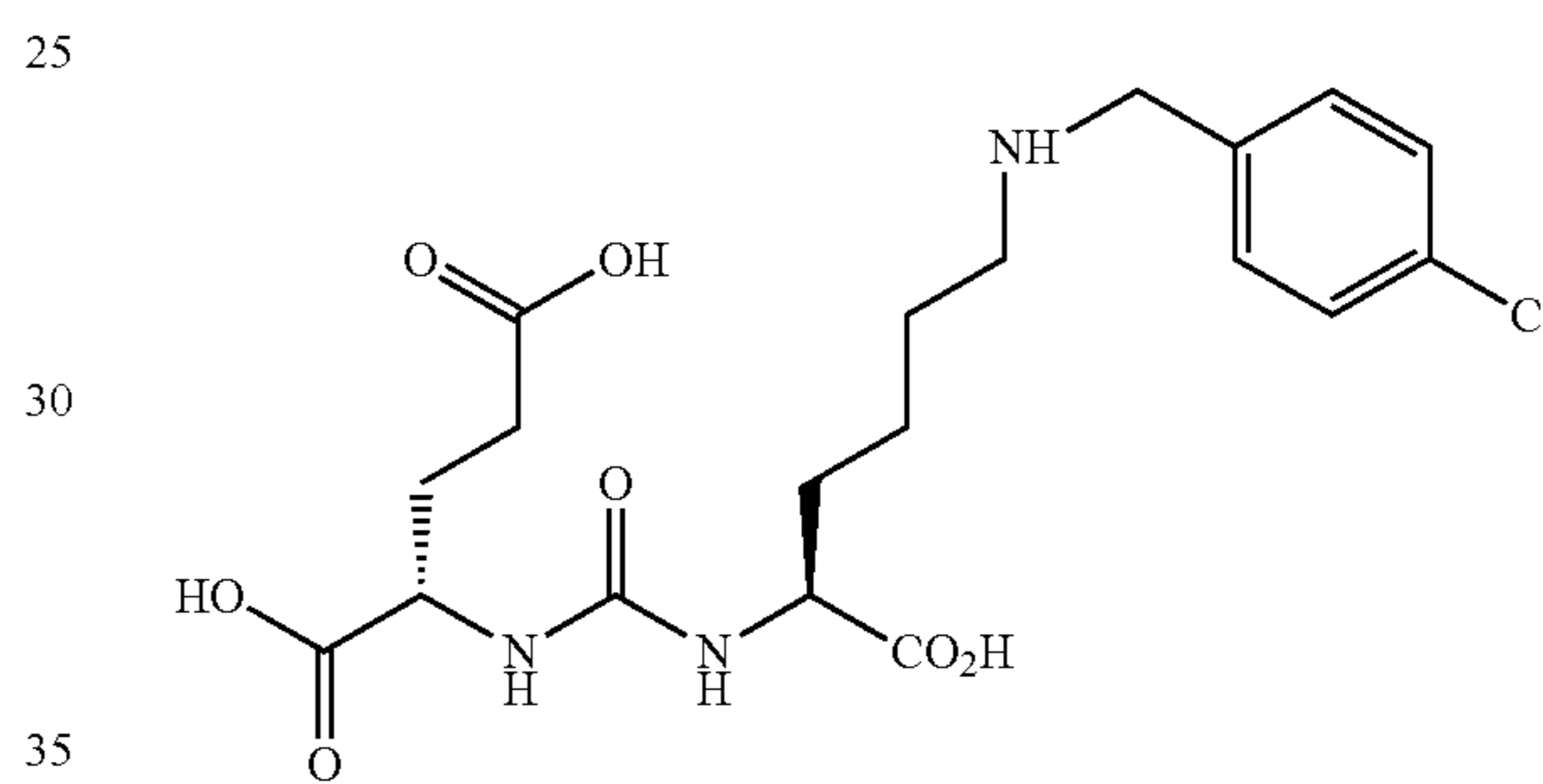
(S)-2-(3-((R)-5-(benzylamino)-1-carboxypentyl)ureido)pentanedioic acid (10) (MIP-1106)
