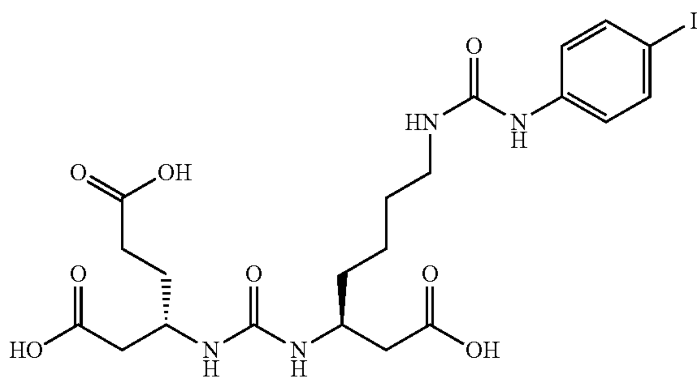
\beta -lys, \beta -glu
