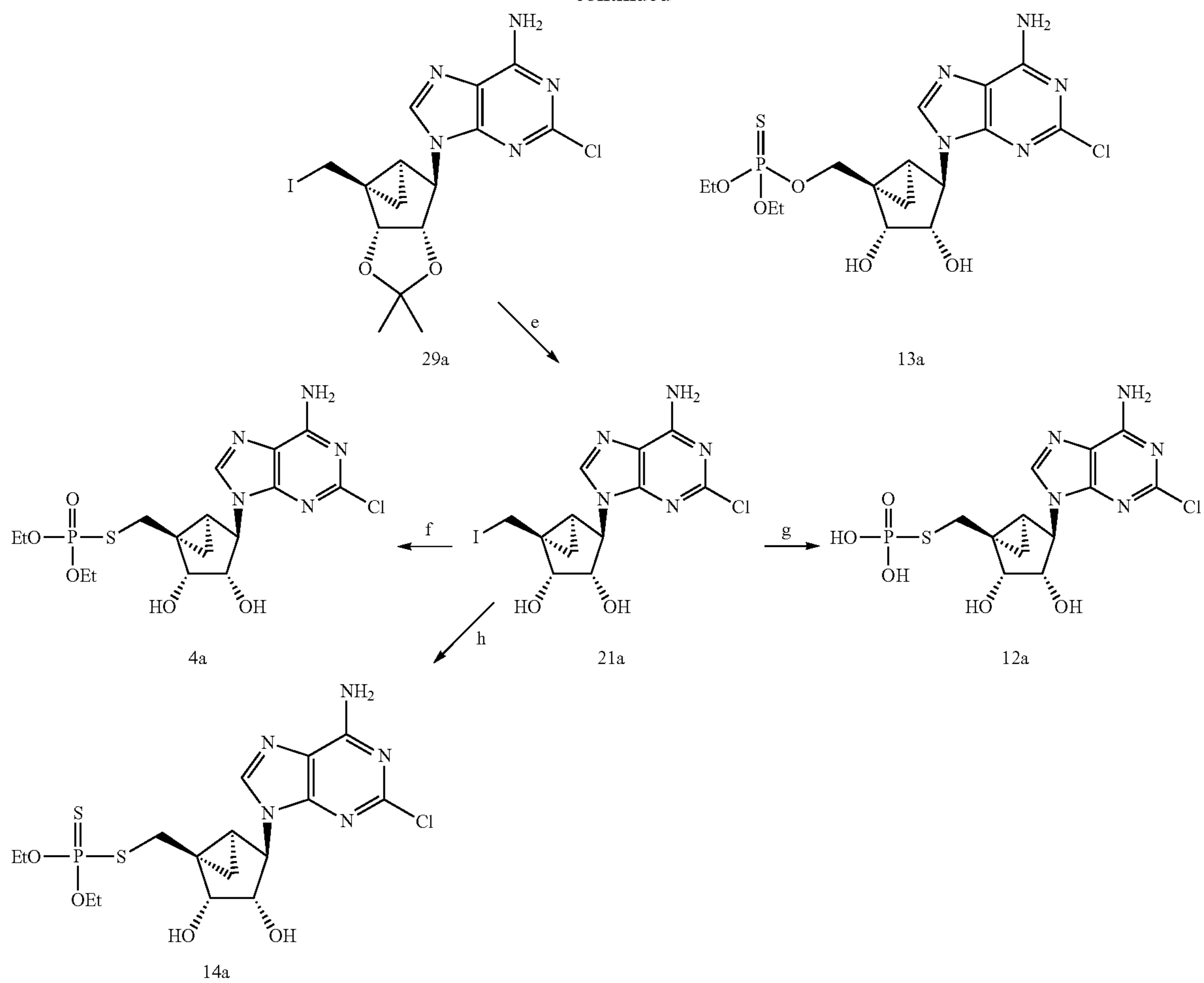
Scheme 2a
