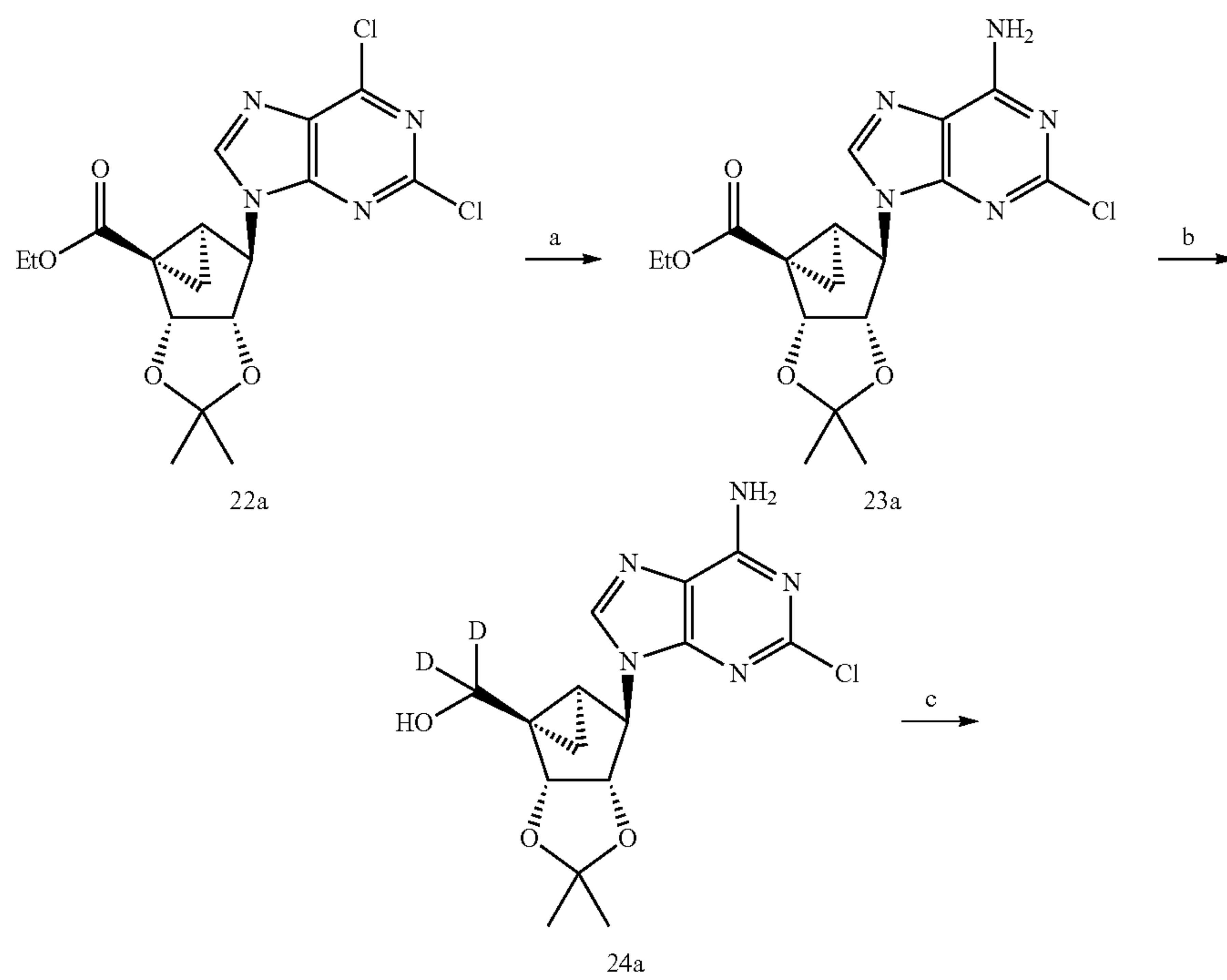
Scheme 2a
