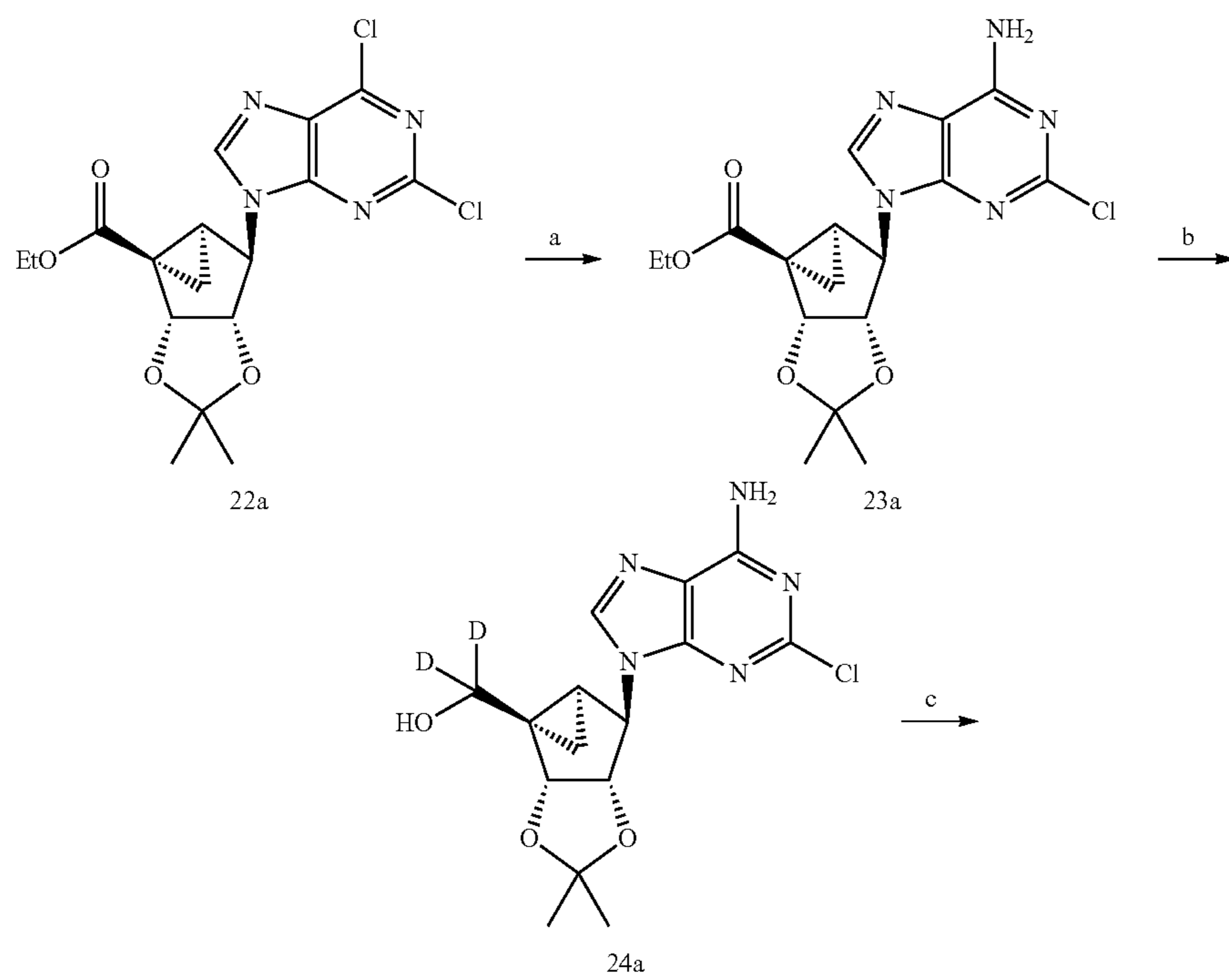
Scheme 2a
