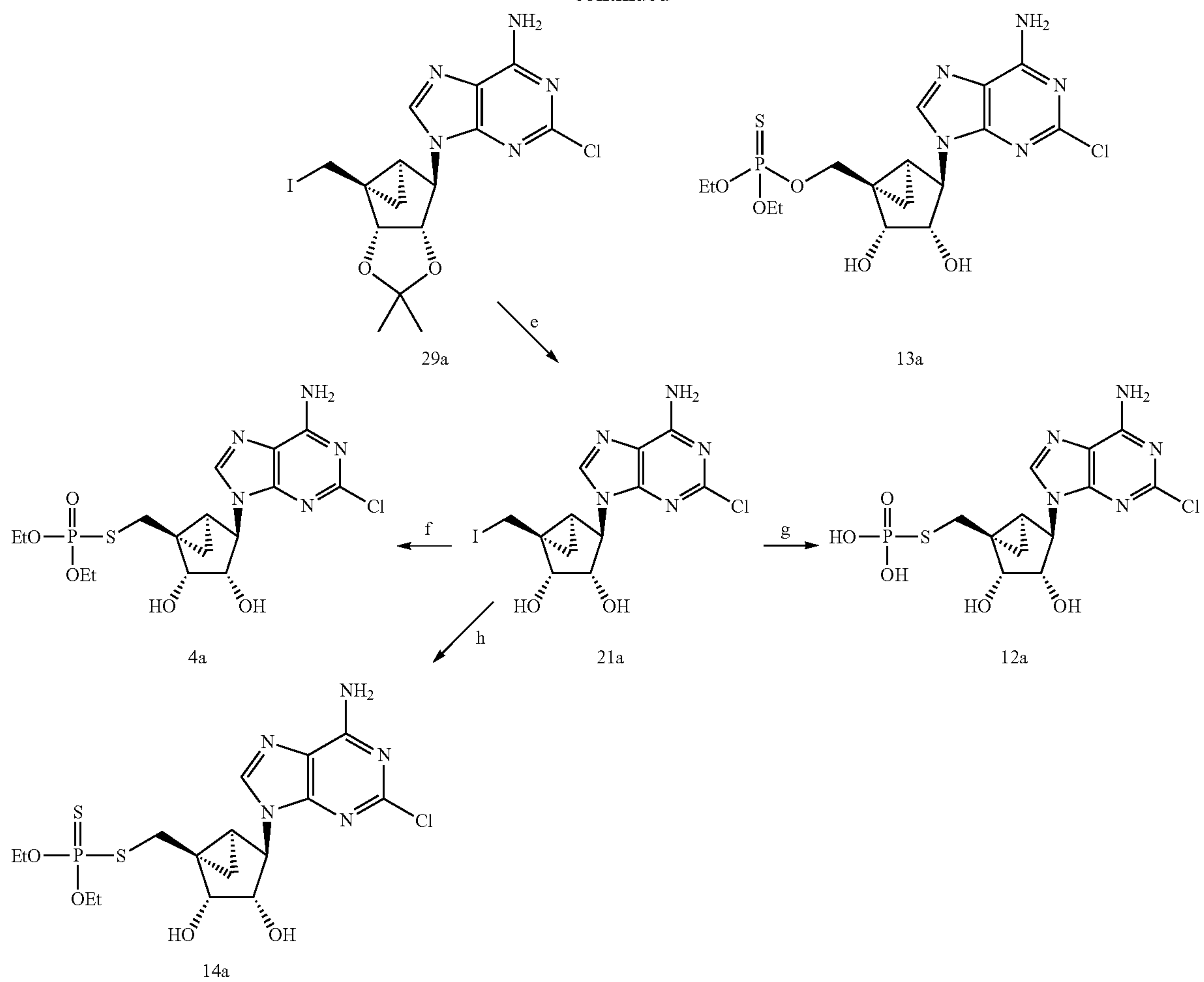
Scheme 2a
