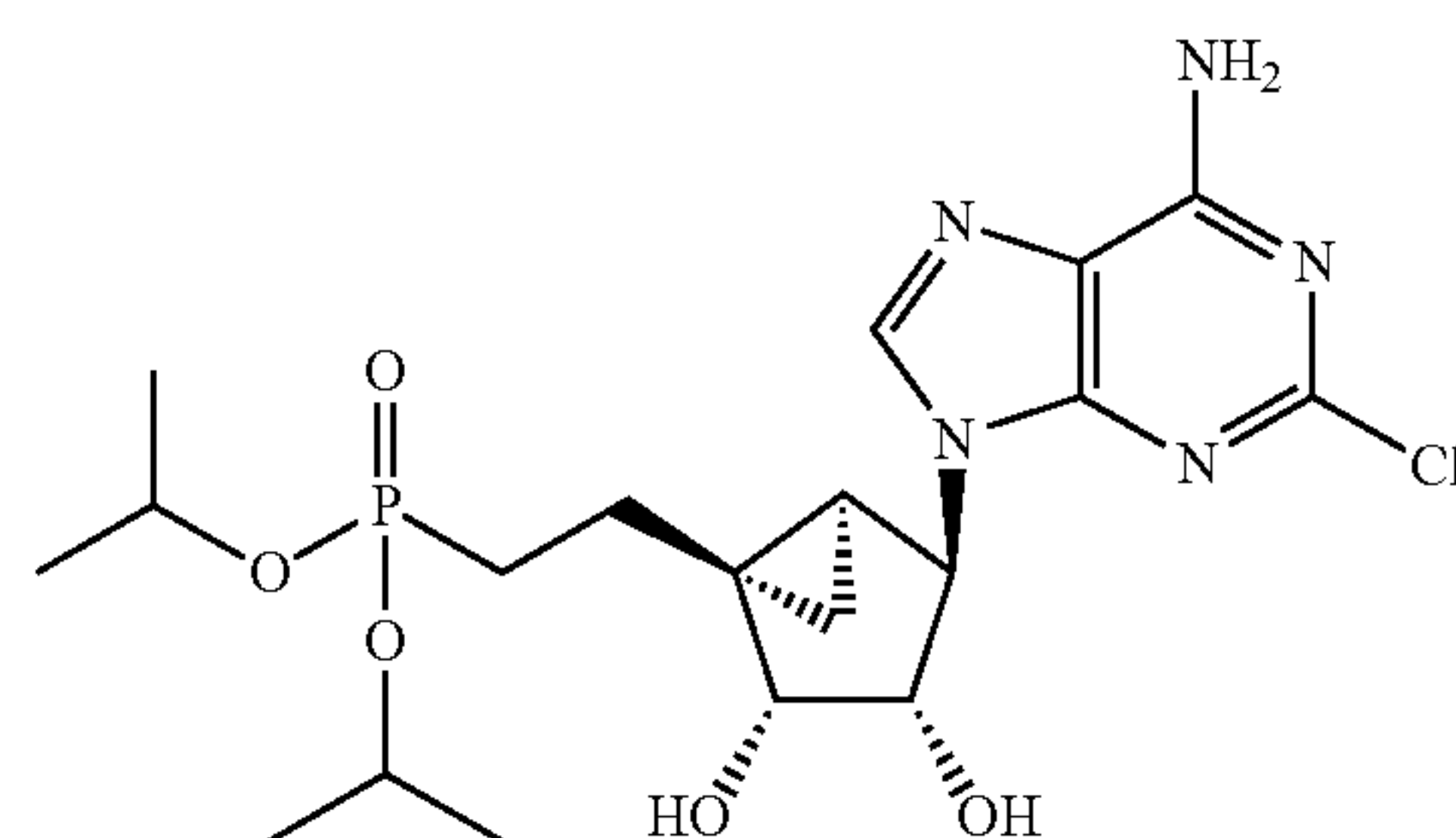
MRS2978
