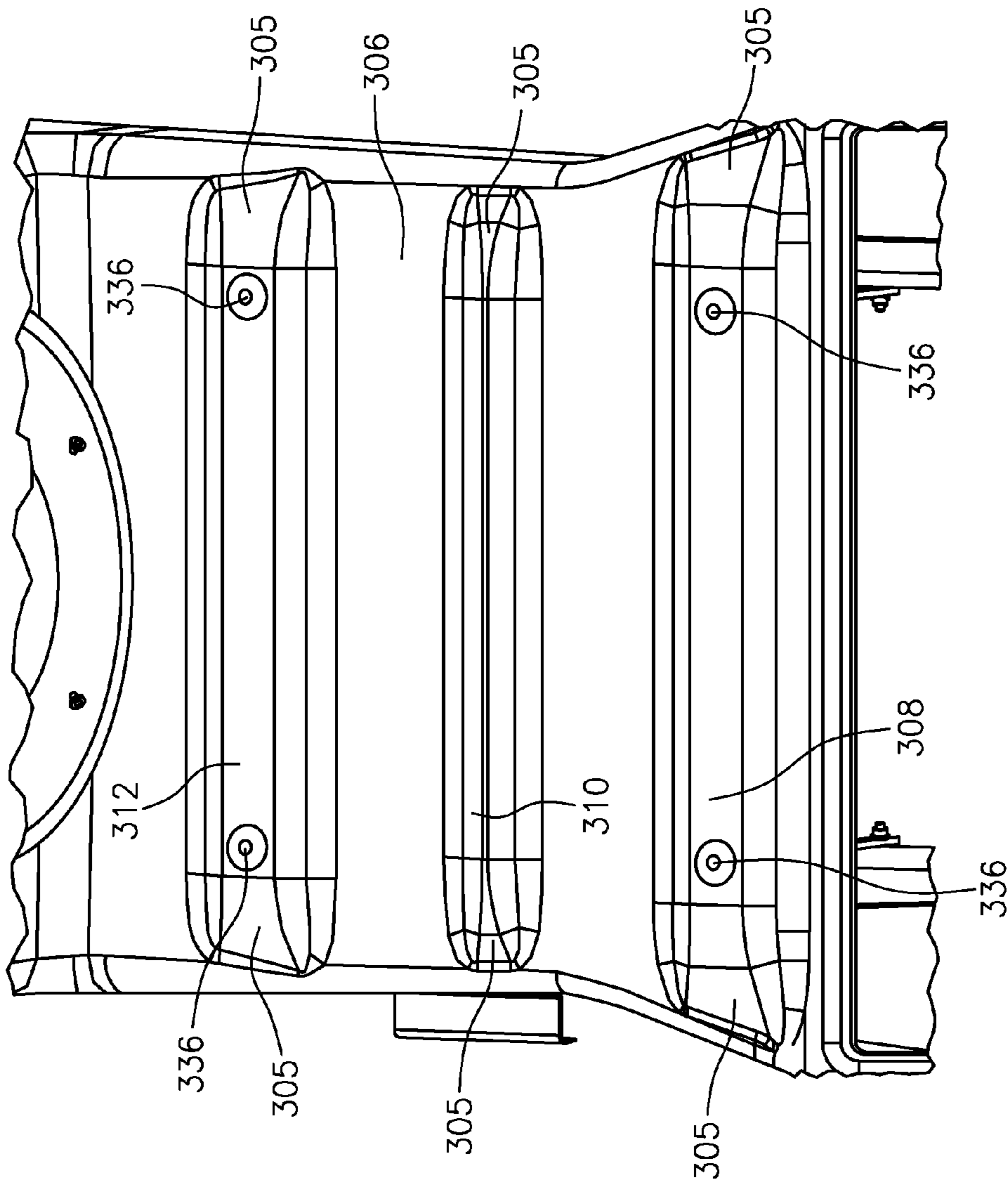
FIG. 5
