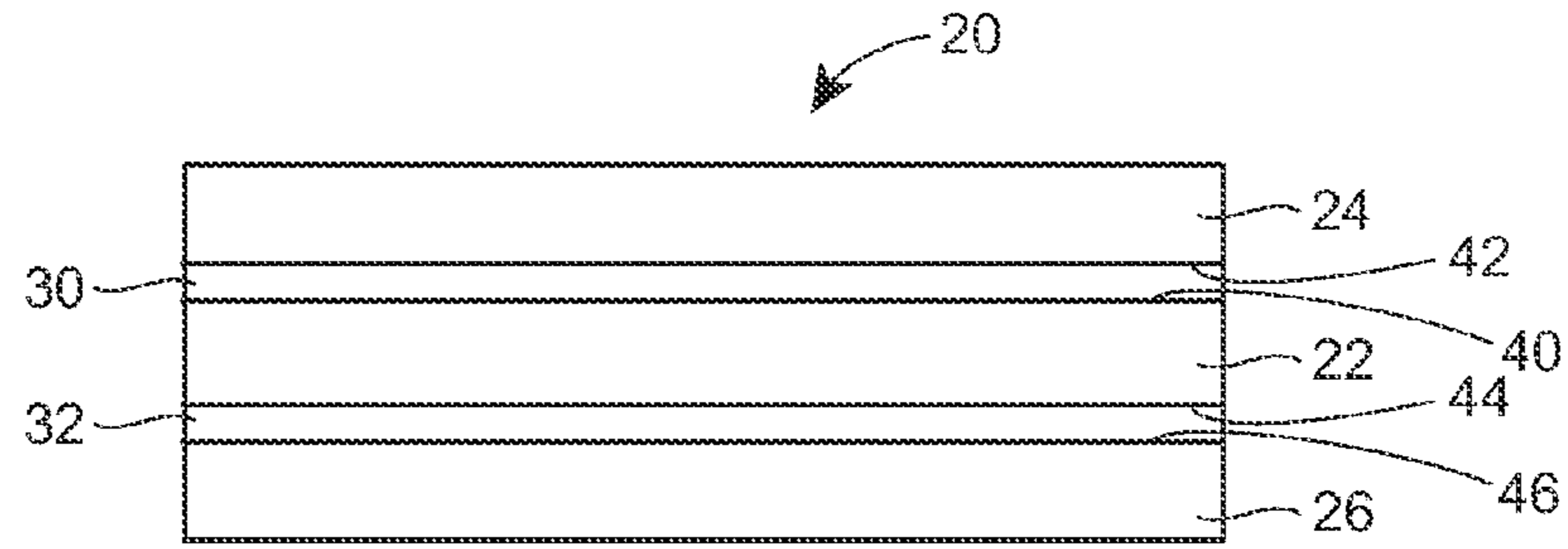
FIG. 1A
