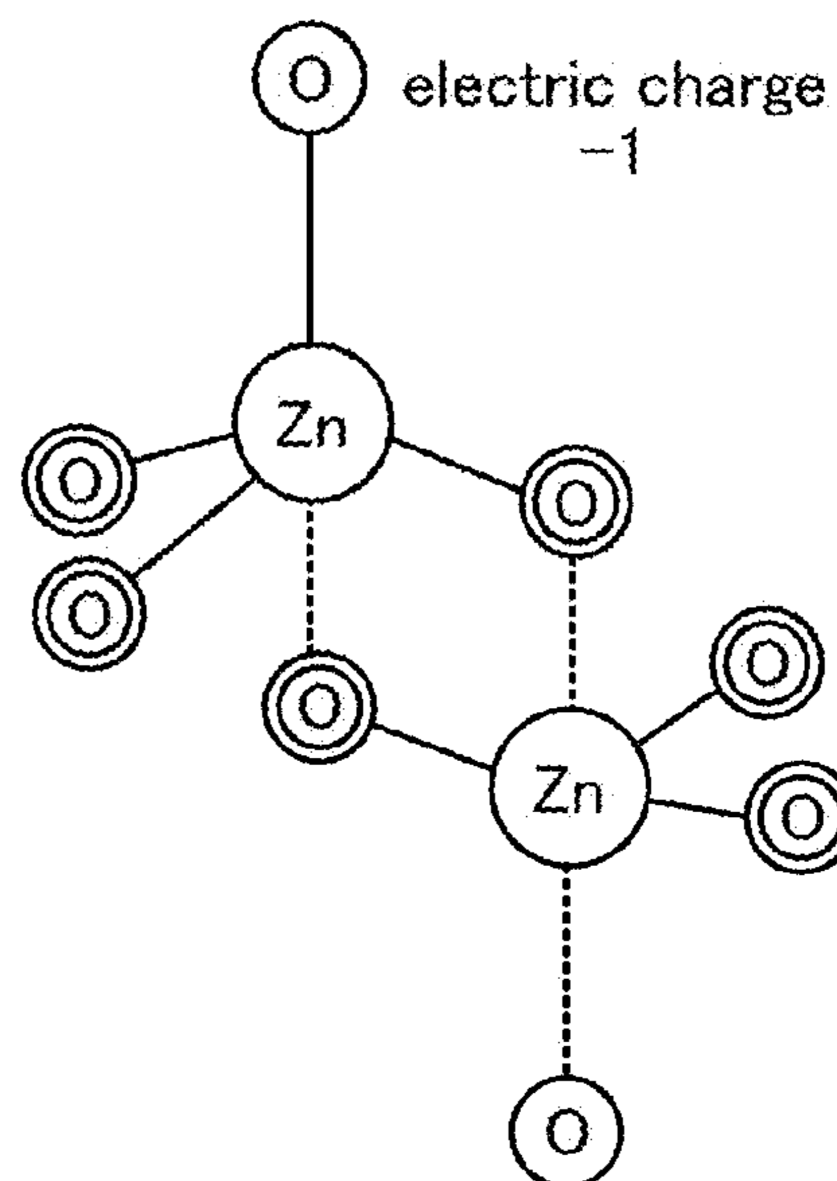
FIG. 12E
