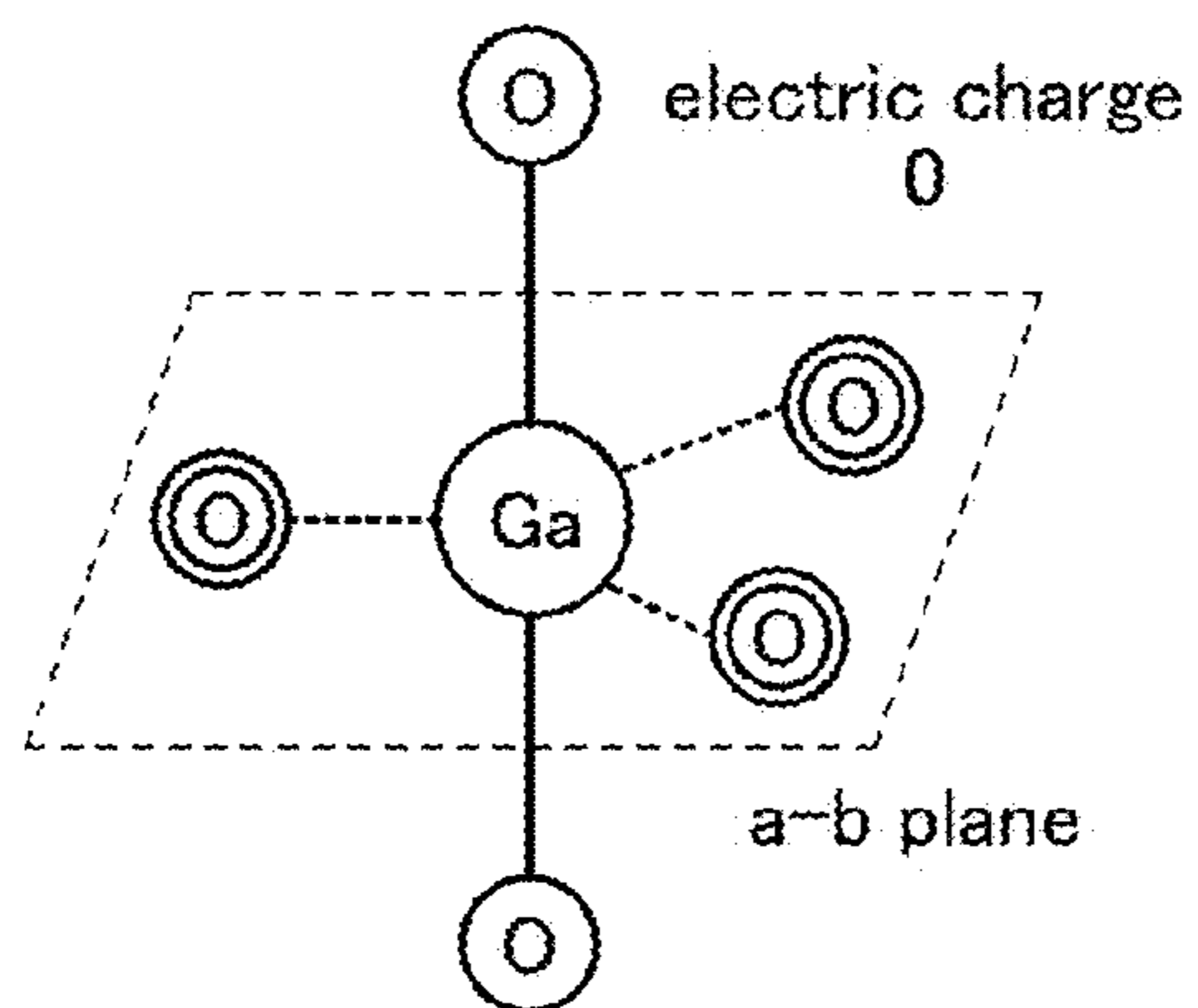
FIG. 12C
