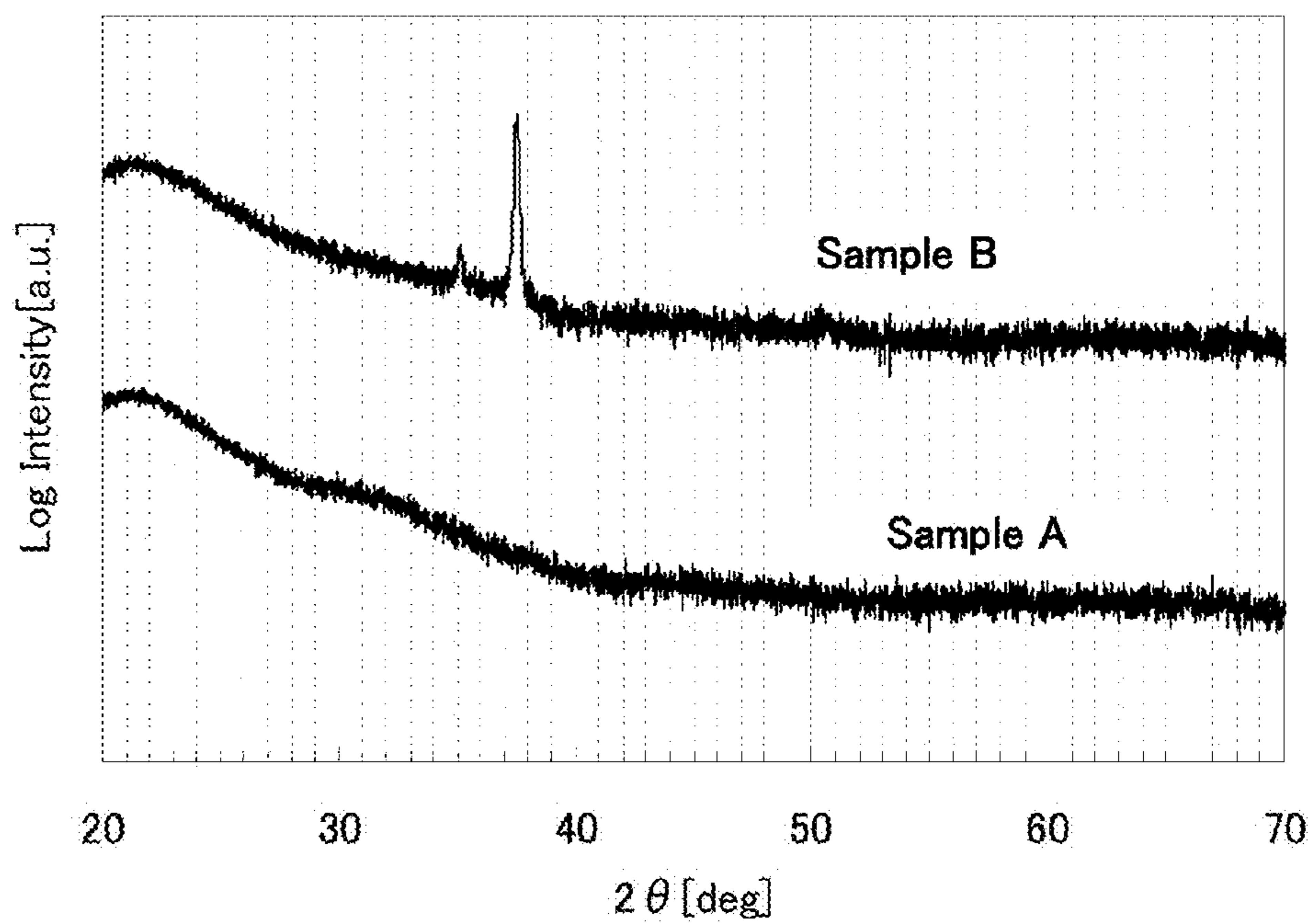
FIG. 25
