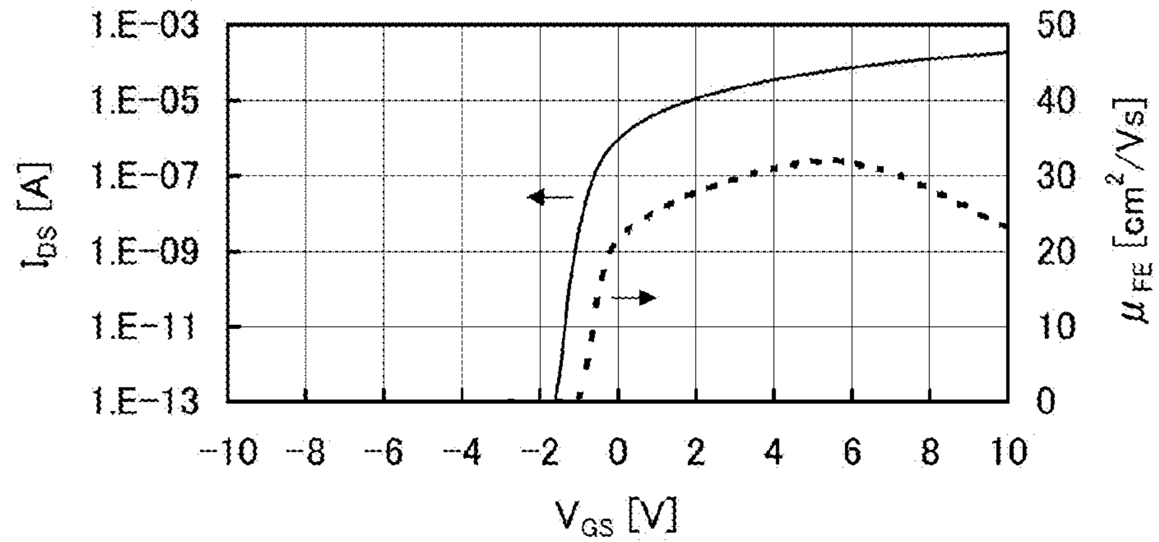
FIG. 20C
