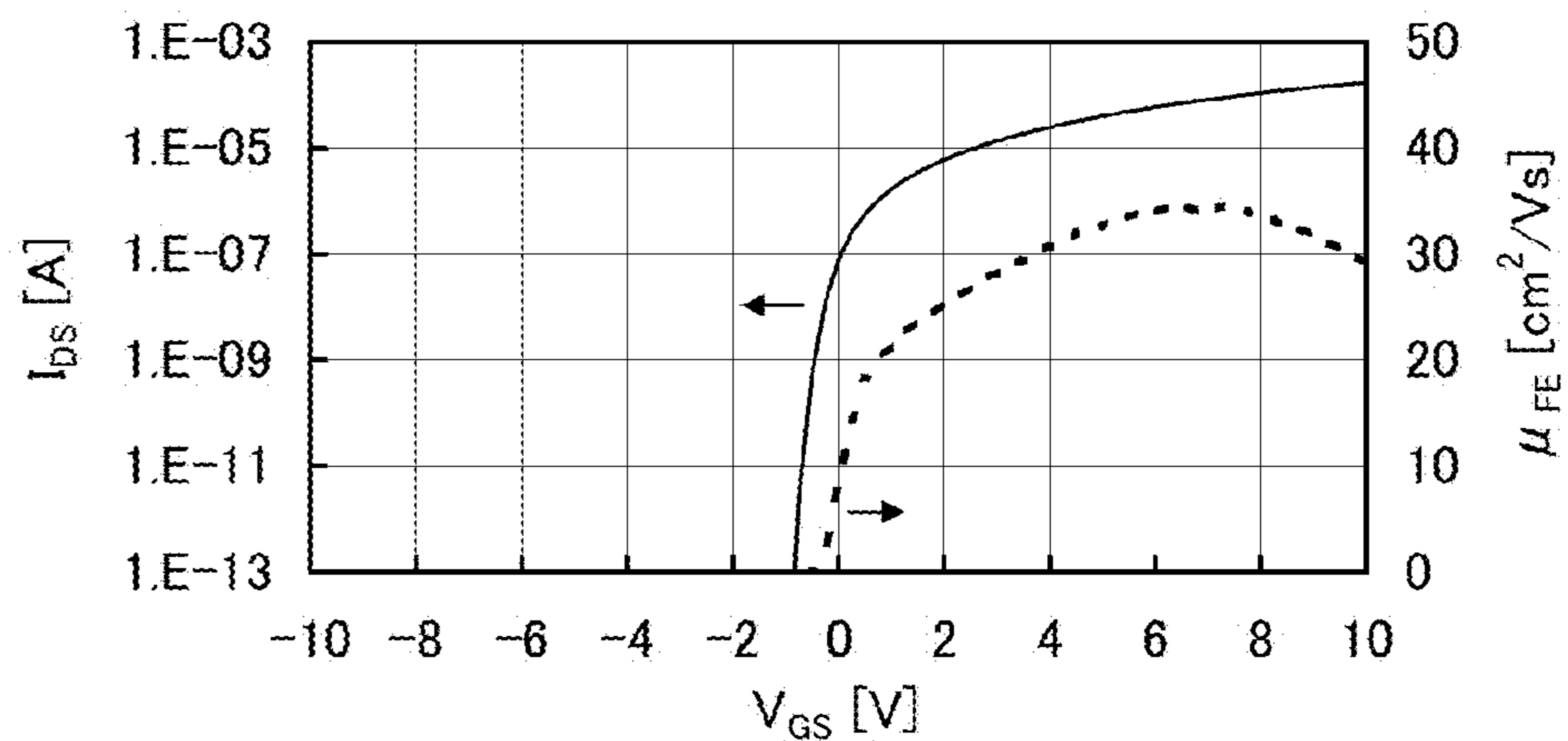
FIG. 20C
