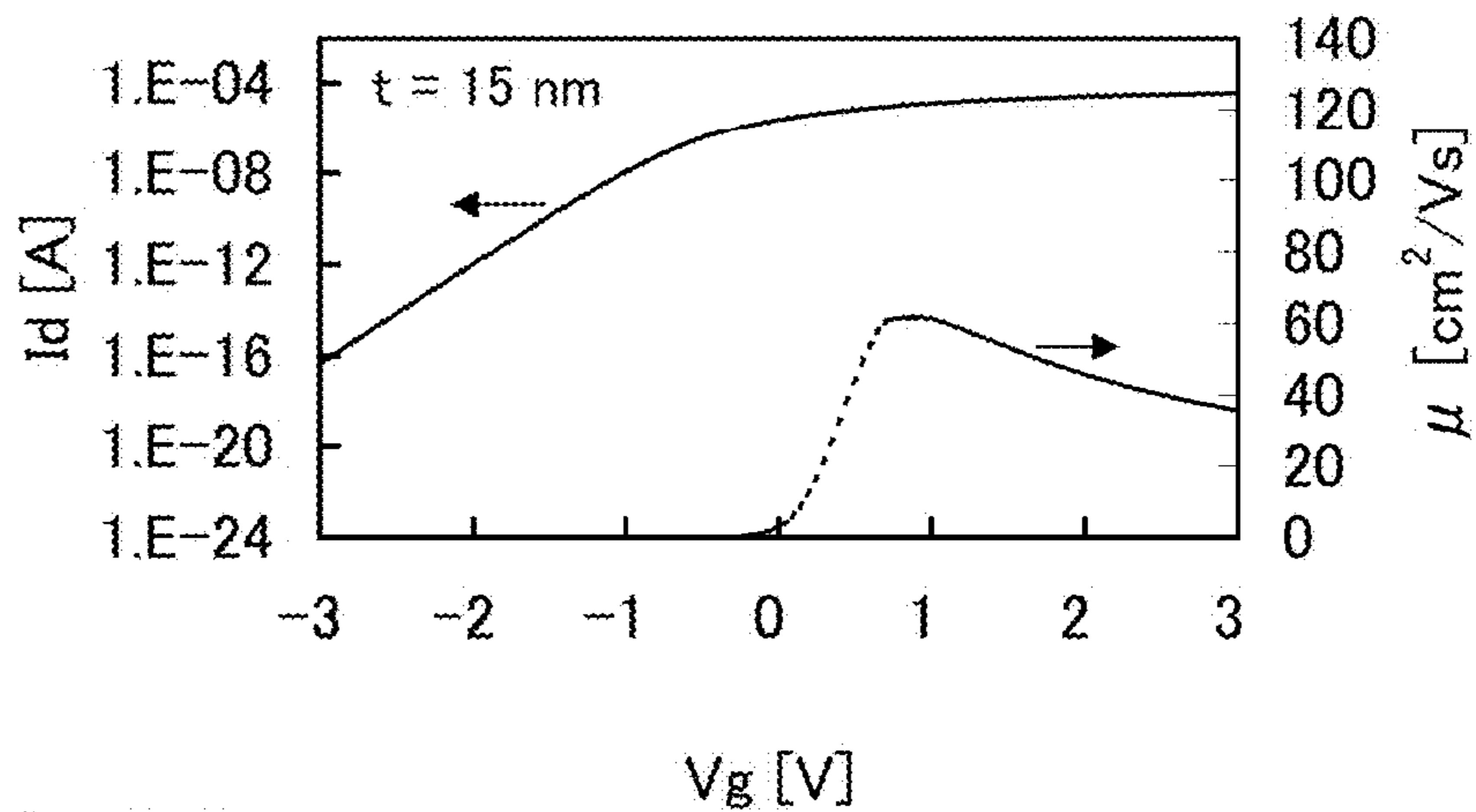
FIG. 17B
