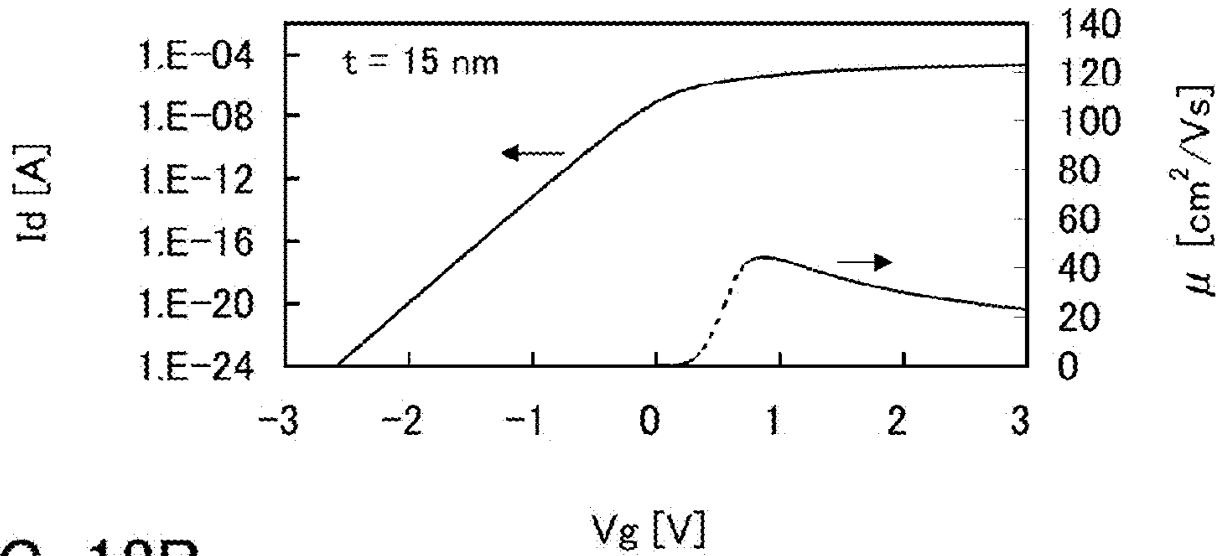
FIG. 18B
