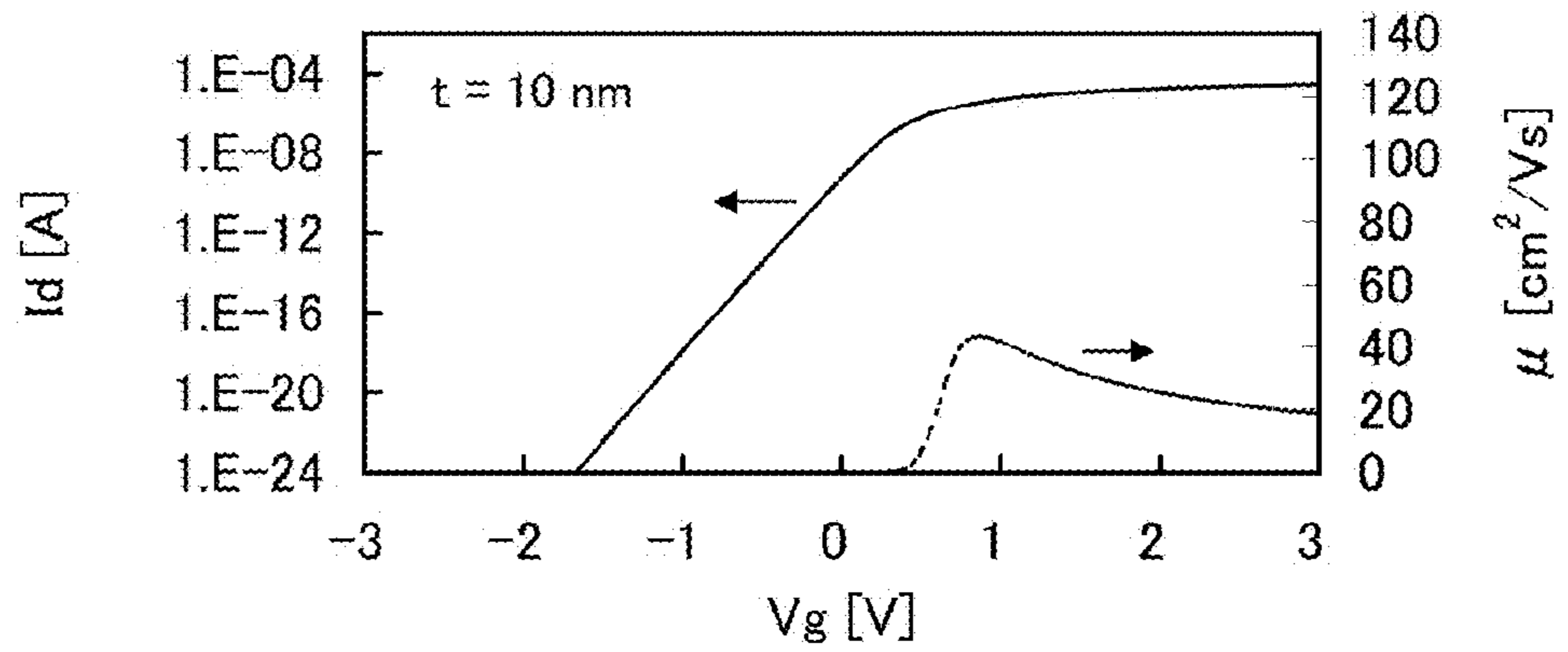
FIG. 18C
