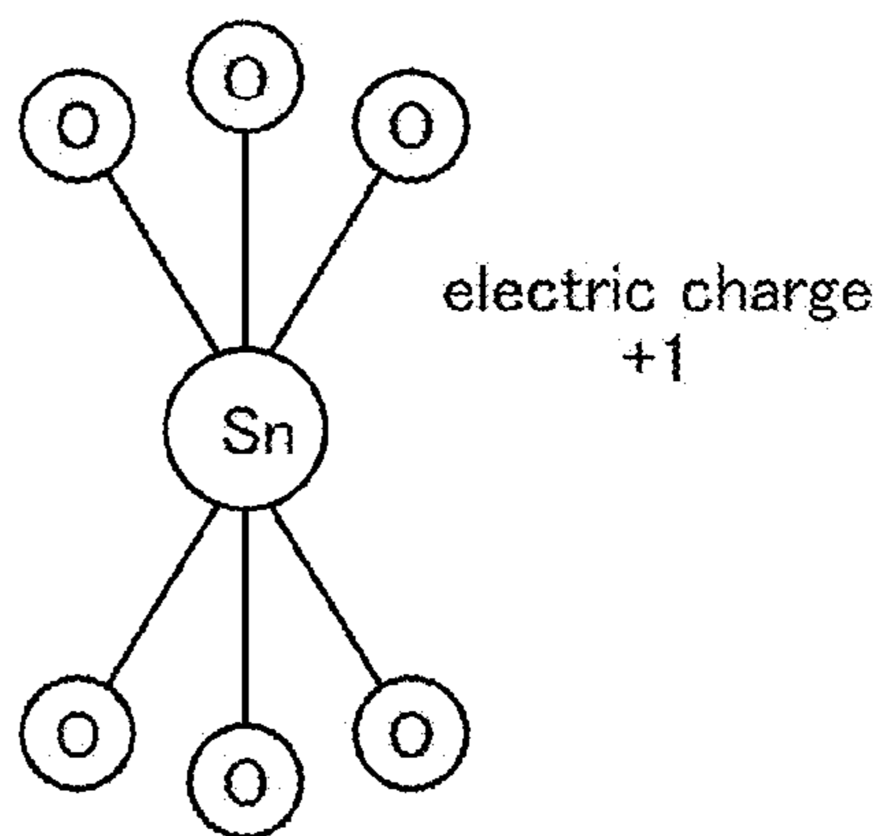
FIG. 12E
