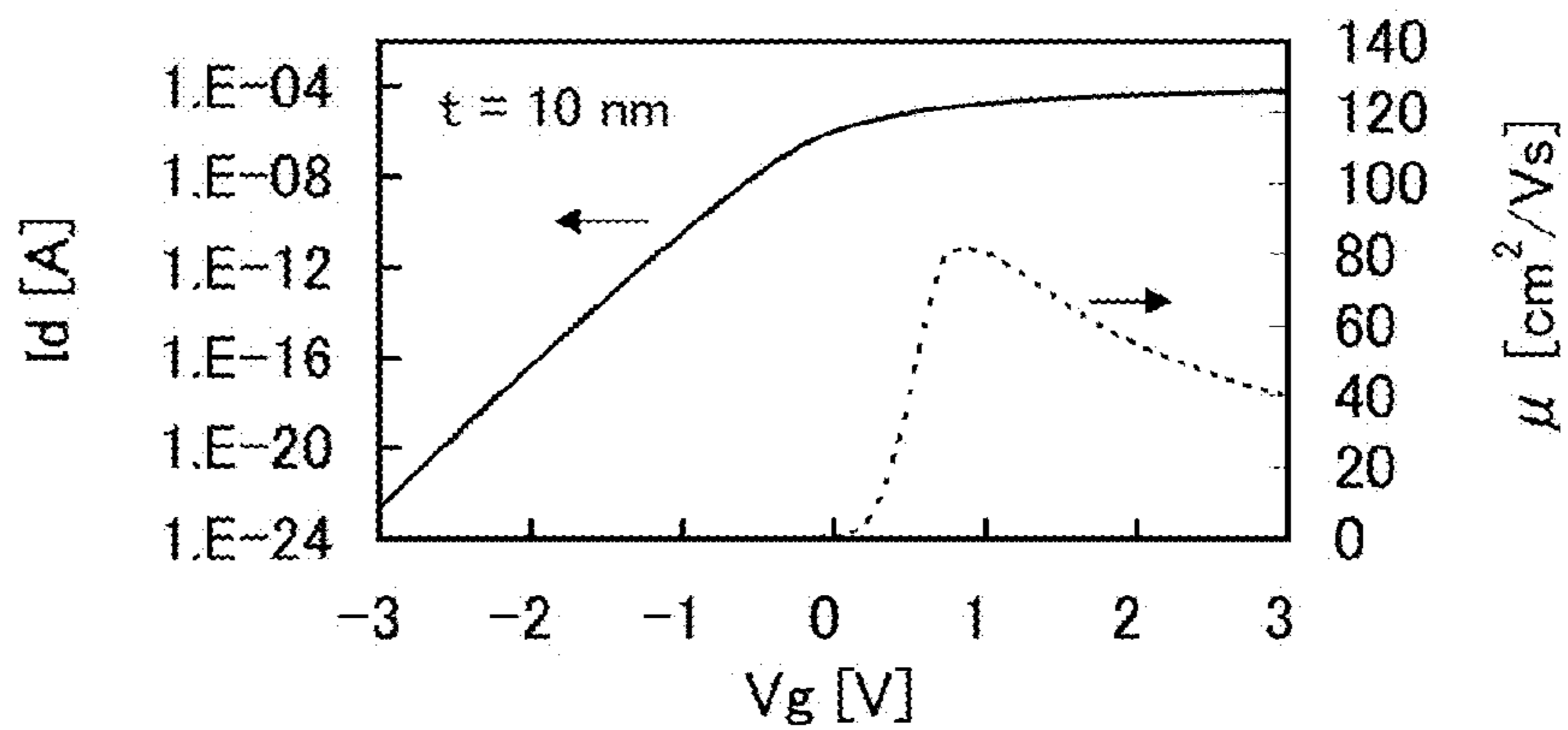
FIG. 16C
