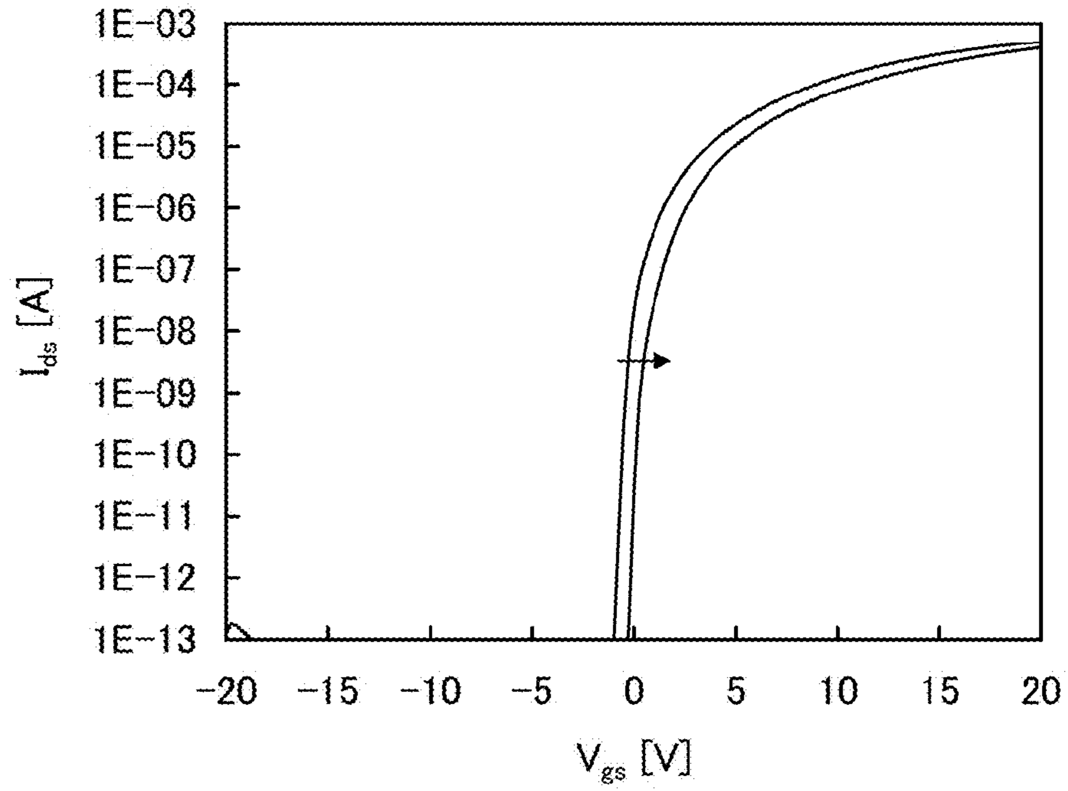
FIG. 22B
