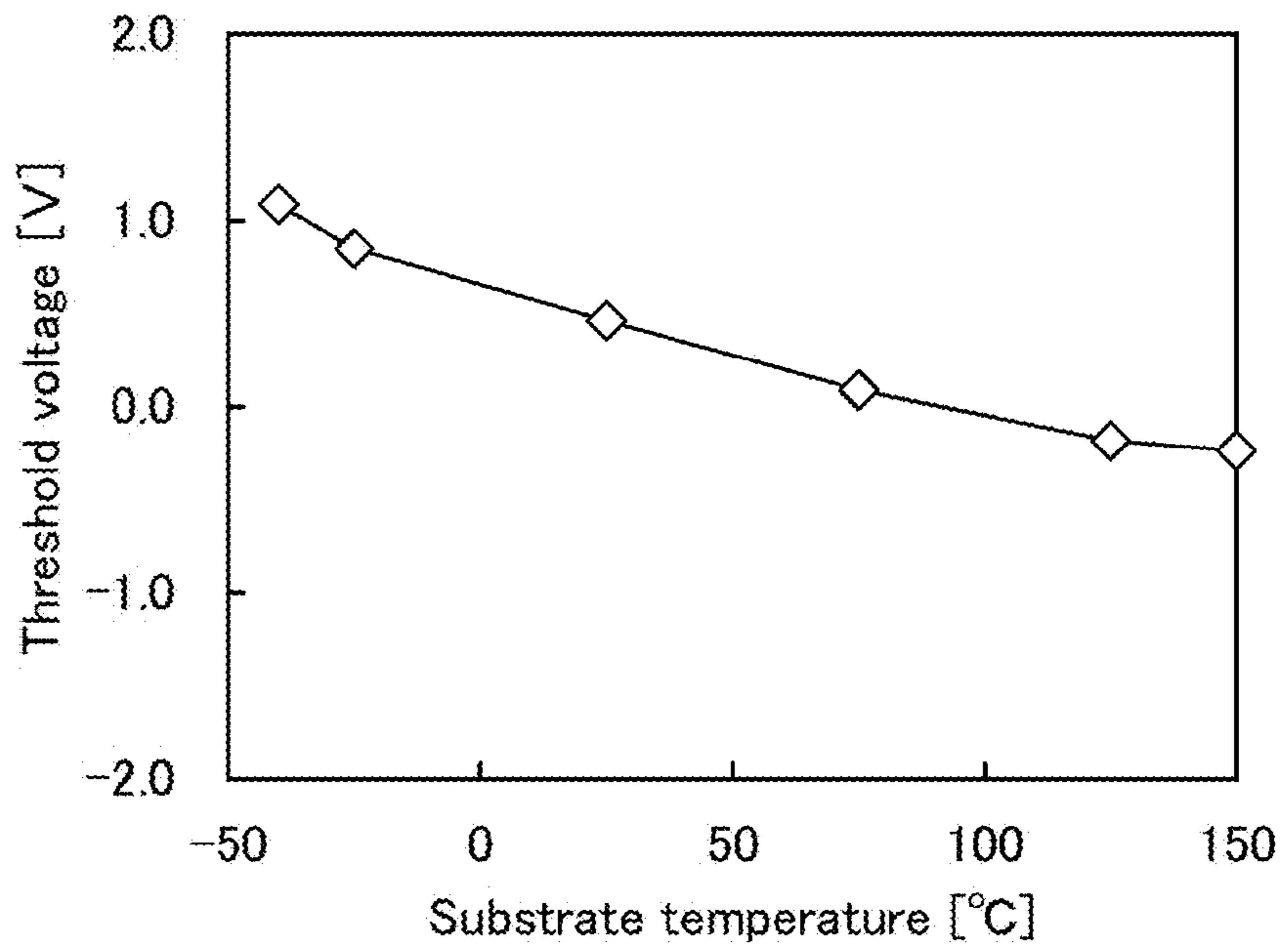
FIG. 24B
