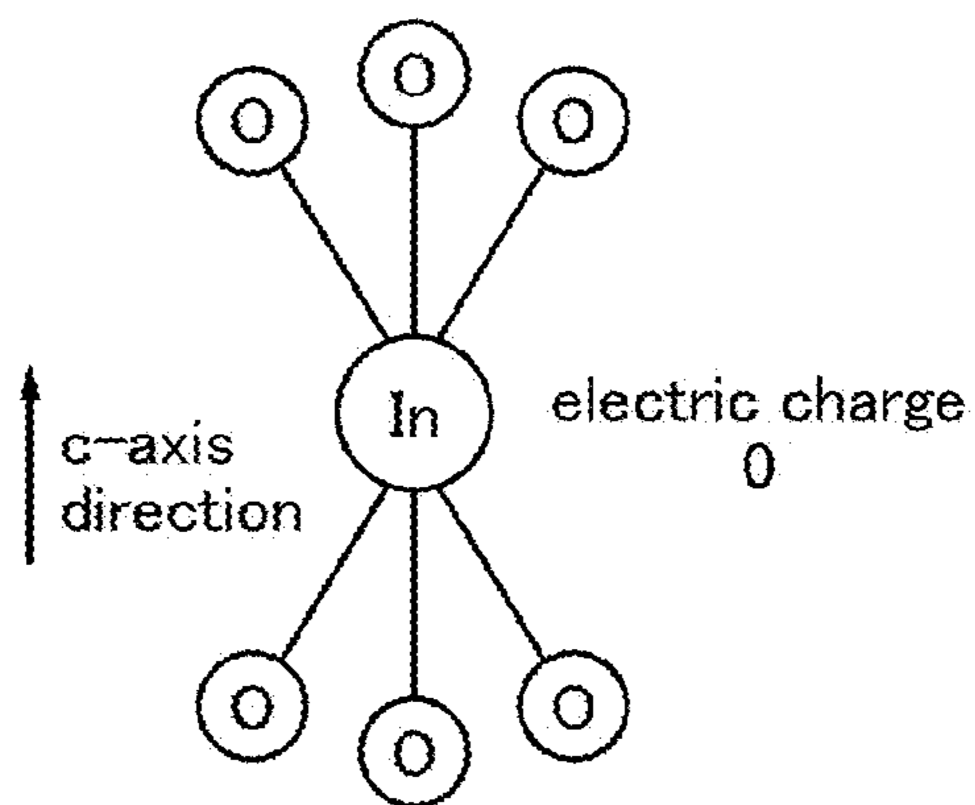
FIG. 12B
