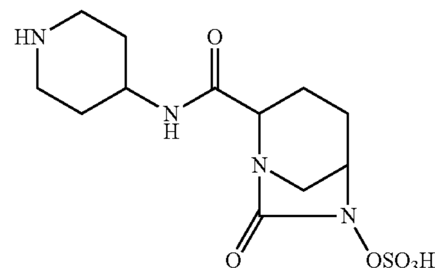
MK-7655
