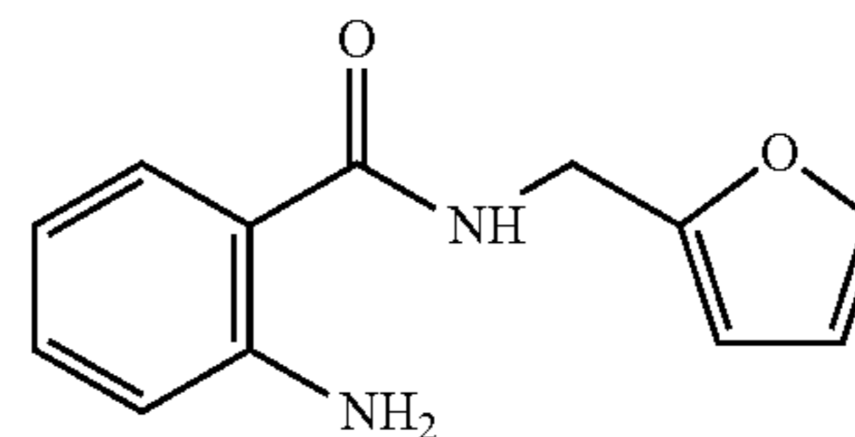
2-Amino-N-(furan-2-ylmethyl)benzamide
