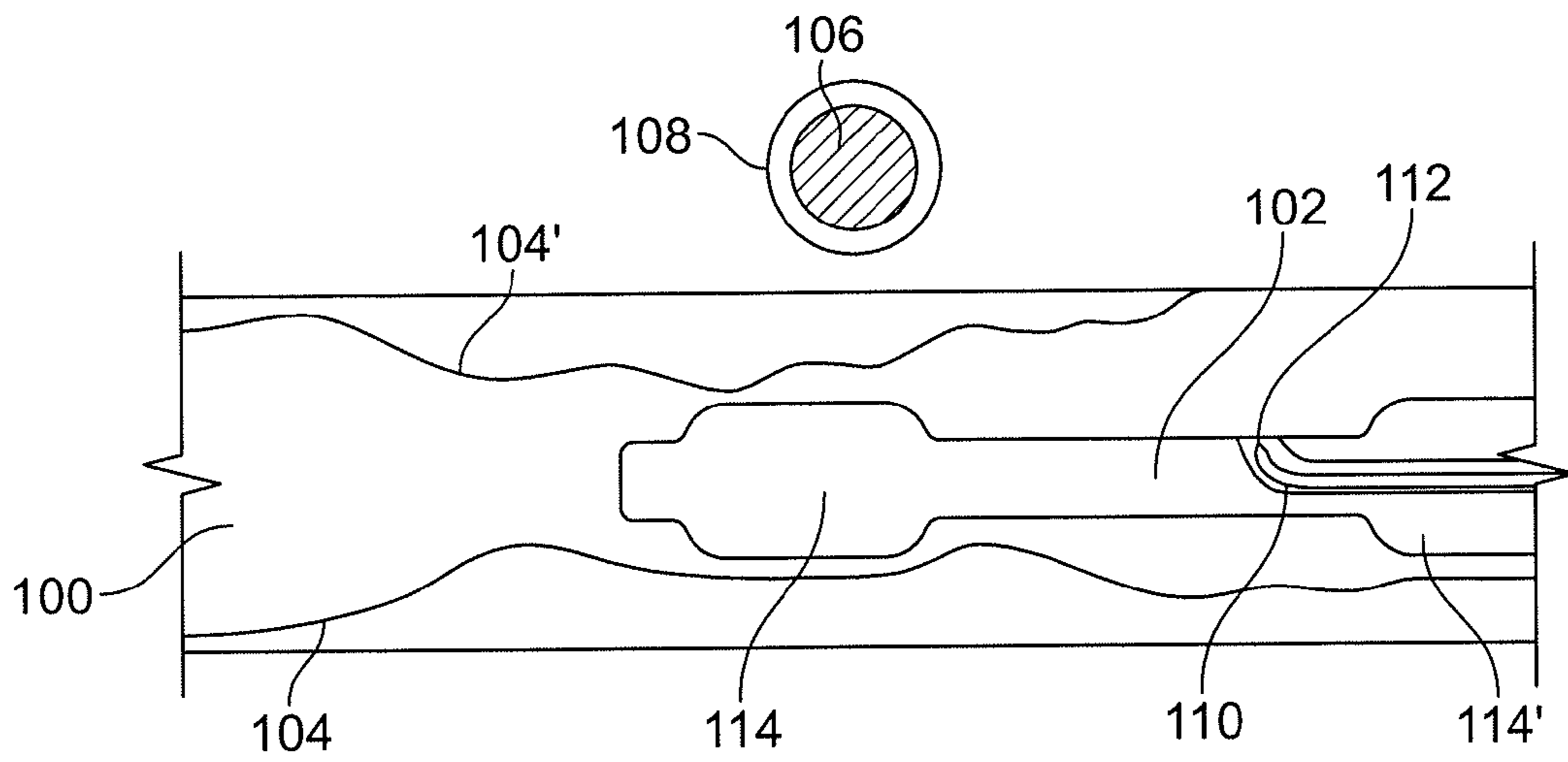
FIG. 1A
