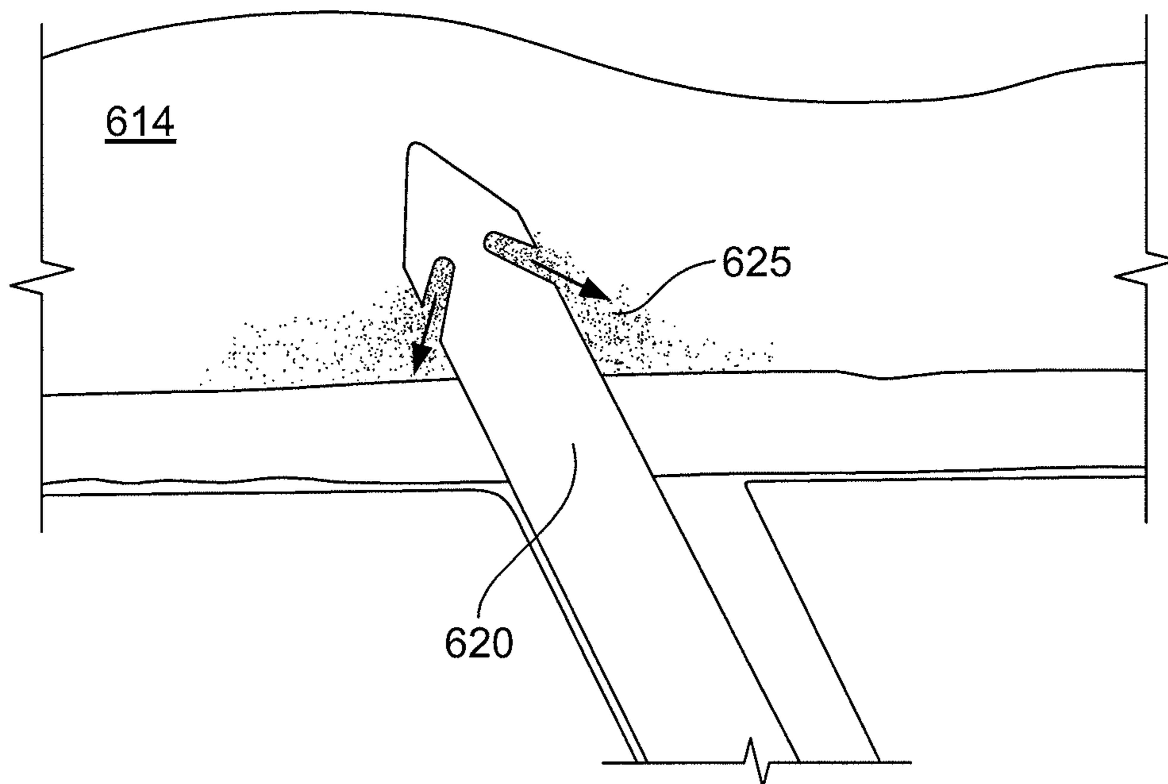
FIG. 6B
