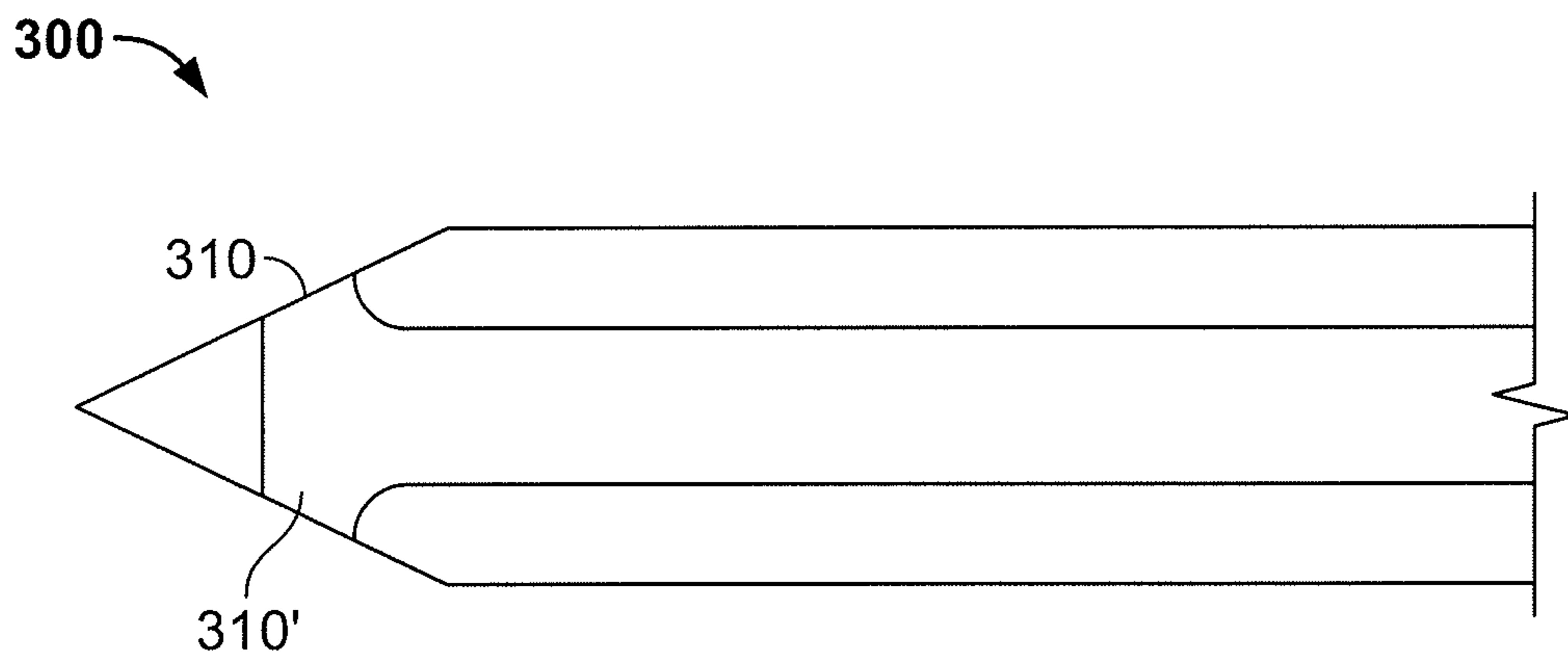
FIG. 3B
