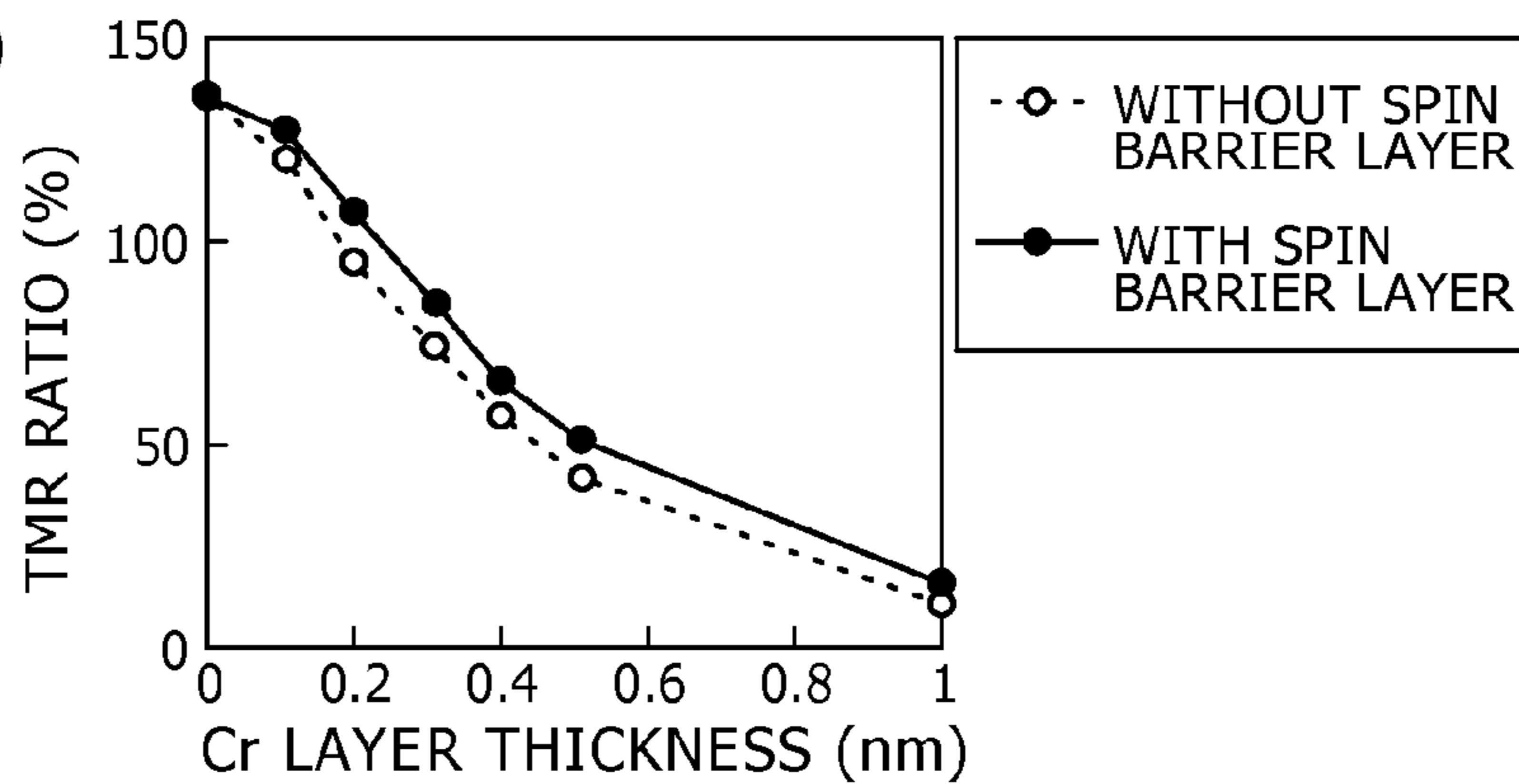
FIG. 9D
