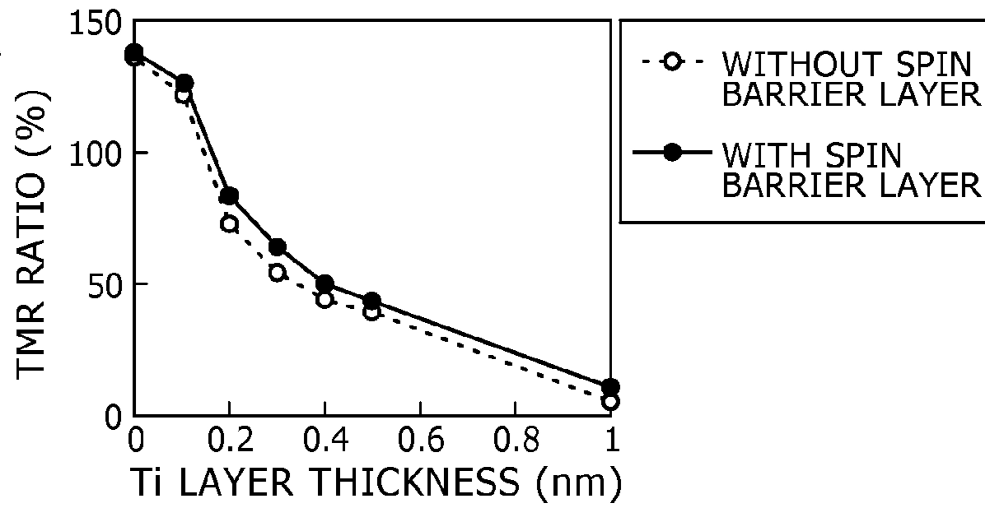
FIG. 9A
