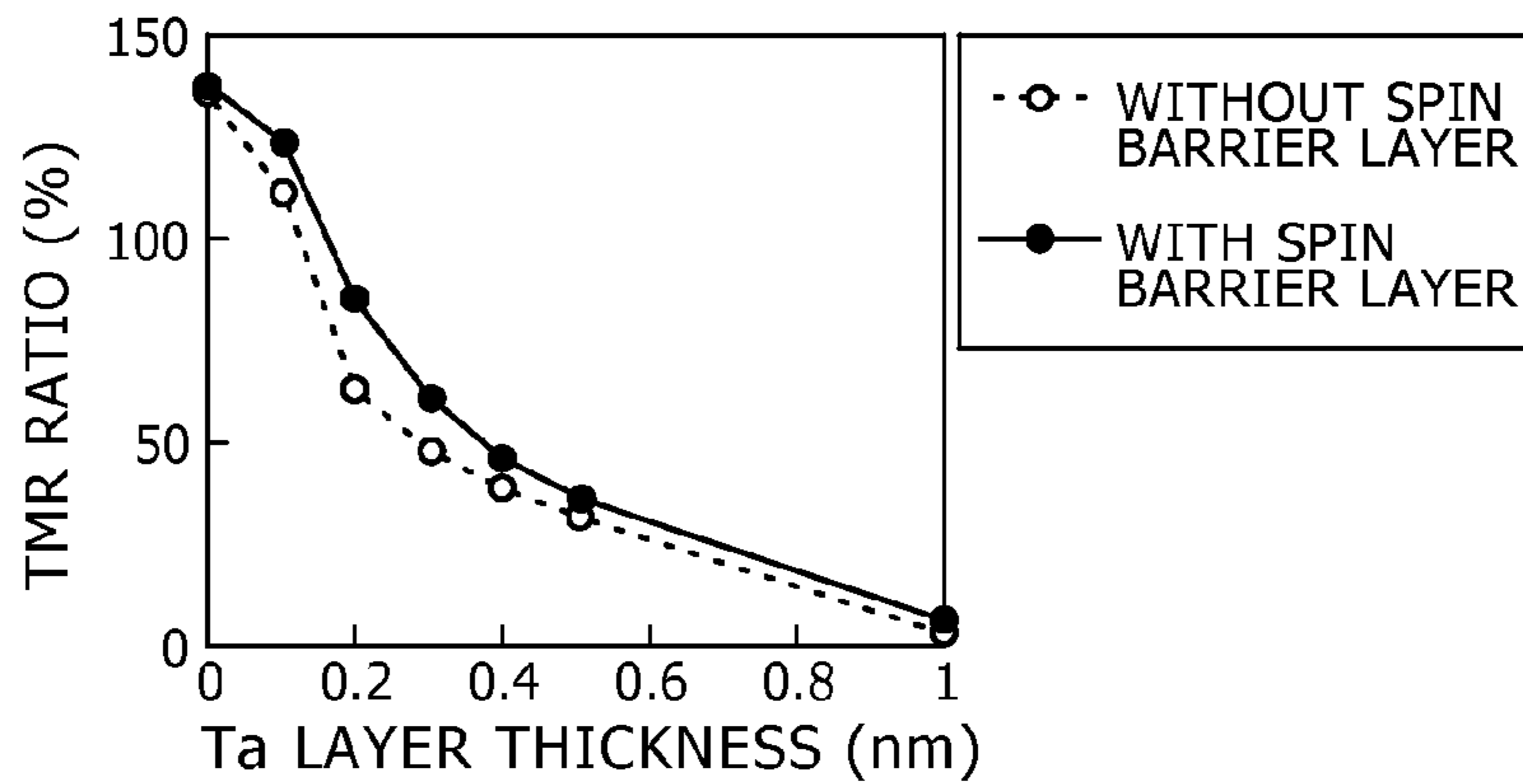
FIG. 9B
