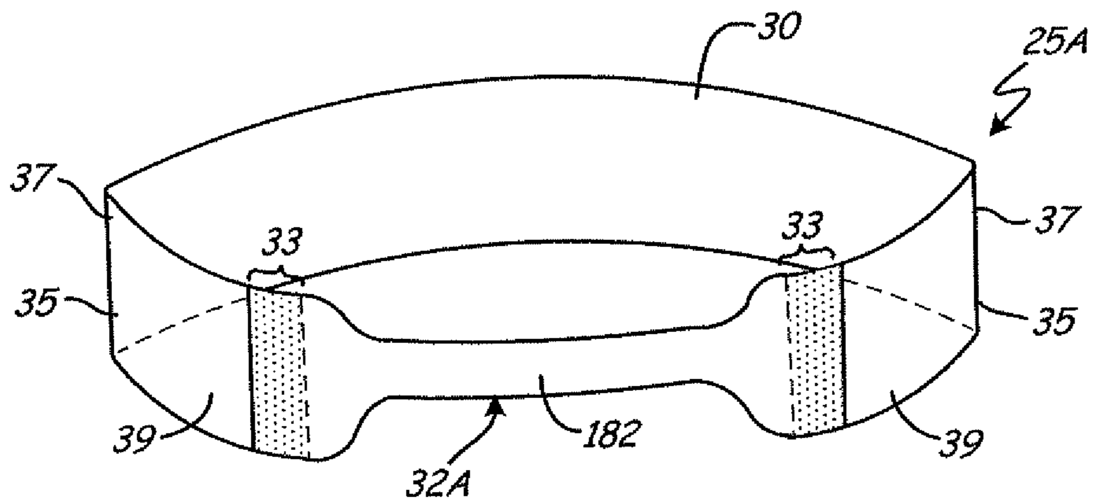
Fig. 19
