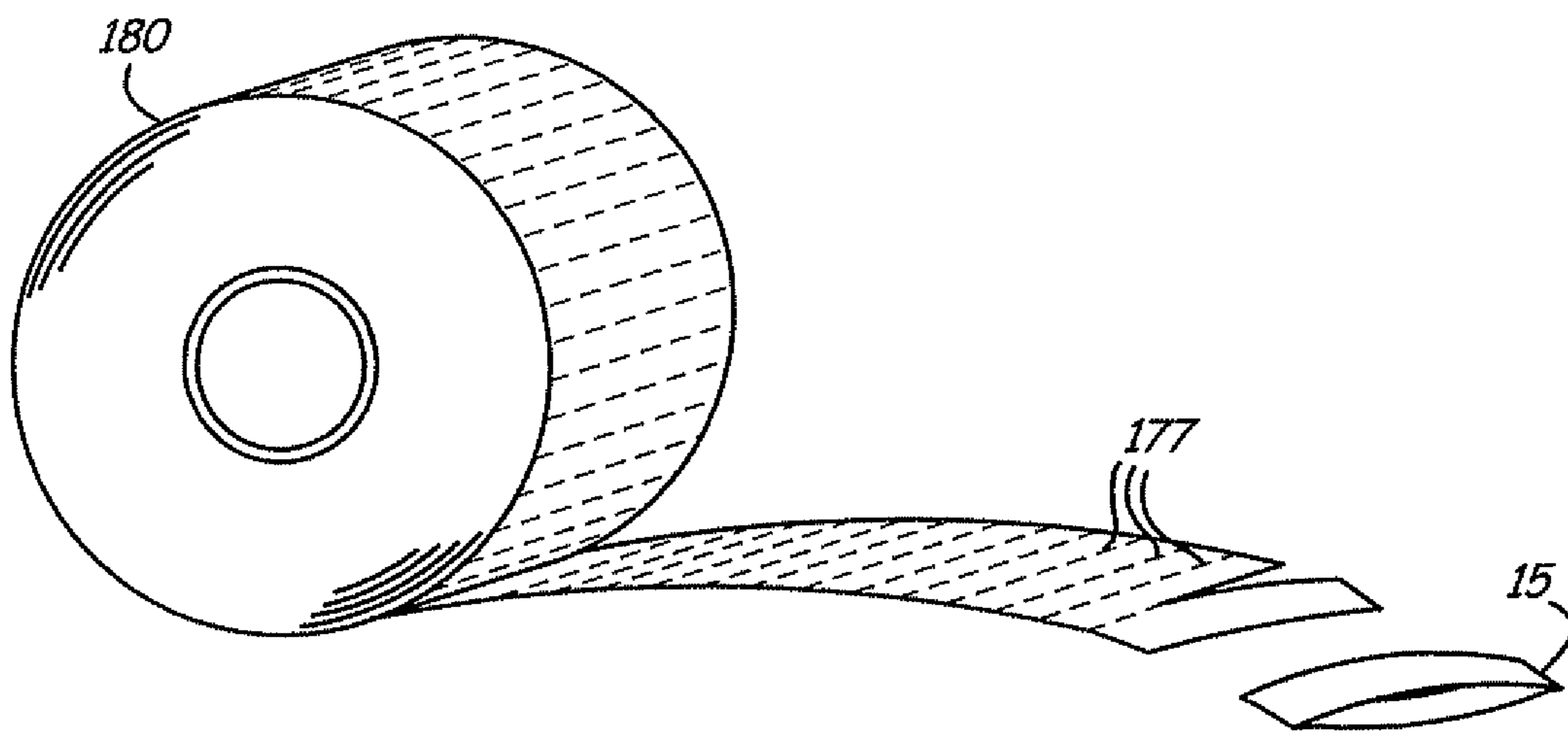
Fig. 18
