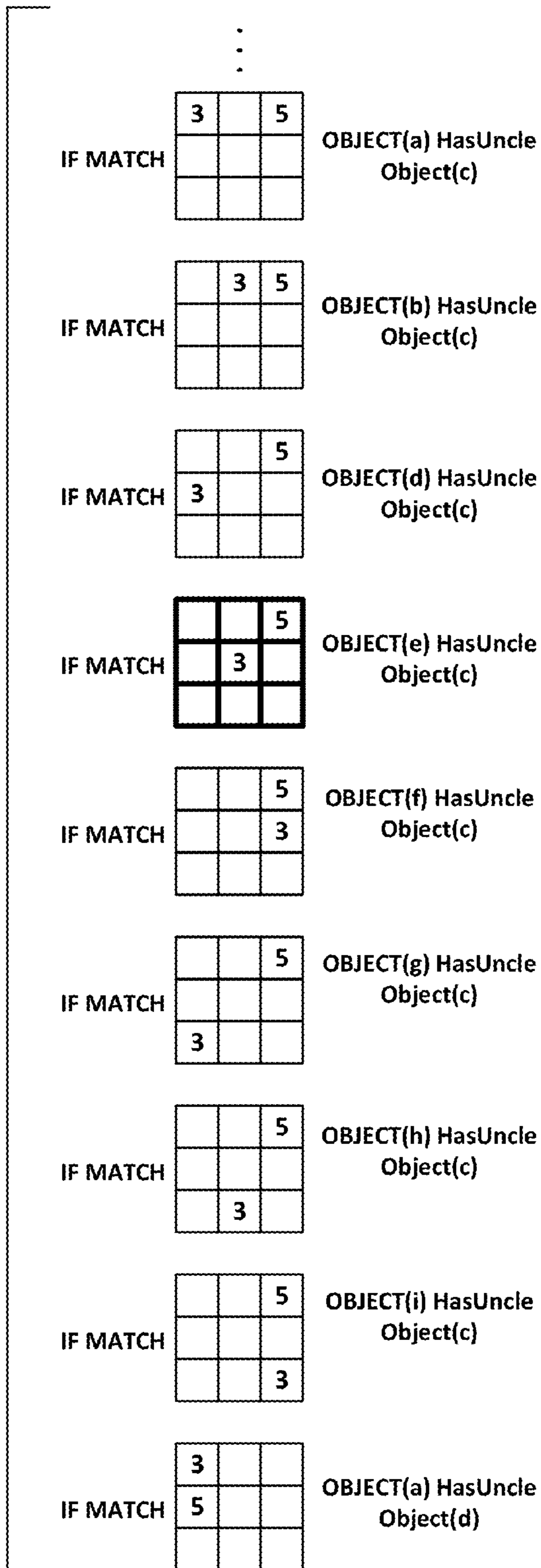
FIG. 26 – PREDICATE TEMPLATES
