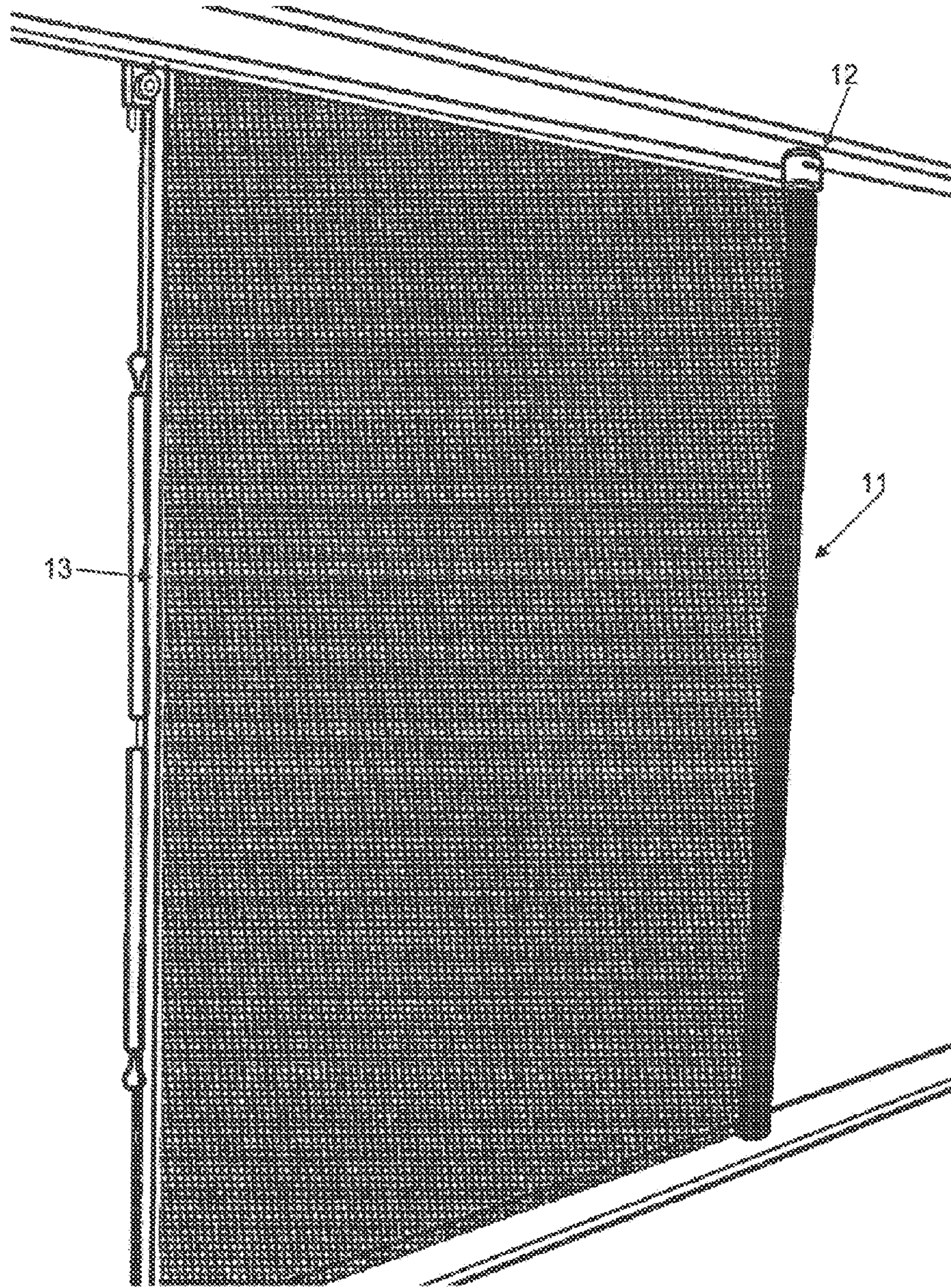
FIG. 6
