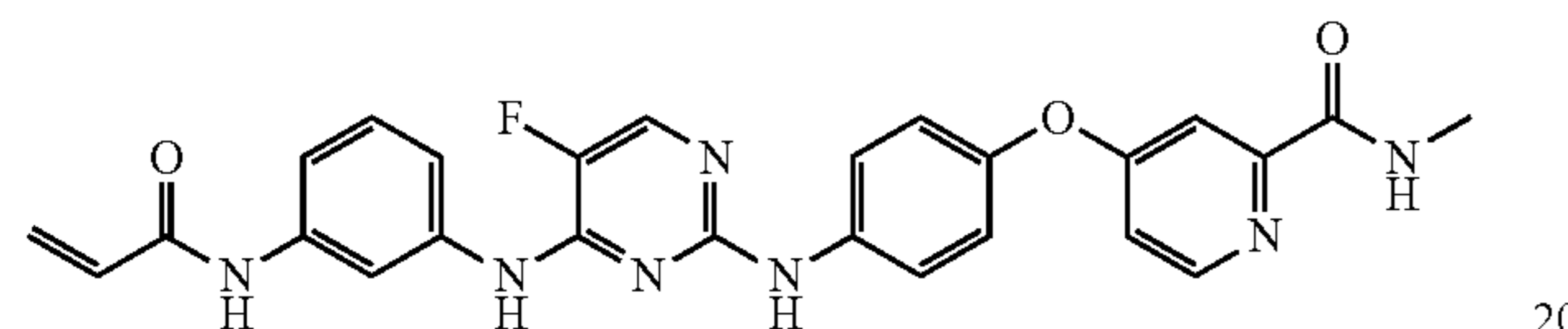
CNX-774
