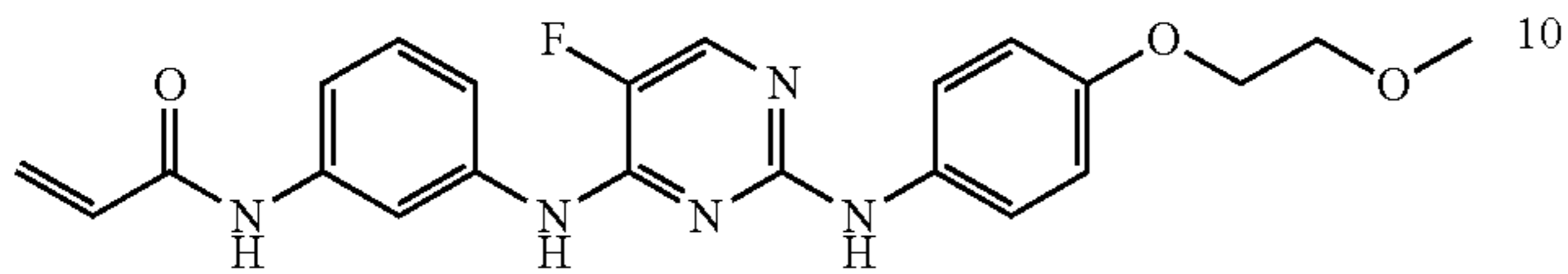
CC-292
