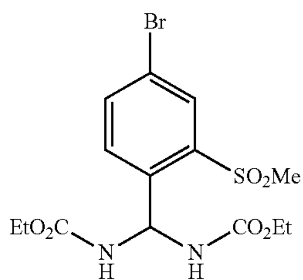
Diethyl (4-Bromo-2-methylsulfonyl)phenyl)methylenedicarbamate
