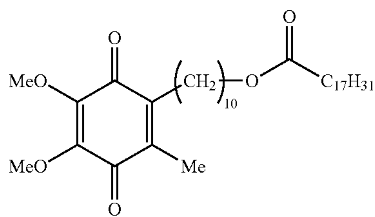
(idebenone linoleate ester)
