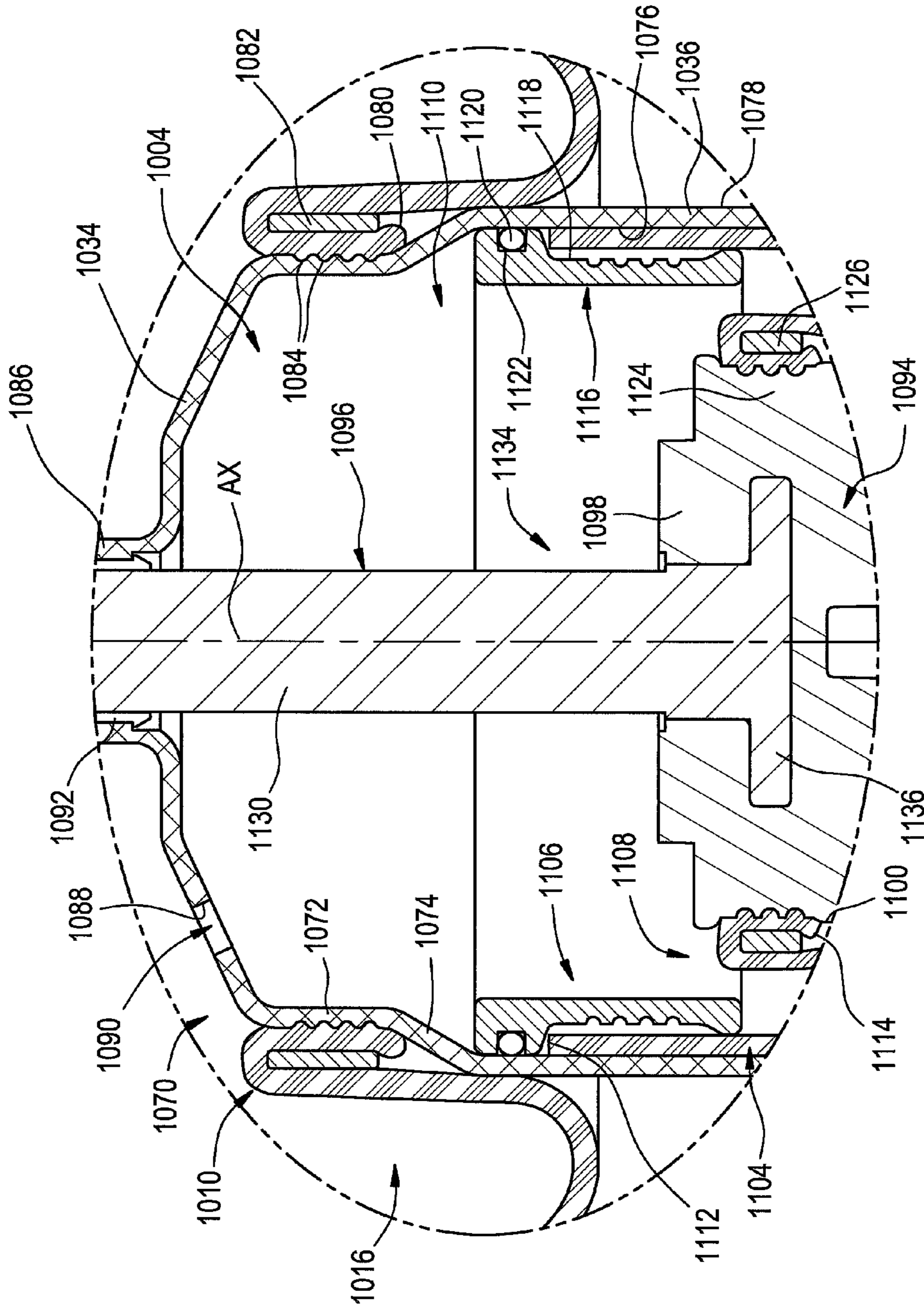
FIG. 19
