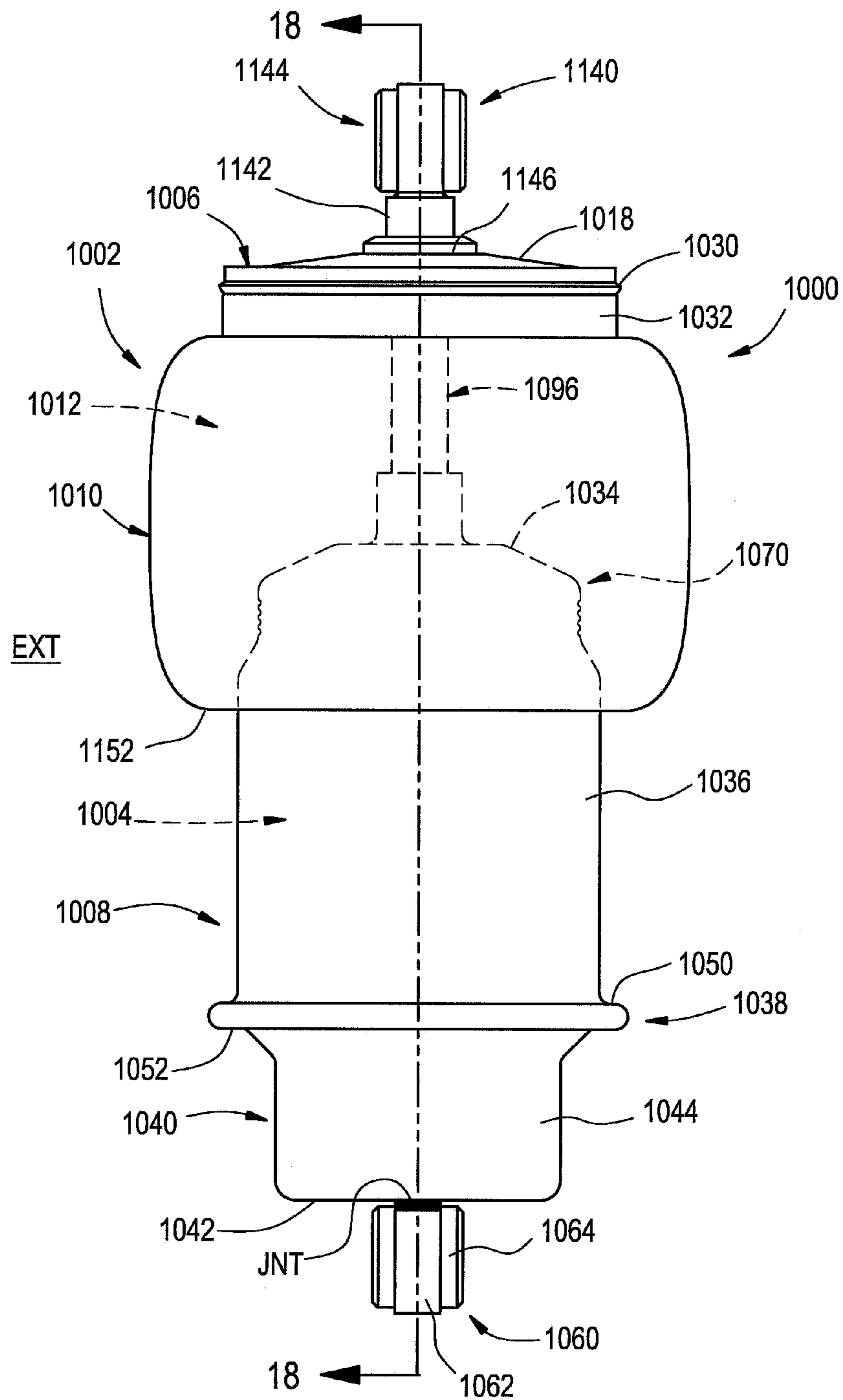
FIG. 17
