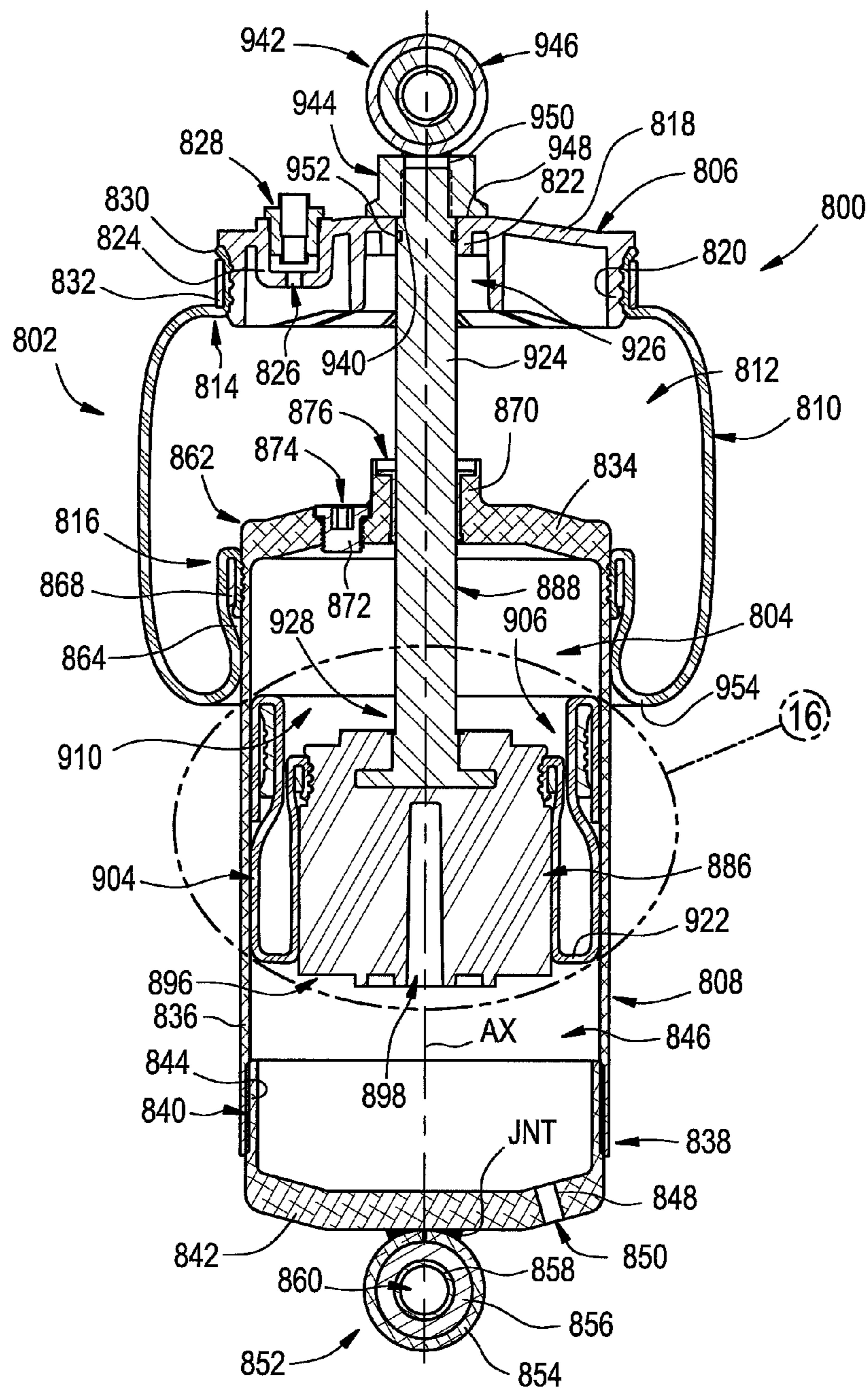
FIG. 15
