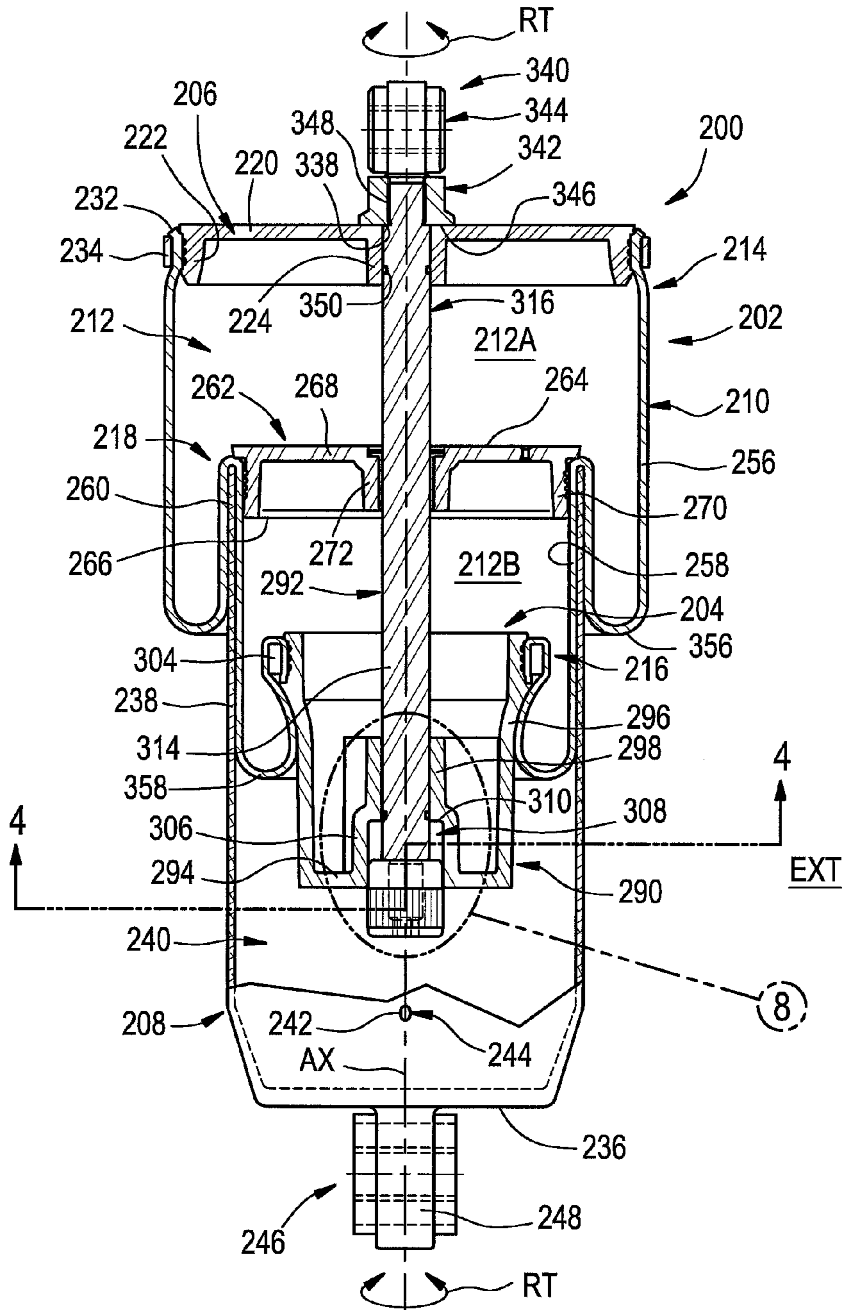
FIG. 3
