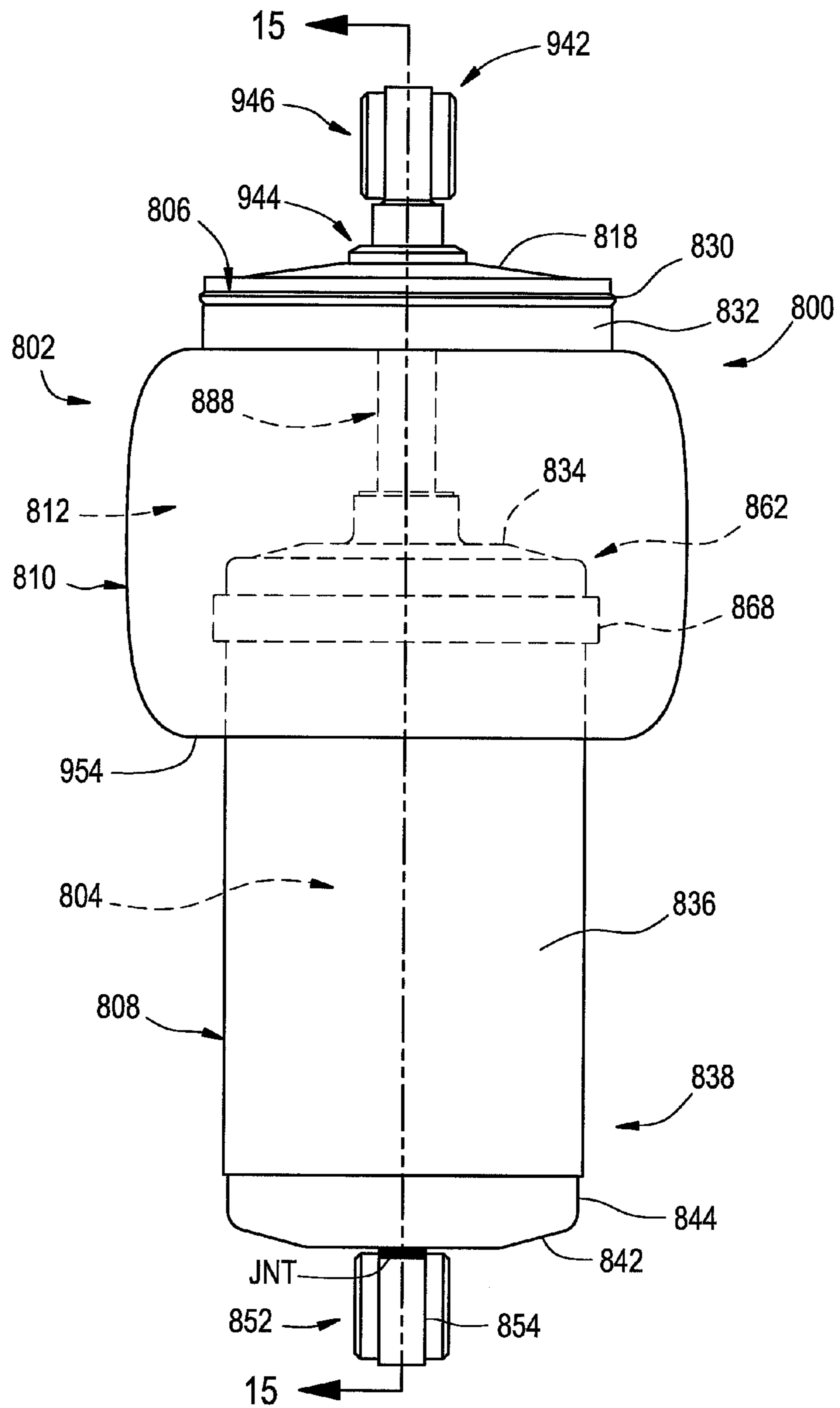
FIG. 14
