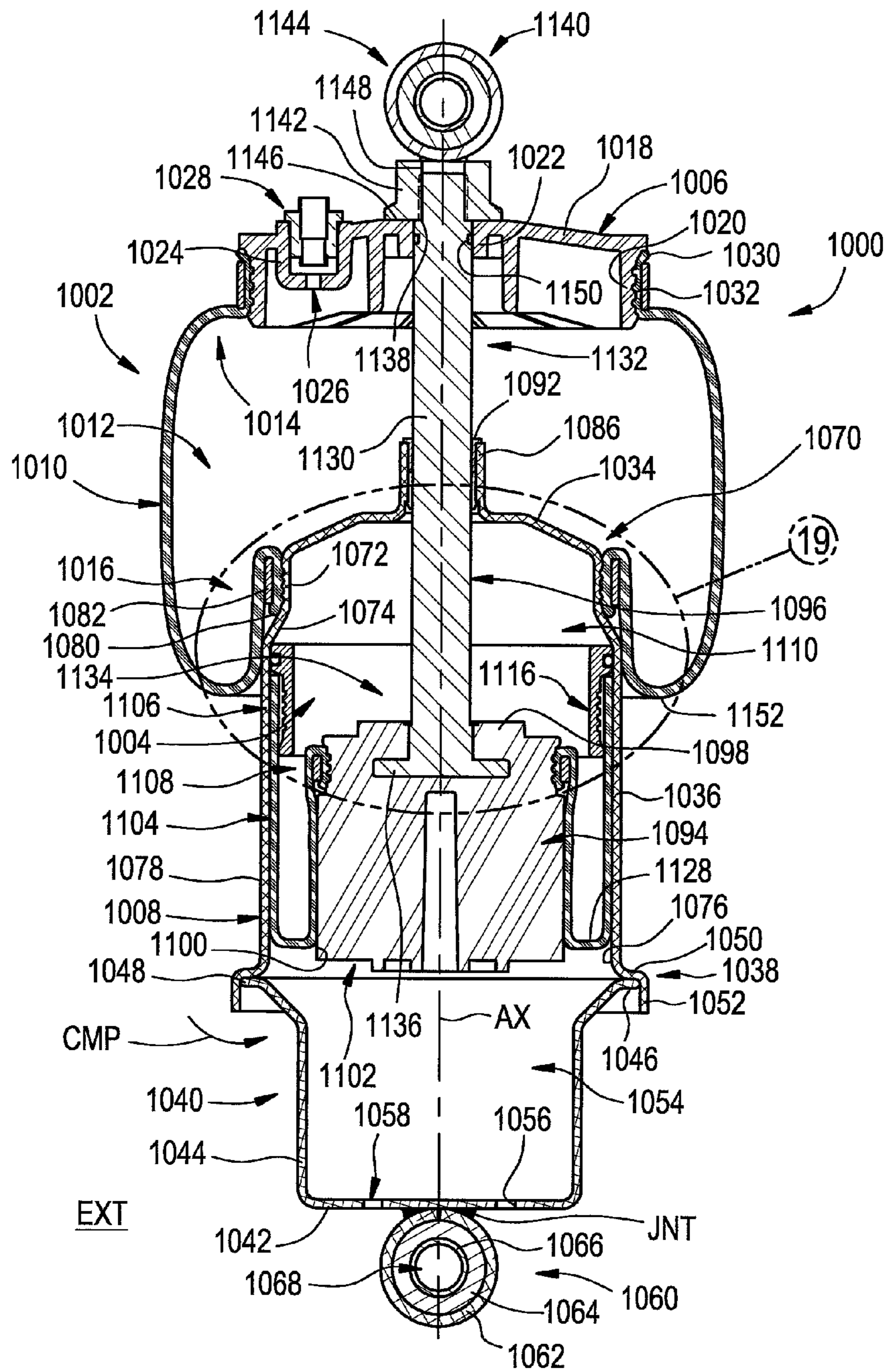
FIG. 18
