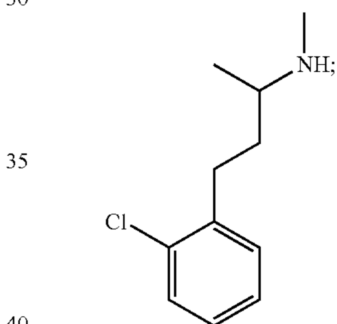
4-(2-fluorophenyl)butan-2-amine
