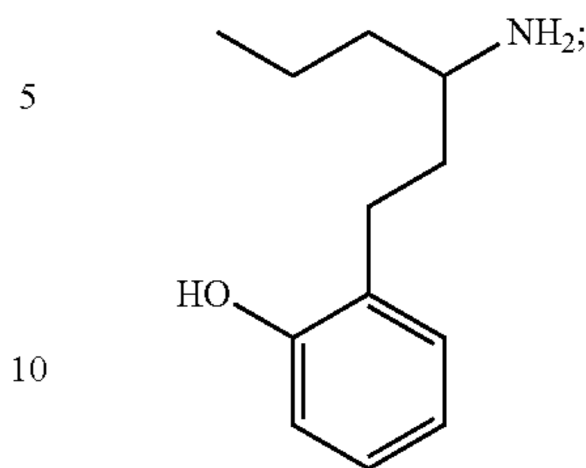
4-(2-chlorophenyl)-butan-2-amine
