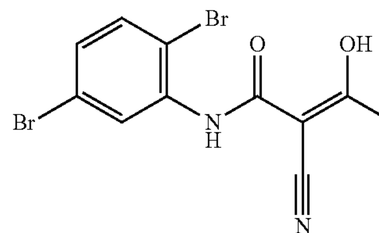
LFM-A13
