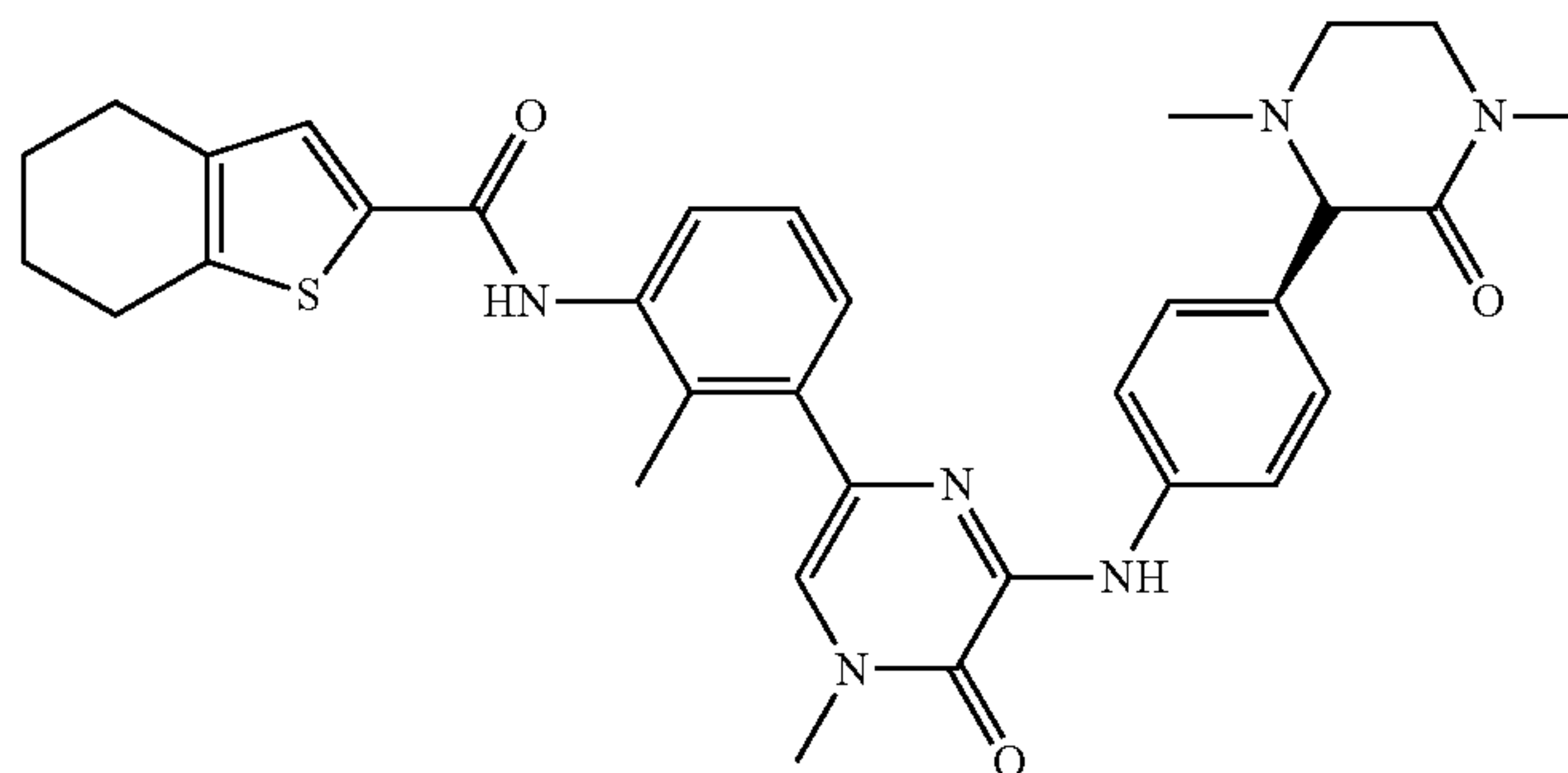
GDC-0834
