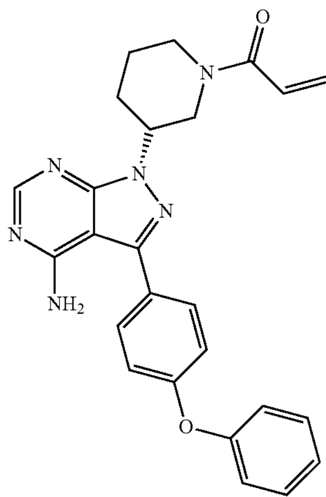
Ibrutinib
