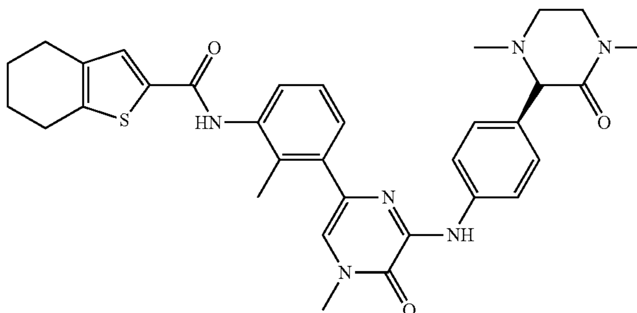
GDC-0834
