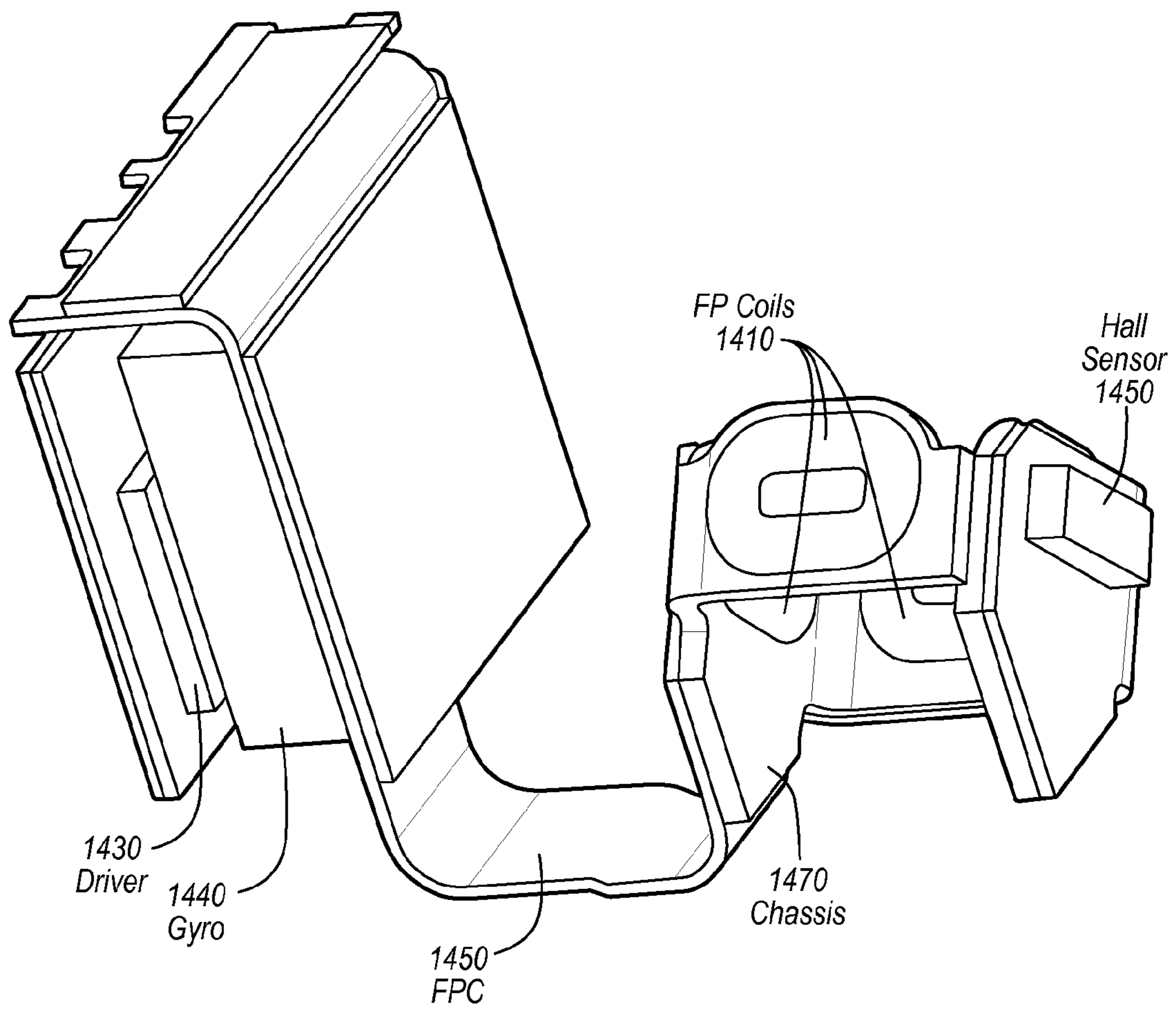
FIG. 14
