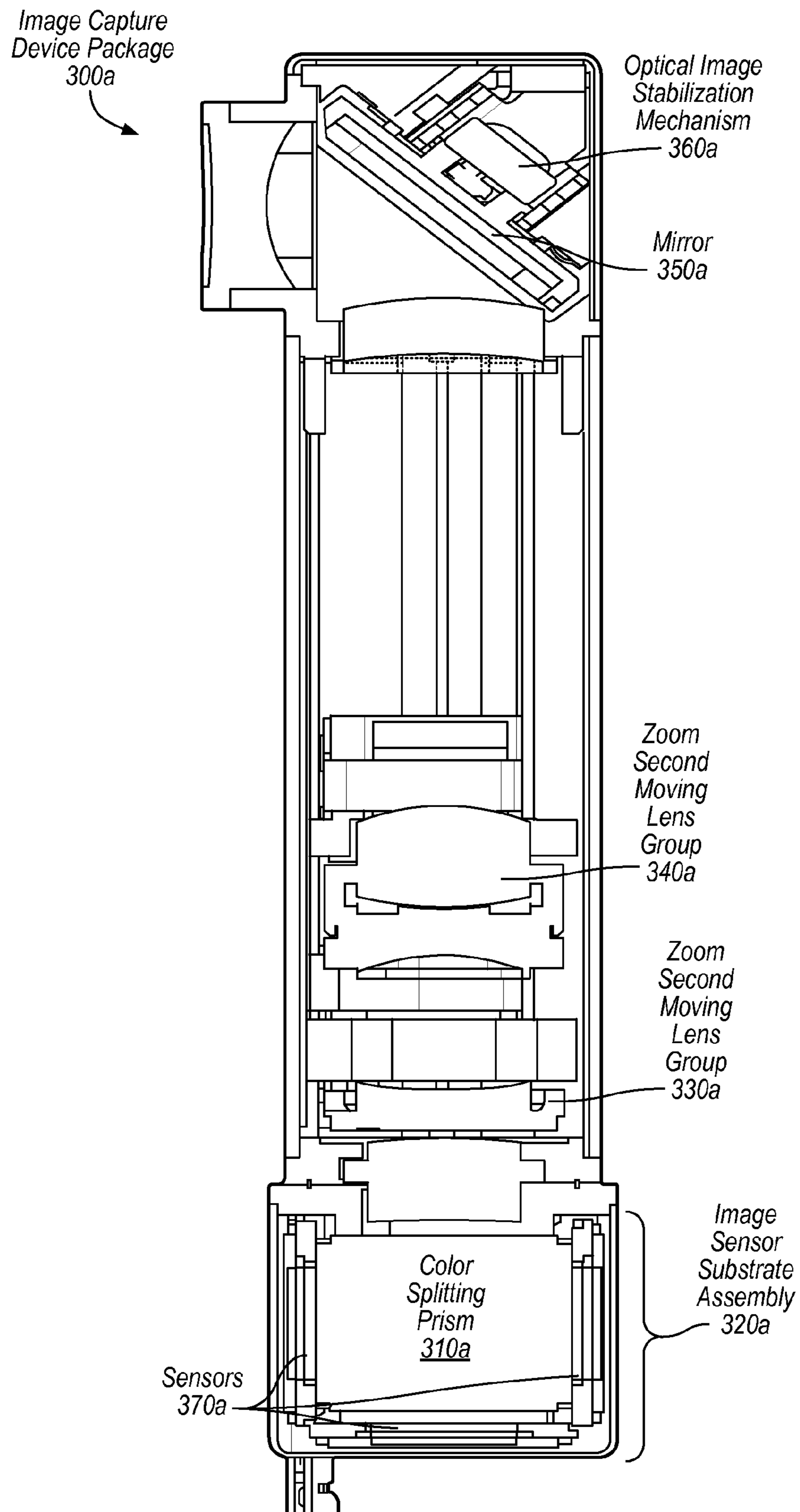
FIG. 3A
