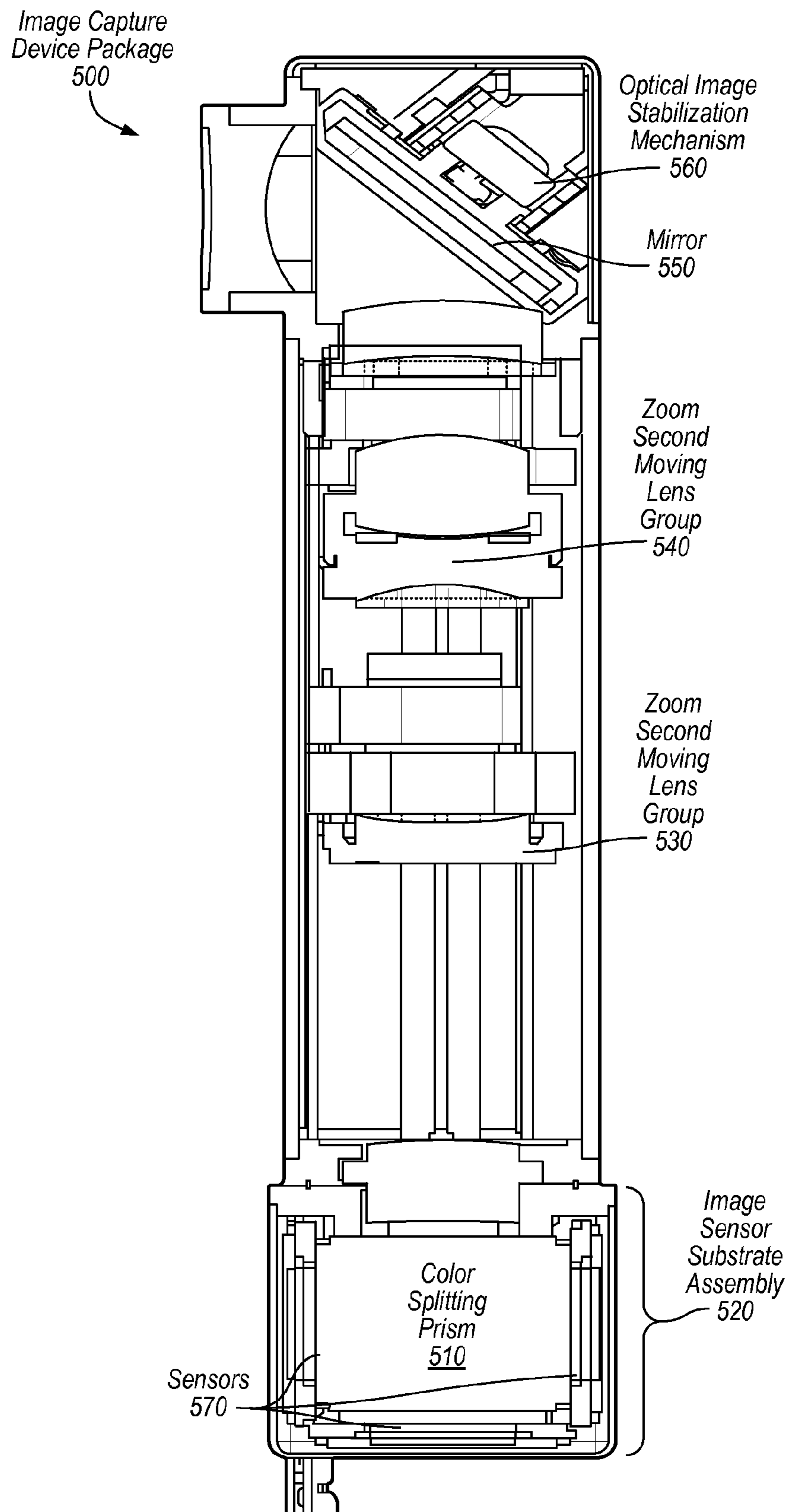
FIG. 5
