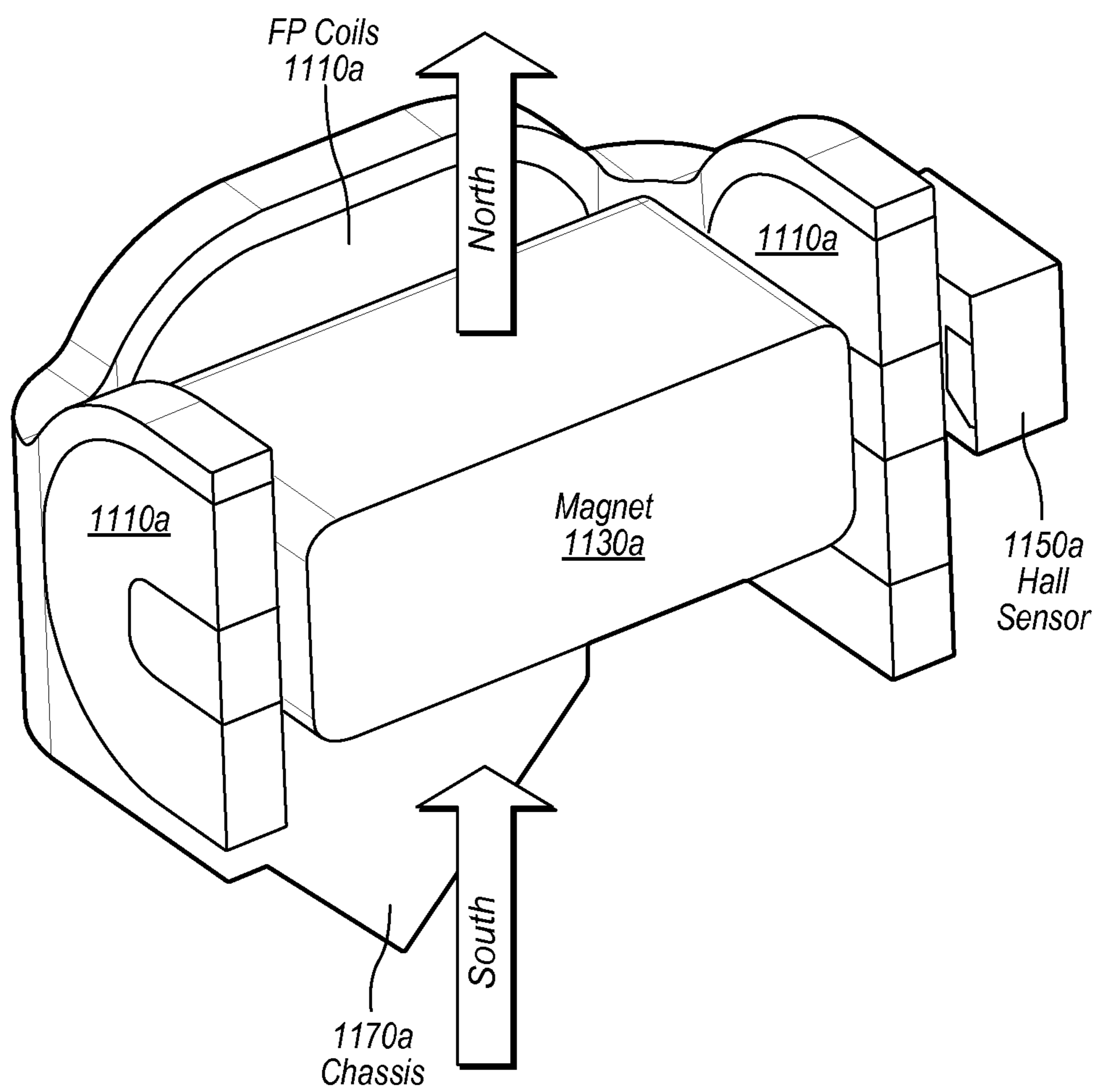
FIG. 11A
