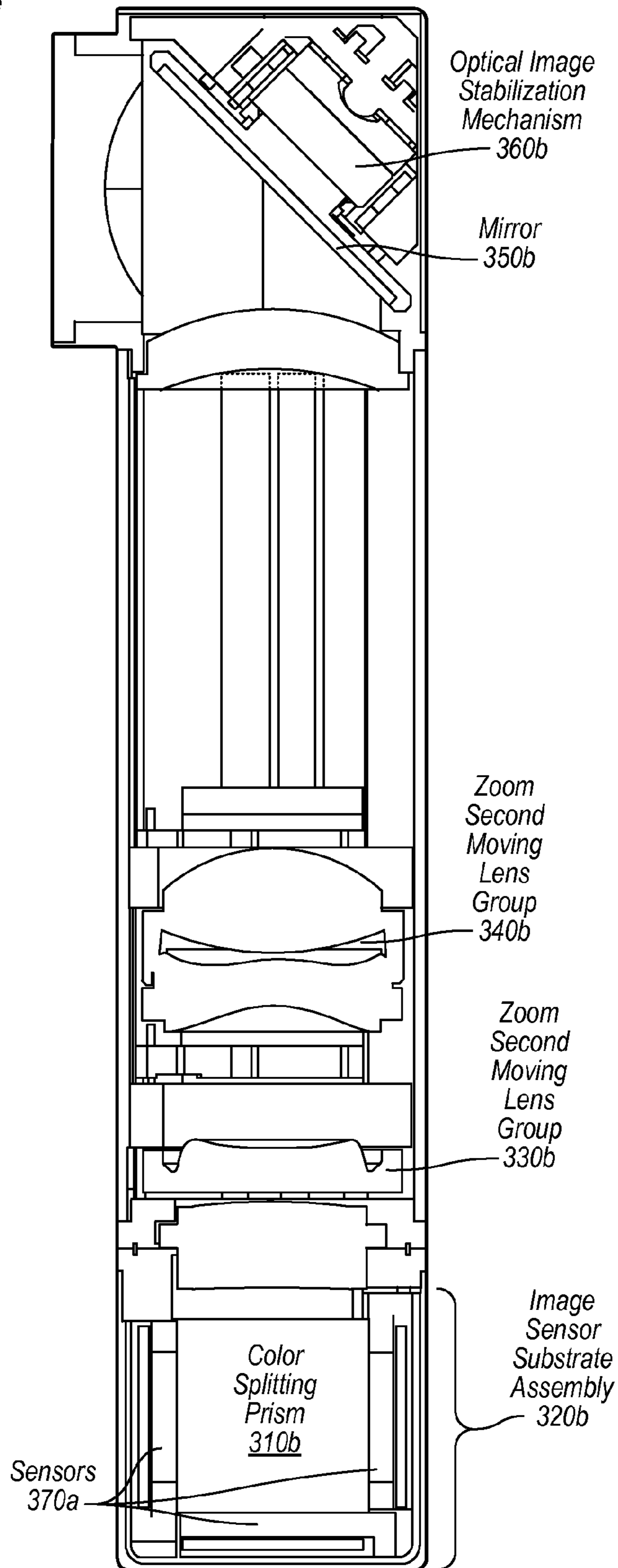
FIG. 3B
