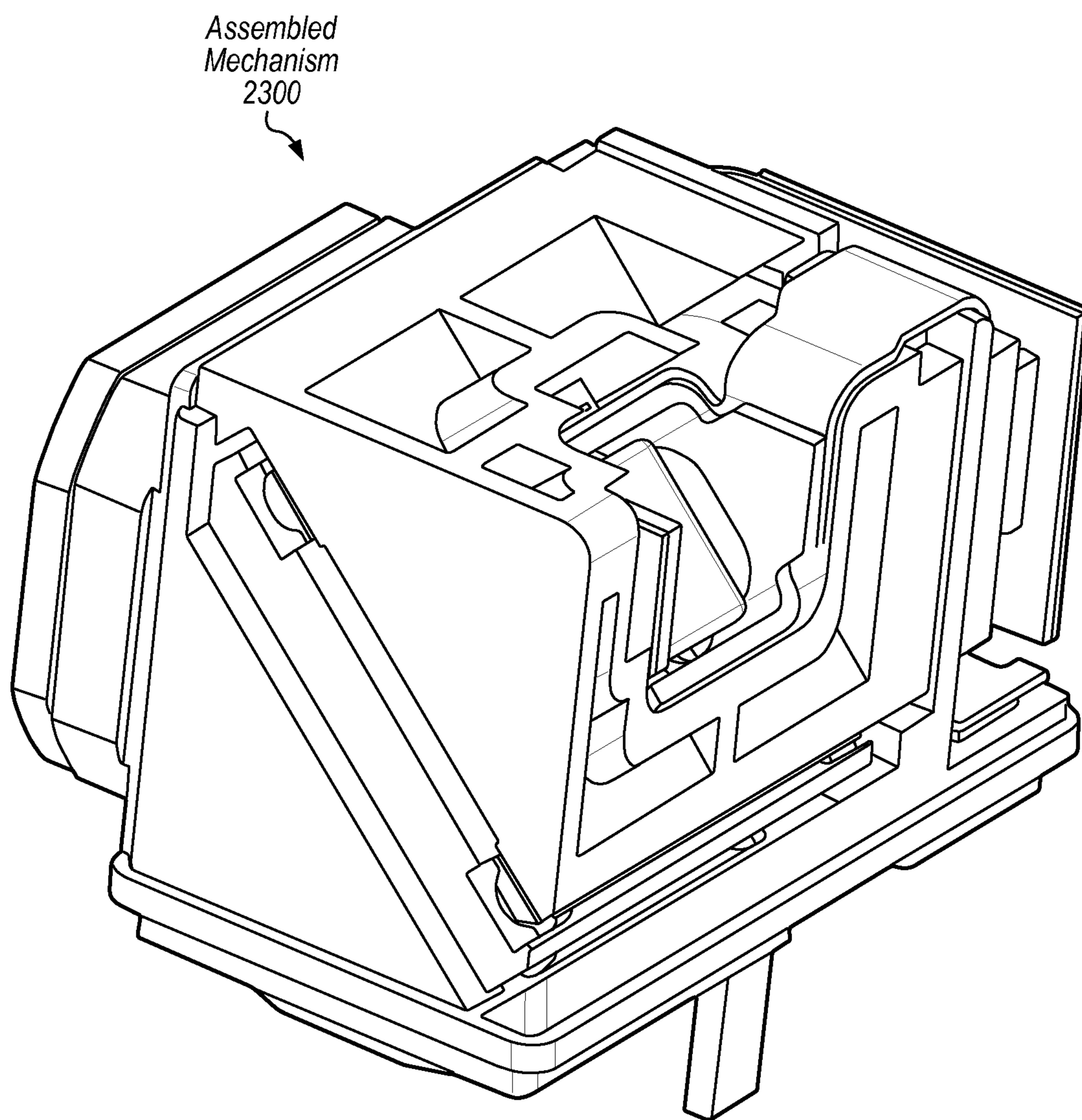
FIG. 23
