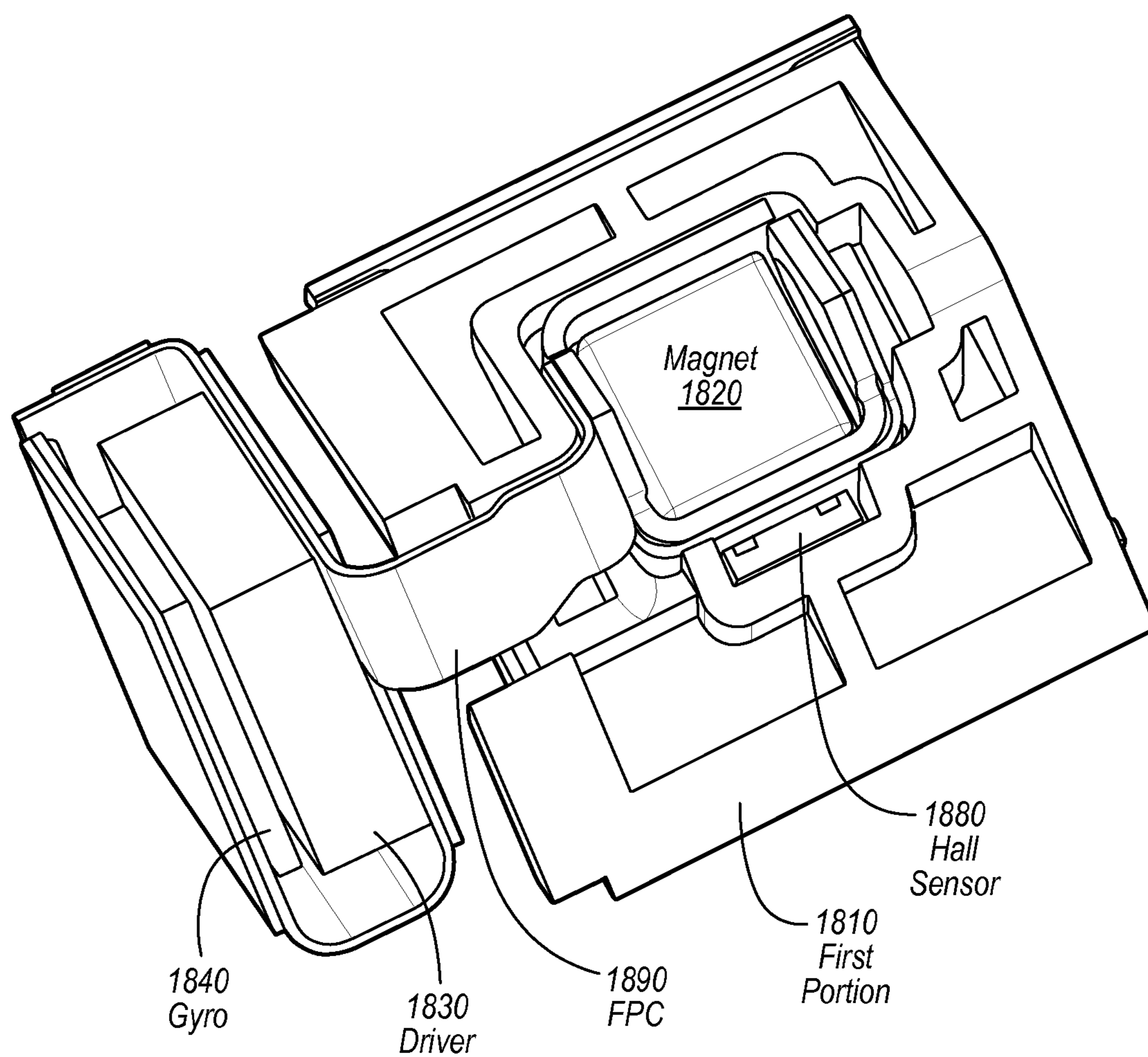
FIG. 18
