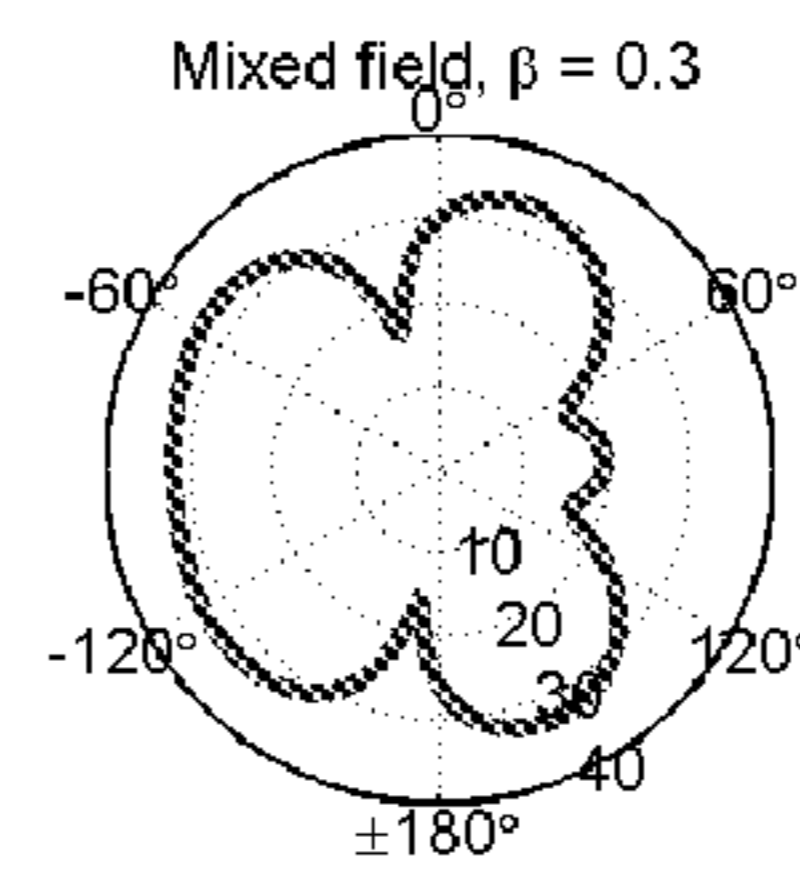
FIG. 8E
